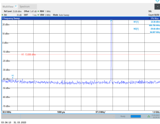
Band12-1.4MHz-QPSK-23017-1RB#0- Range1:30~1000MHz
