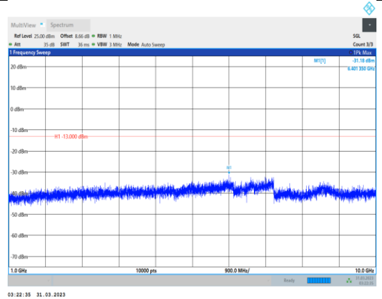
Band12-10MHz-QPSK-23130-1RB#0- Range2:1000~10000MHz
