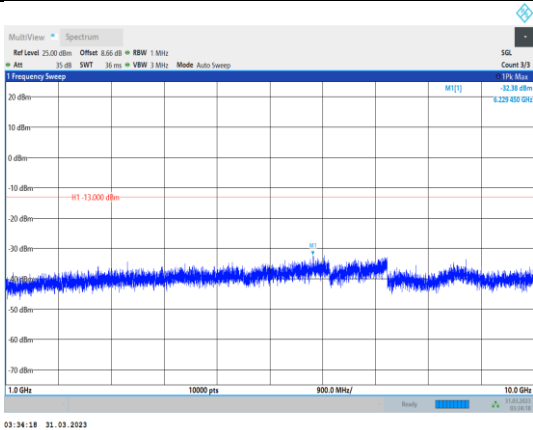
Band12-1.4MHz-QPSK-23017-1RB#0- Range2:1000~10000MHz
