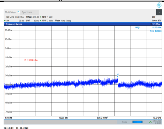
Band12-5MHz-QPSK-23155-1RB#0- Range2:1000~10000MHz
