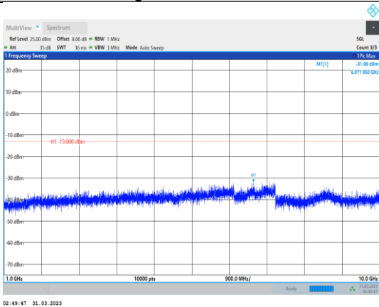
Band26-1.4MHz-QPSK-26697-1RB#0- Range2:1000~10000MHz
