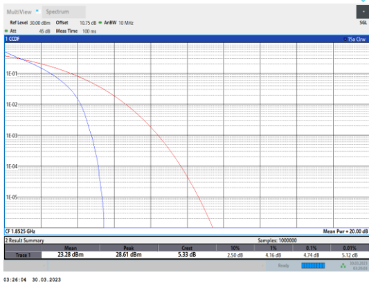
Band2-5MHz-QPSK-18625-25RB#0
