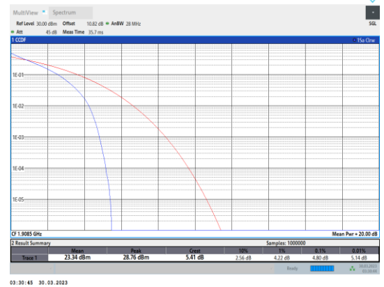
Band2-3MHz-QPSK-19185-15RB#0
