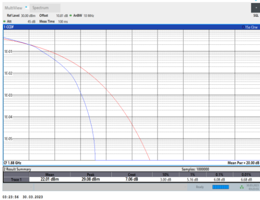
Band2-10MHz-16QAM-18900-50RB#0
