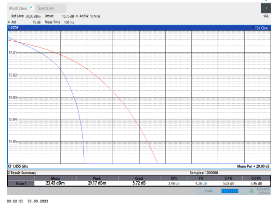
Band2-10MHz-QPSK-18650-50RB#0
