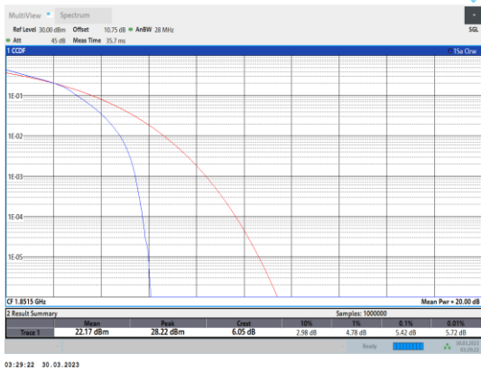
Band2-3MHz-16QAM-18615-15RB#0
