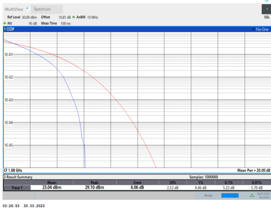
Band2-5MHz-QPSK-18900-25RB#0
