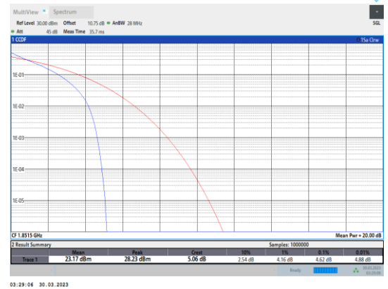
Band2-3MHz-QPSK-18615-15RB#0
