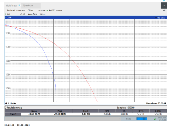
Band2-10MHz-QPSK-18900-50RB#0
