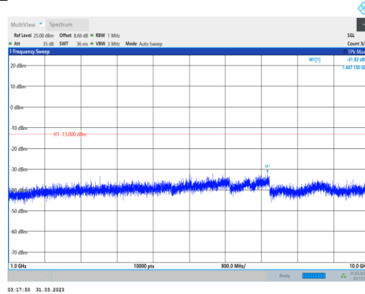
Band26-3MHz-QPSK-26775-1RB#0- Range2:1000~10000MHz
