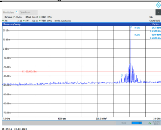
Band38-5MHz-QPSK-38225-1RB#0- Range2:1000~3000MHz
