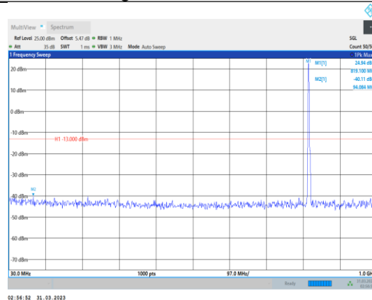
Band26-5MHz-QPSK-26765-1RB#0- Range1:30~1000MHz
