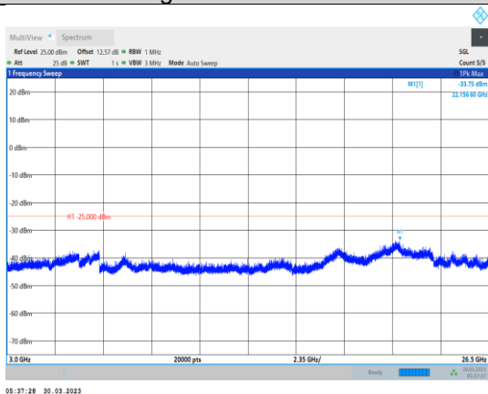
Band38-5MHz-QPSK-38225-1RB#0- Range3:3000~26500MHz
