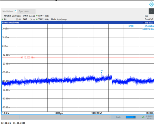
Band26-5MHz-QPSK-26715-1RB#0- Range2:1000~10000MHz
