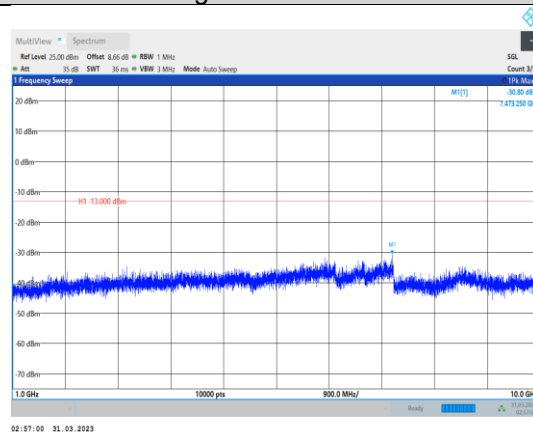
Band26-5MHz-QPSK-26765-1RB#0- Range2:1000~10000MHz
