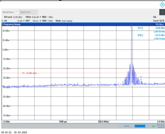
Band38-20MHz-QPSK-38000-1RB#0- Range2:1000~3000MHz
