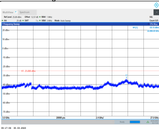
Band41-15MHz-QPSK-39725-1RB#0- Range3:3000~27000MHz
