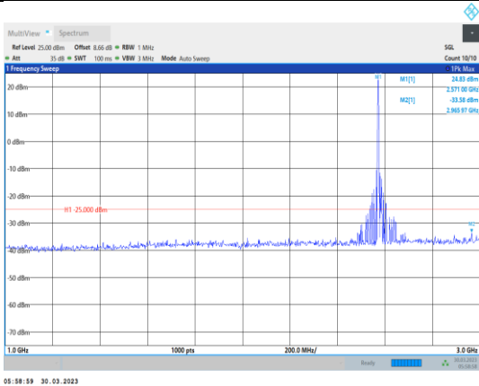
Band38-20MHz-16QAM-37850-1RB#0- Range2:1000~3000MHz
