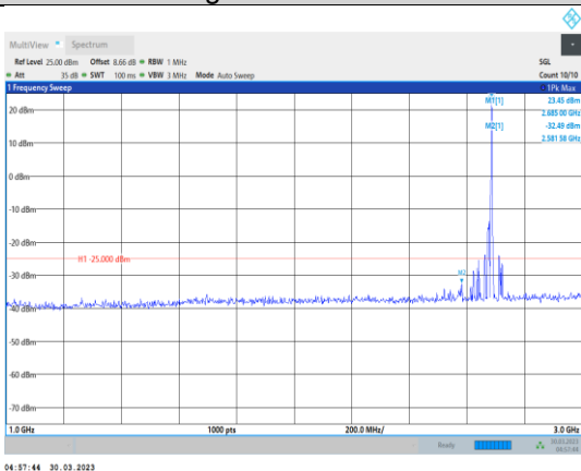
Band41-5MHz-QPSK-41565-1RB#0- Range2:1000~3000MHz
