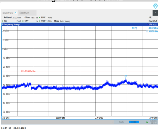
Band41-5MHz-QPSK-41565-1RB#0- Range3:3000~27000MHz
