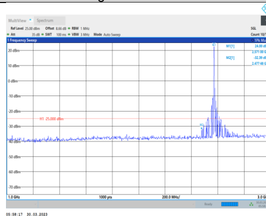
Band38-20MHz-QPSK-37850-1RB#0- Range2:1000~3000MHz
