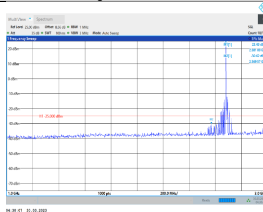
Band41-10MHz-QPSK-41540-1RB#0- Range2:1000~3000MHz
