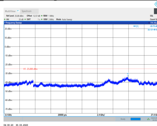
Band41-10MHz-QPSK-41540-1RB#0- Range3:3000~27000MHz
