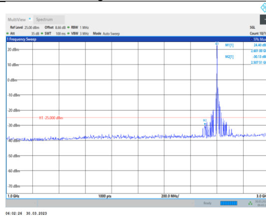
Band38-20MHz-QPSK-38150-1RB#0- Range2:1000~3000MHz
