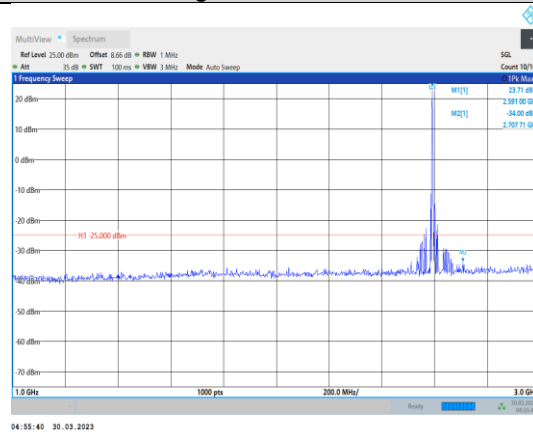
Band41-5MHz-QPSK-40620-1RB#0- Range2:1000~3000MHz
