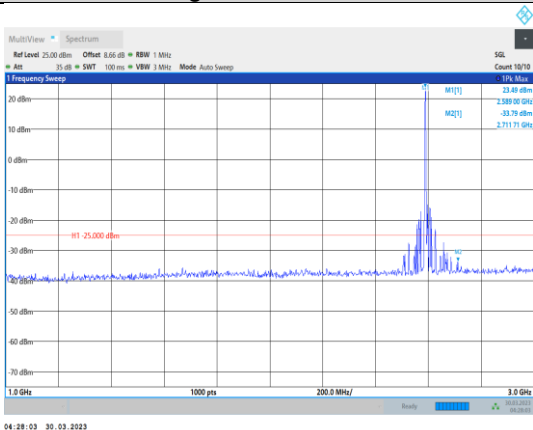
Band41-10MHz-QPSK-40620-1RB#0- Range2:1000~3000MHz
