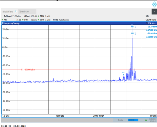
Band41-15MHz-QPSK-41515-1RB#0- Range2:1000~3000MHz
