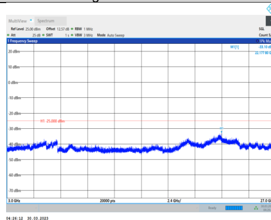
Band41-10MHz-QPSK-39700-1RB#0- Range3:3000~27000MHz
