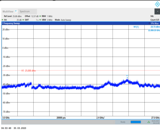
Band41-5MHz-QPSK-39675-1RB#0- Range3:3000~27000MHz
