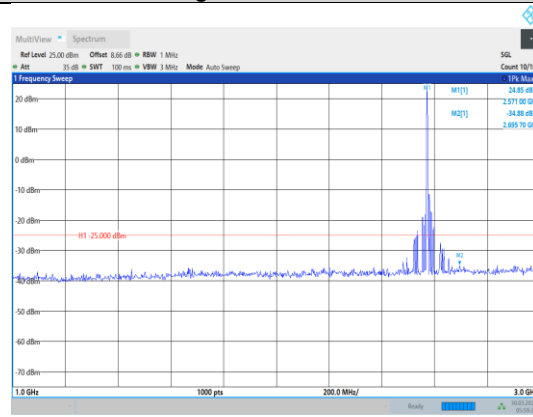
Band38-20MHz-64QAM-37850-1RB#0- Range2:1000~3000MHz
