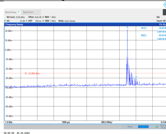
Band41-10MHz-QPSK-39700-1RB#0- Range2:1000~3000MHz
