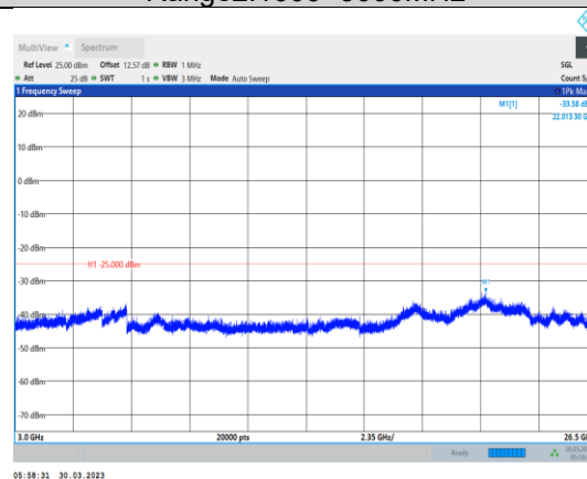
Band38-20MHz-QPSK-37850-1RB#0- Range3:3000~26500MHz
