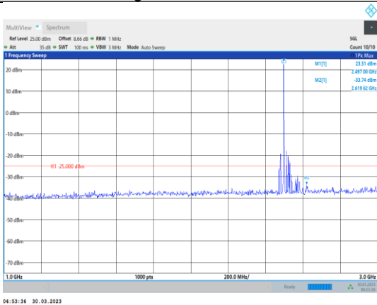
Band41-5MHz-QPSK-39675-1RB#0- Range2:1000~3000MHz
