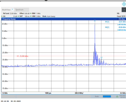
Band41-15MHz-QPSK-39725-1RB#0- Range2:1000~3000MHz
