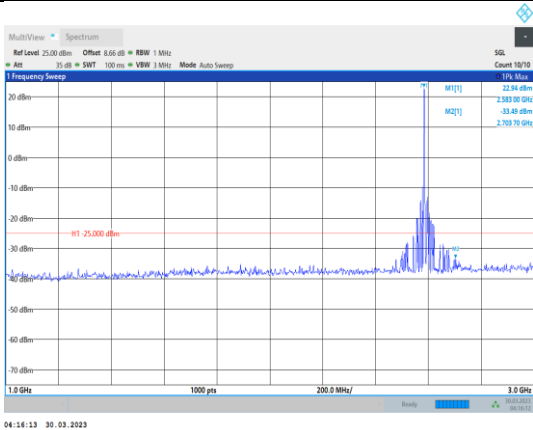
Band41-20MHz-QPSK-40620-1RB#0- Range2:1000~3000MHz
