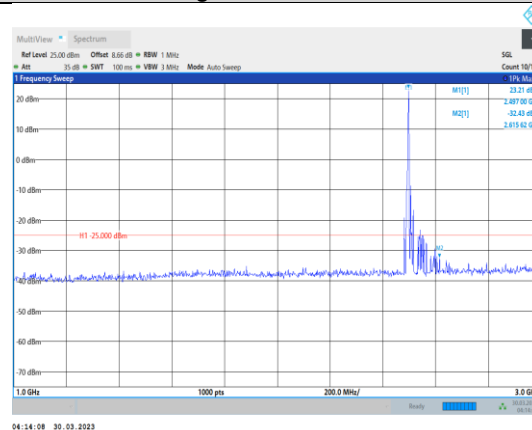
Band41-20MHz-QPSK-39750-1RB#0- Range2:1000~3000MHz
