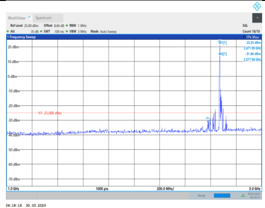
Band41-20MHz-QPSK-41490-1RB#0- Range2:1000~3000MHz
