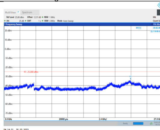
Band41-20MHz-QPSK-39750-1RB#0- Range3:3000~27000MHz
