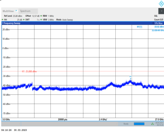
Band41-20MHz-QPSK-40620-1RB#0- Range3:3000~27000MHz
