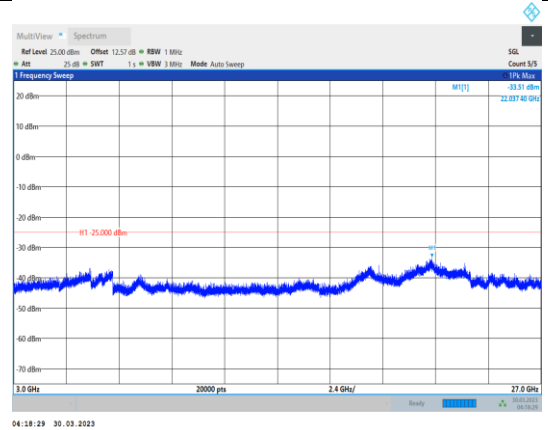
Band41-20MHz-QPSK-41490-1RB#0- Range3:3000~27000MHz
