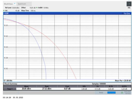
Band2-20MHz-QPSK-18900-100RB#0
