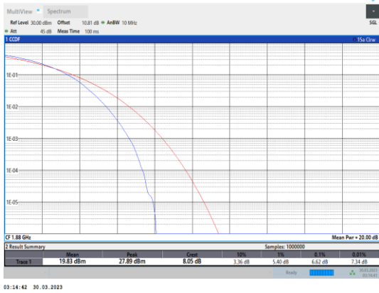
Band2-20MHz-16QAM-18900-100RB#0
