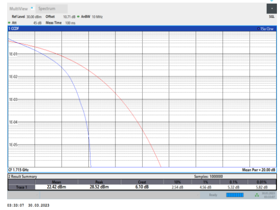
Band4-10MHz-QPSK-20000-50RB#0
