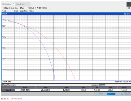
Band2-20MHz-16QAM-18700-100RB#0
