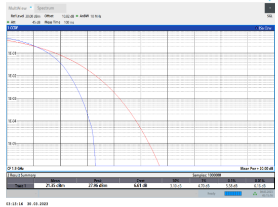
Band2-20MHz-QPSK-19100-100RB#0
