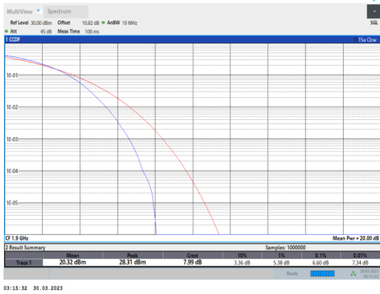
Band2-20MHz-16QAM-19100-100RB#0
