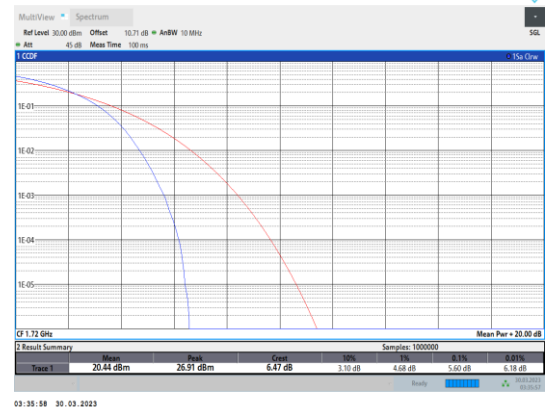
Band4-20MHz-QPSK-20050-100RB#0
