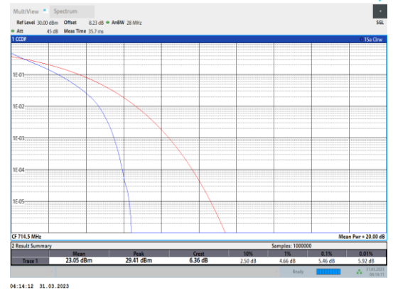
Band12-3MHz-QPSK-23165-15RB#0
