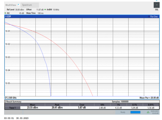
Band7-10MHz-QPSK-20800-50RB#0
