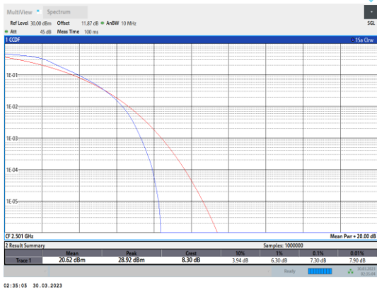
Band41-10MHz-QPSK-39700-50RB#0
