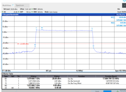
Band2-20MHz-16QAM-18900-100RB#0
