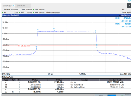
Band2-20MHz-16QAM-19100-100RB#0
