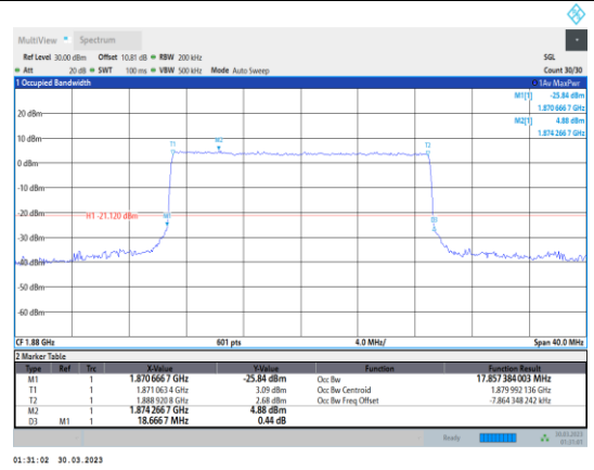
Band2-20MHz-QPSK-18900-100RB#0
