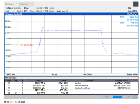
Band5-3MHz-QPSK-20635-15RB#0
