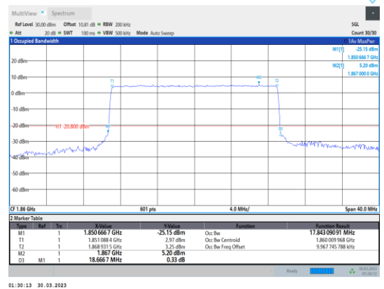
Band2-20MHz-QPSK-18700-100RB#0
