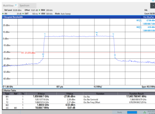
Band2-20MHz-16QAM-18700-100RB#0
