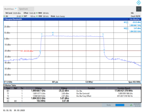
Band2-20MHz-QPSK-19100-100RB#0
