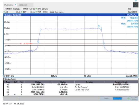
Band41-10MHz-QPSK-39700-50RB#0
