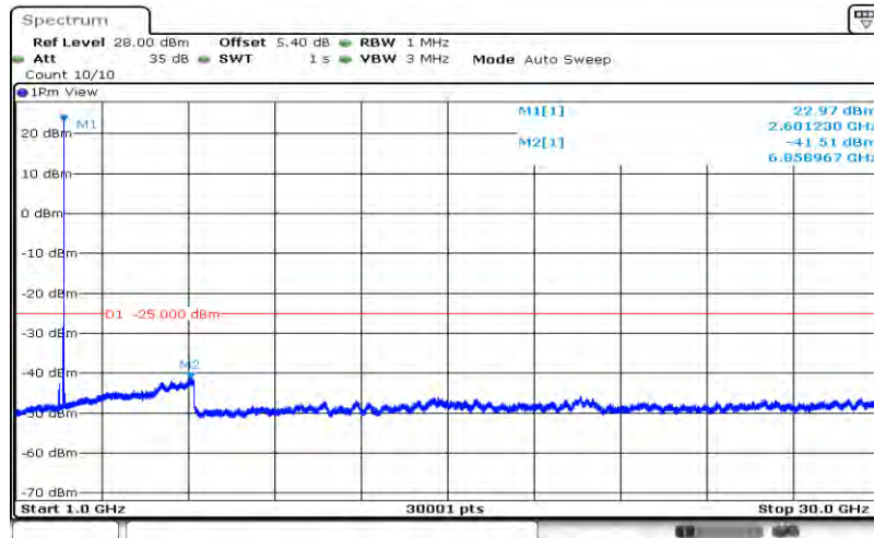
Band38-20MHz-QPSK-38150-1RB#0-Range2:1000~30000MHz
