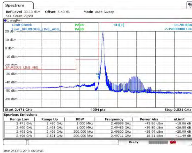
Band41_15MHz_QPSK_39725_75RB#0
