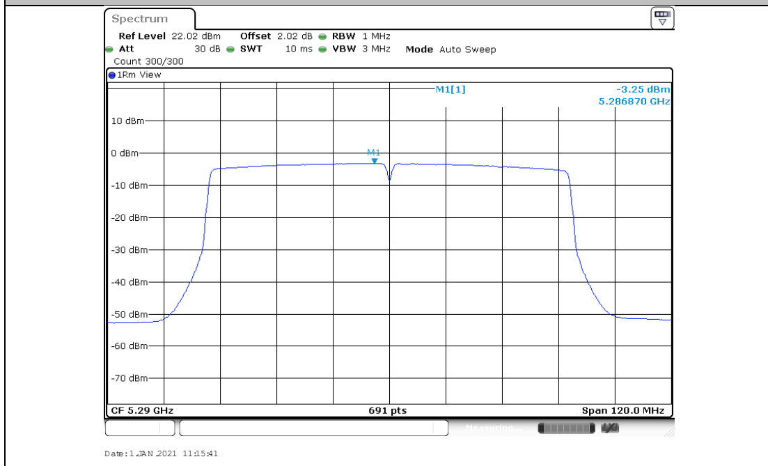
11AC80MIMO_Ant2_5290
