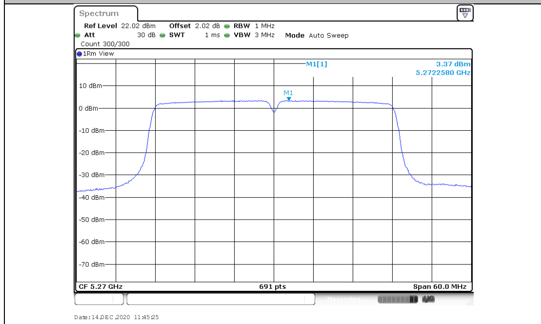
11AC40MIMO_Ant2_5270
