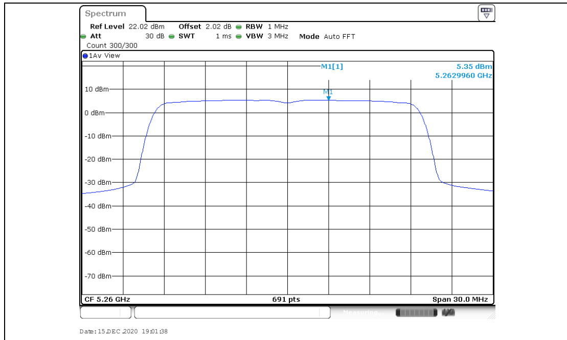
11AX20SISO_Ant2_5260
