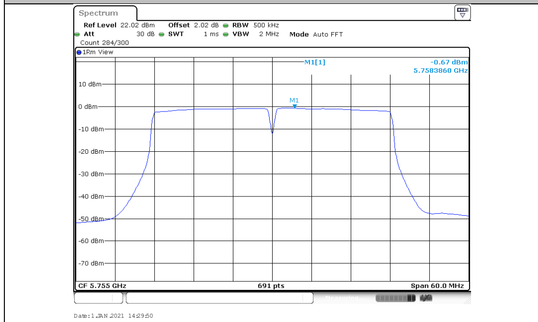
11AC40MIMO_Ant2_5755
