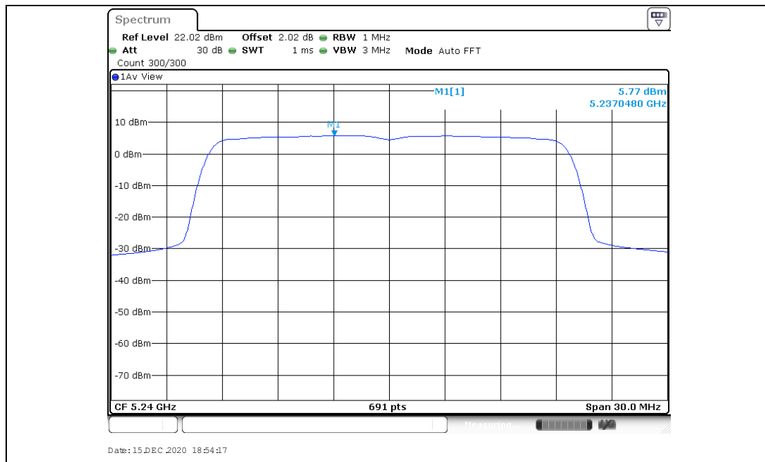
11AX20SISO_Ant2_5240
