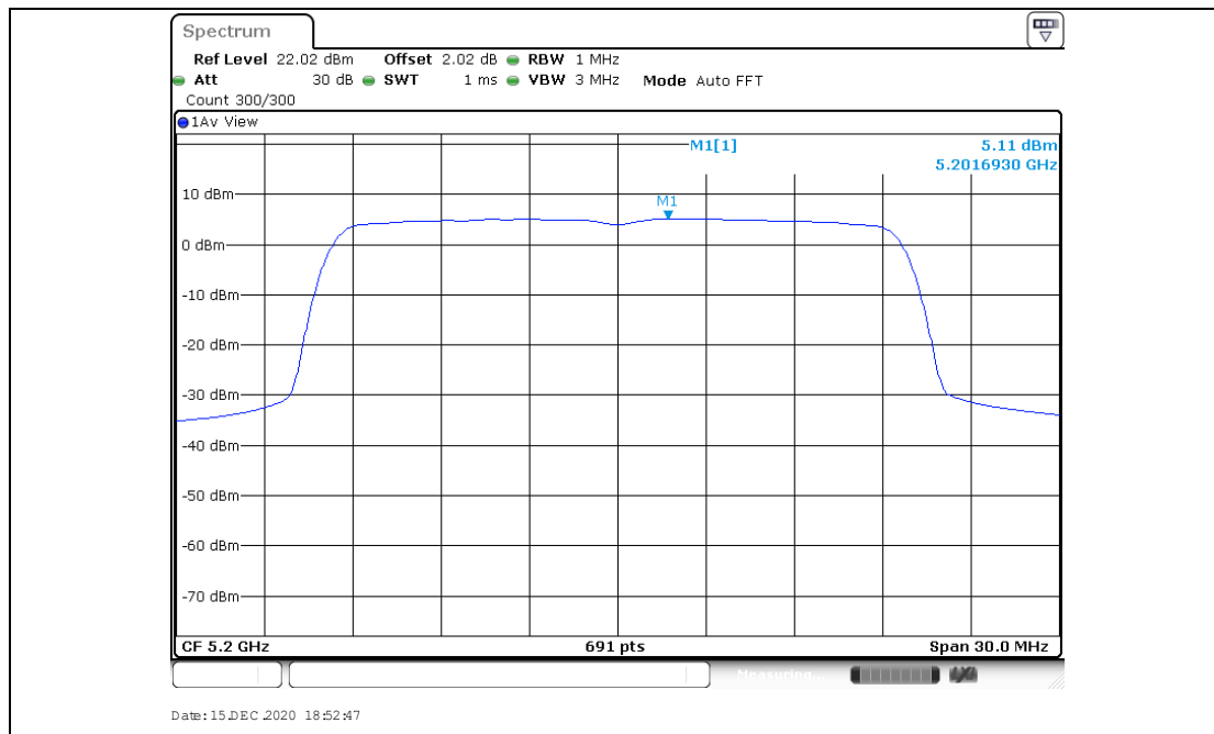
11AX20SISO_Ant2_5200
