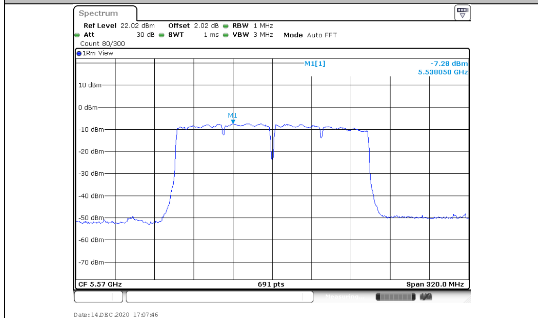
11AC160MIMO_Ant2_5570
