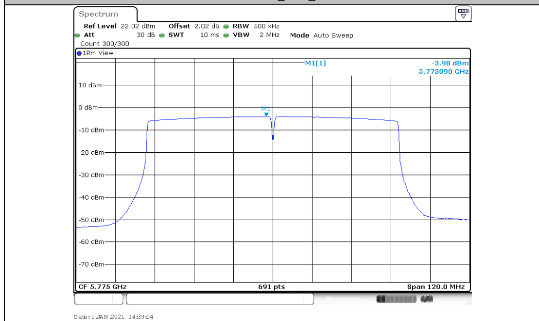
11AC80MIMO_Ant2_5775
