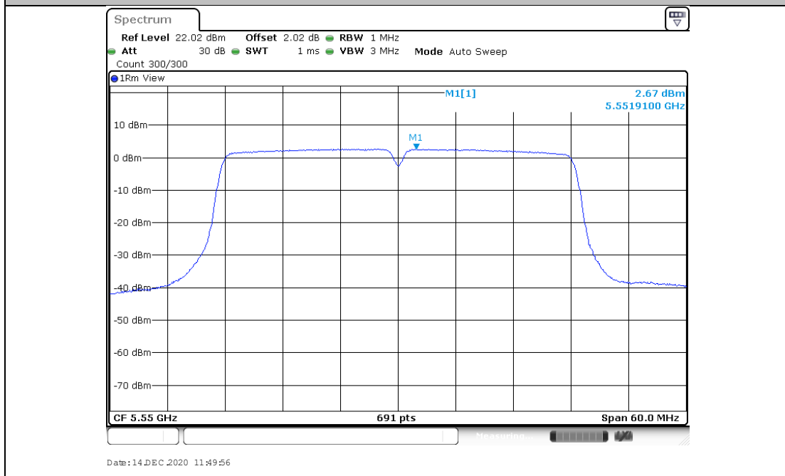
11AC40MIMO_Ant2_5550
