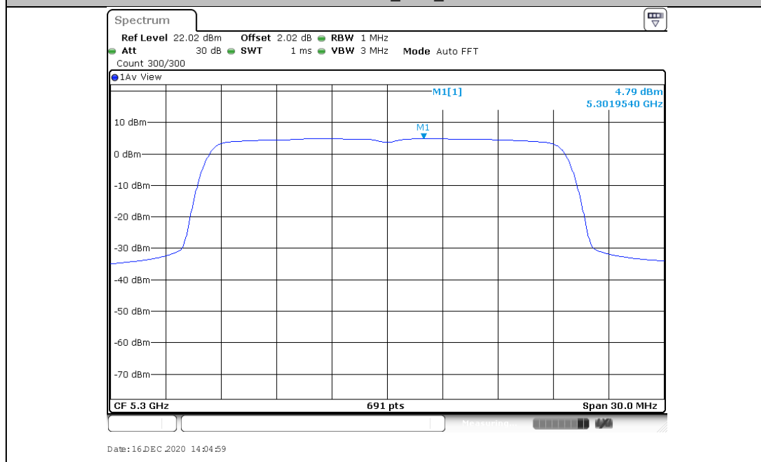
11AX20SISO_Ant2_5300
