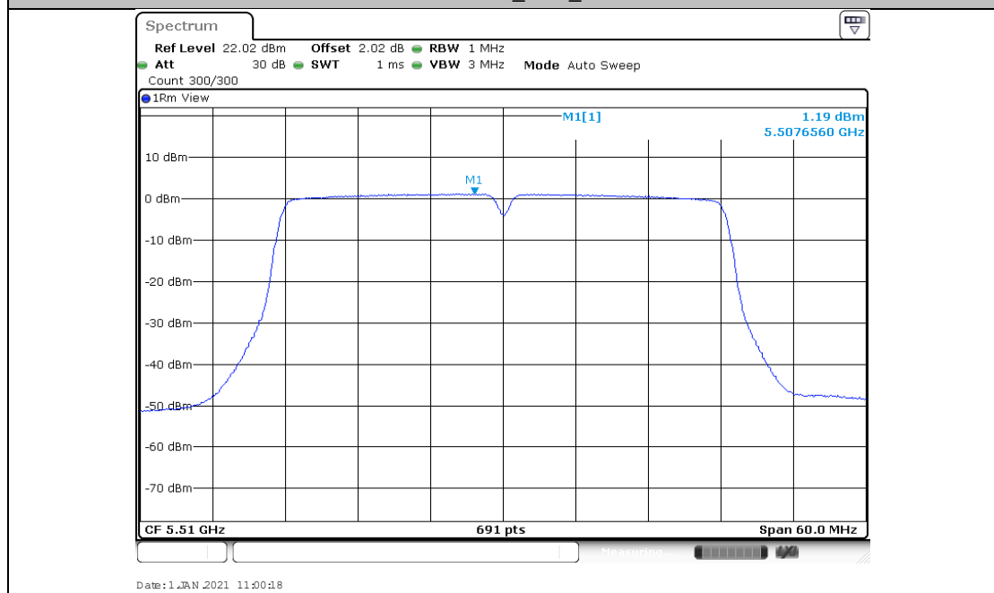
11AC40MIMO_Ant2_5510
