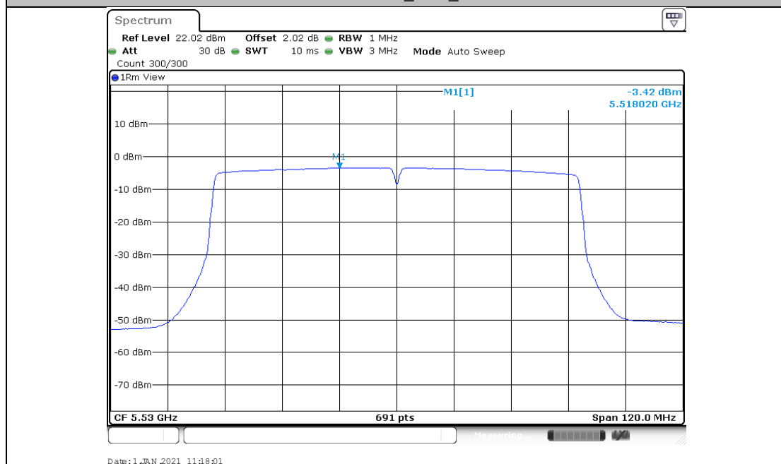
11AC80MIMO_Ant2_5530
