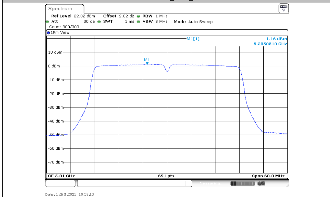
11AC40MIMO_Ant2_5310
