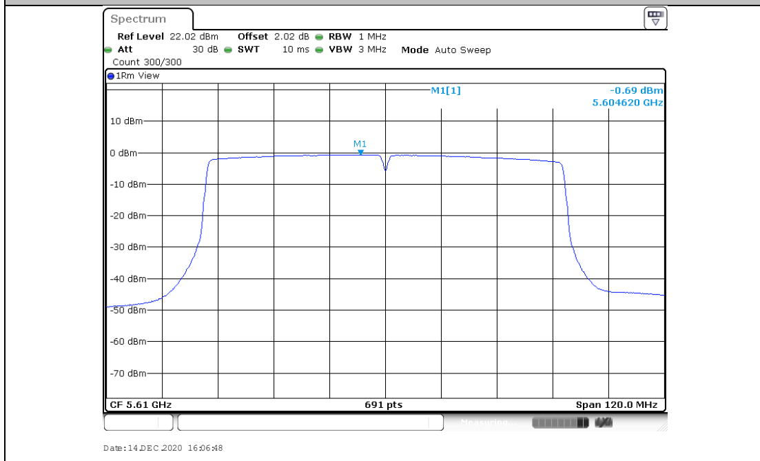
11AC80MIMO_Ant2_5610
