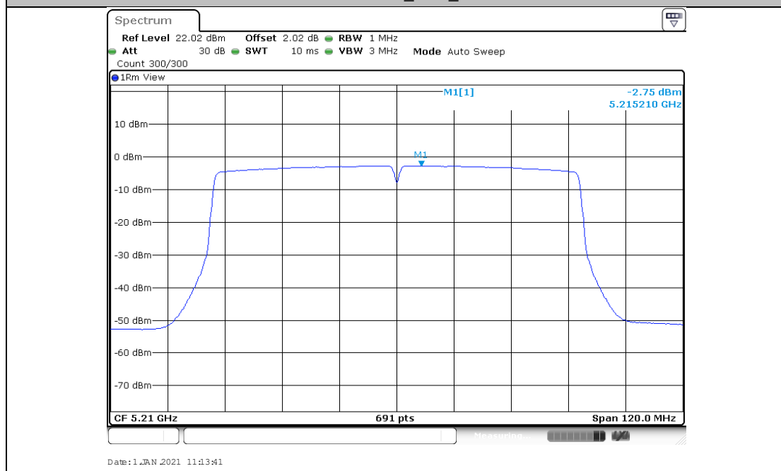
11AC80MIMO_Ant2_5210
