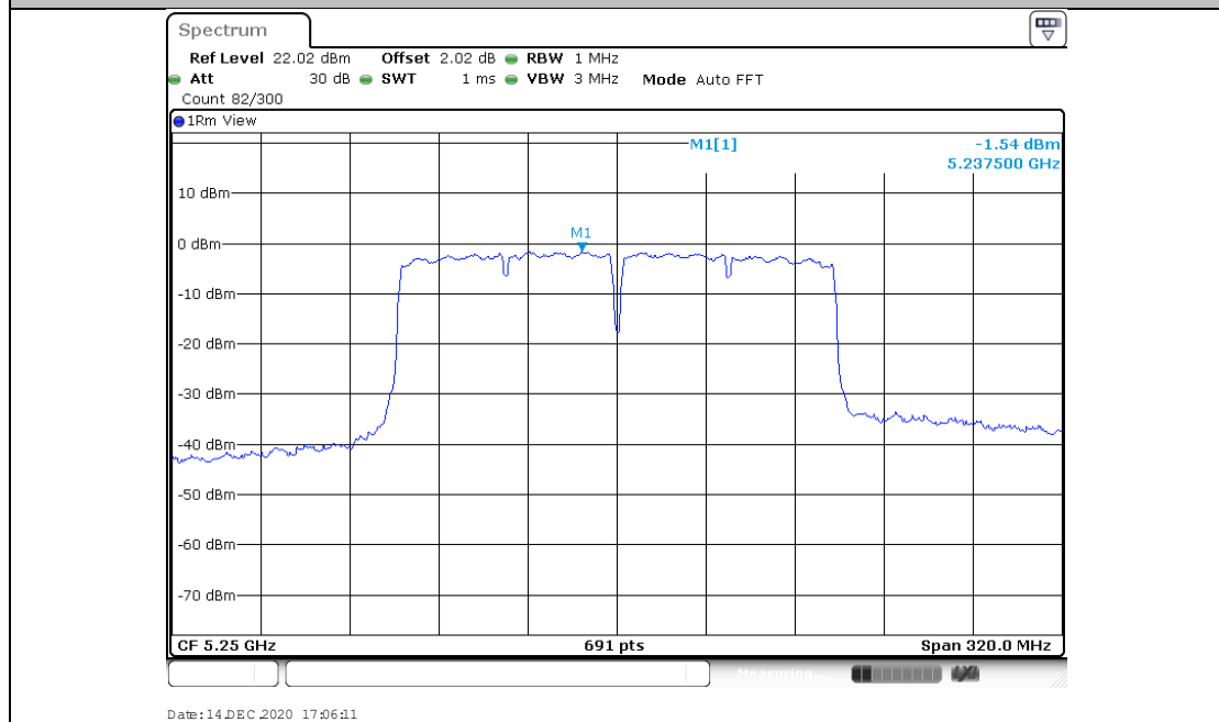
11AC160MIMO_Ant2_5250
