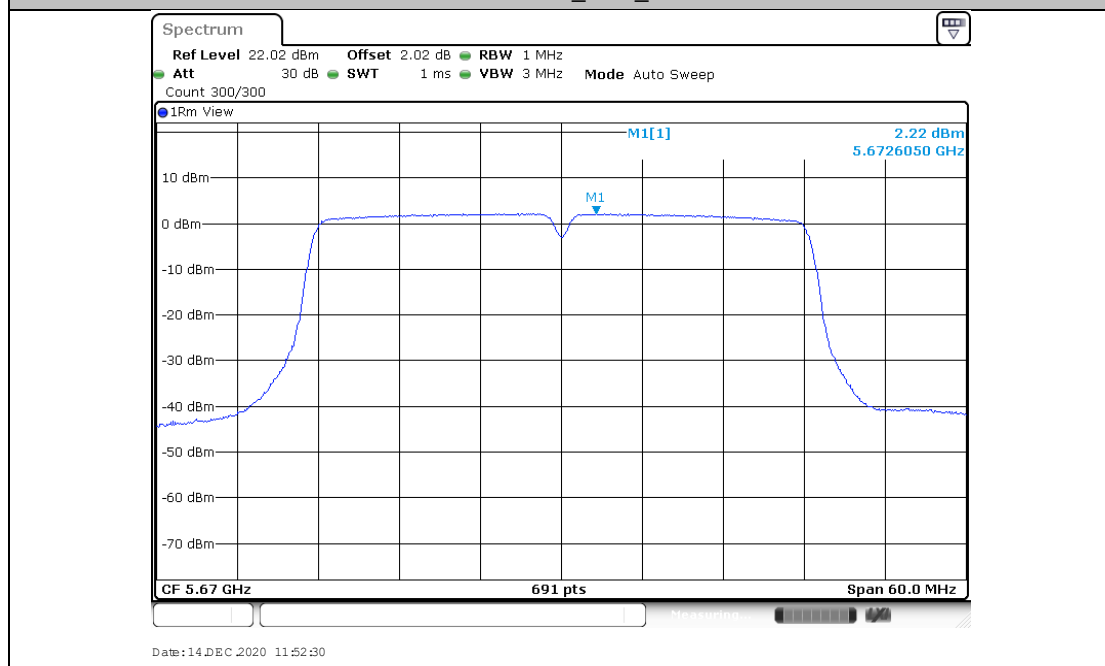
11AC40MIMO_Ant2_5670
