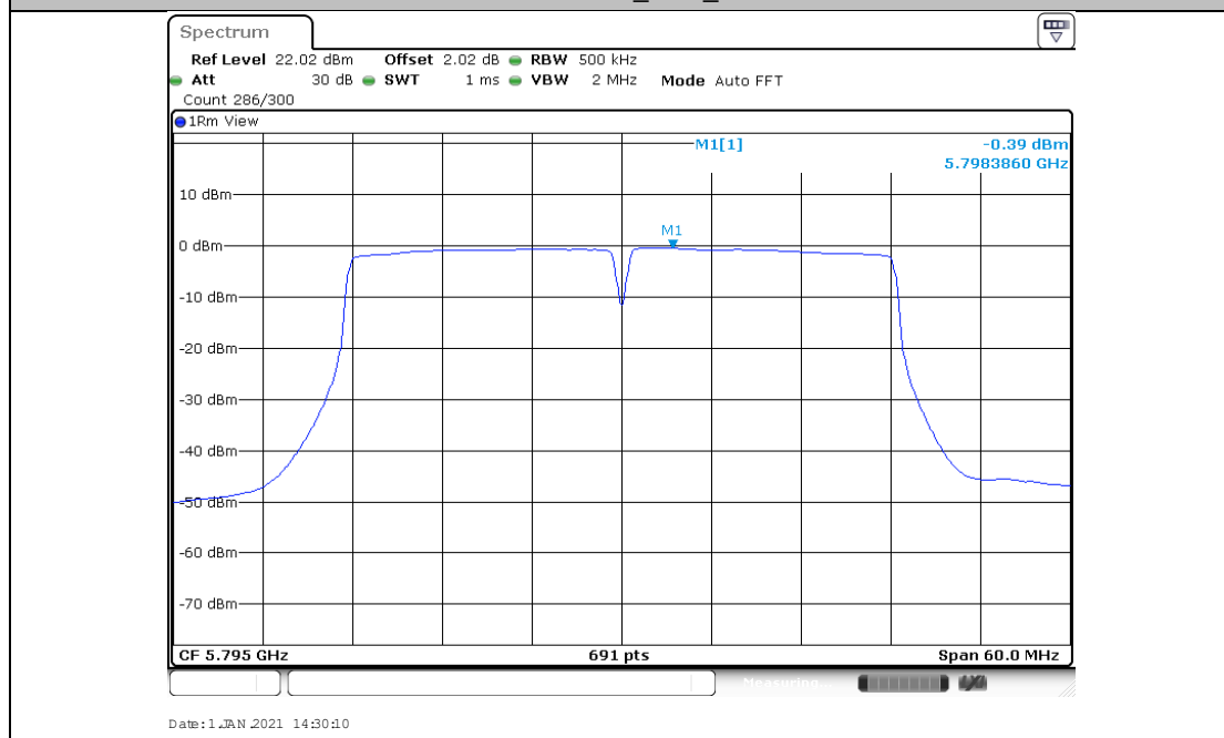
11AC40MIMO_Ant2_5795
