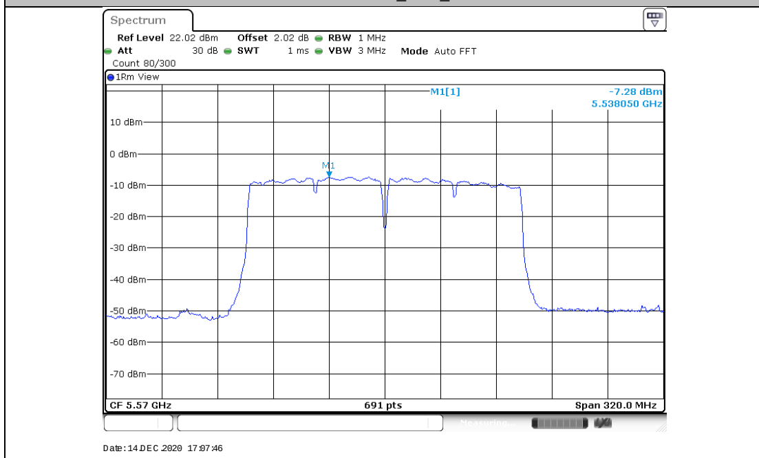
11AC160MIMO_Ant2_5570
