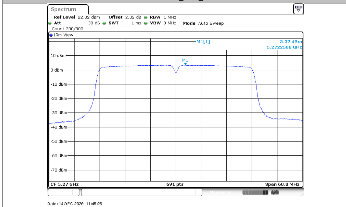
11AC40MIMO_Ant2_5270
