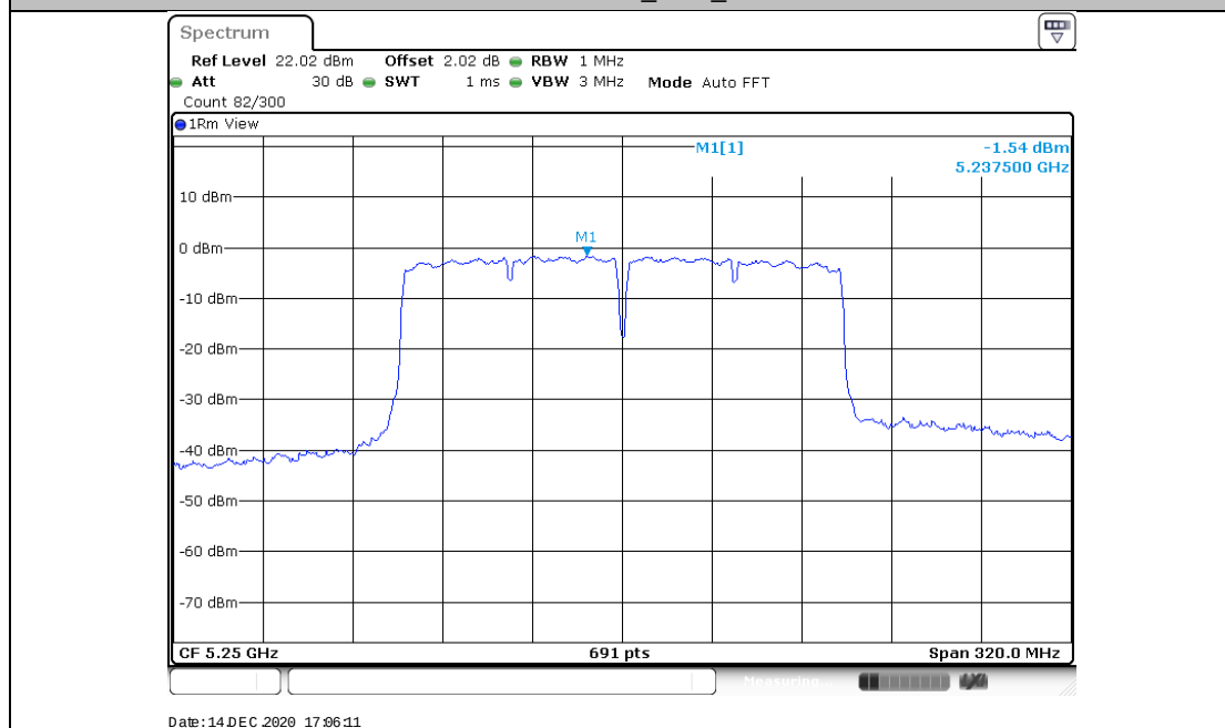
11AC160MIMO_Ant2_5250
