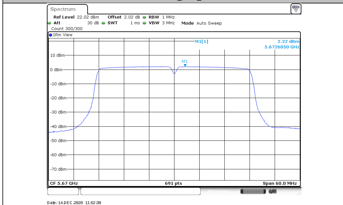
11AC40MIMO_Ant2_5670
