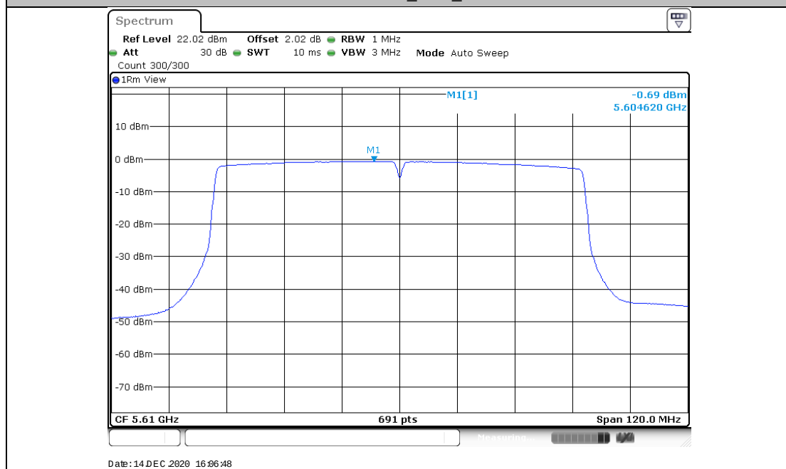
11AC80MIMO_Ant2_5610
