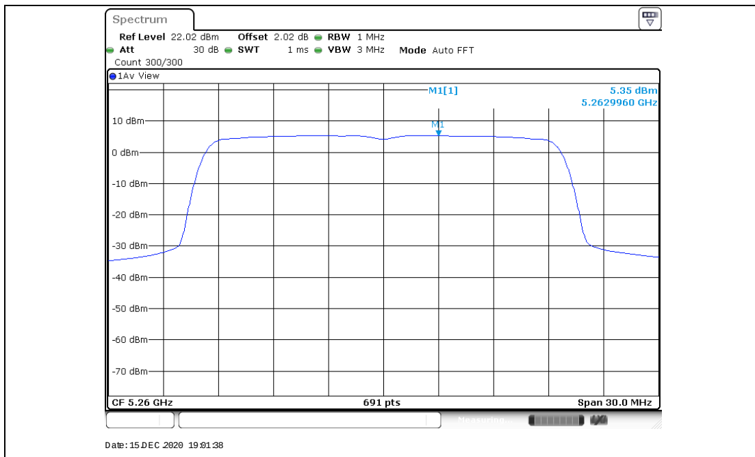
11AX20SISO_Ant2_5260
