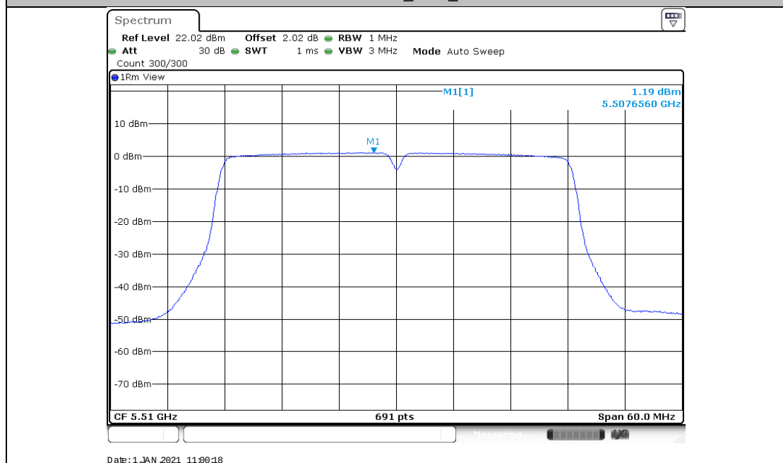
11AC40MIMO_Ant2_5510
