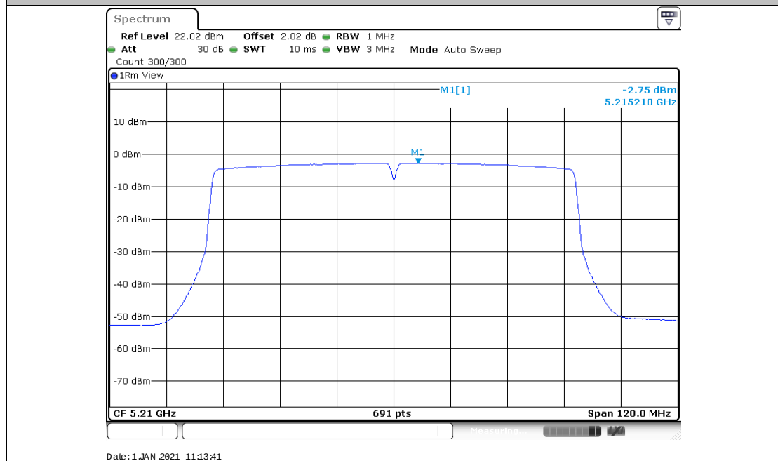
11AC80MIMO_Ant2_5210
