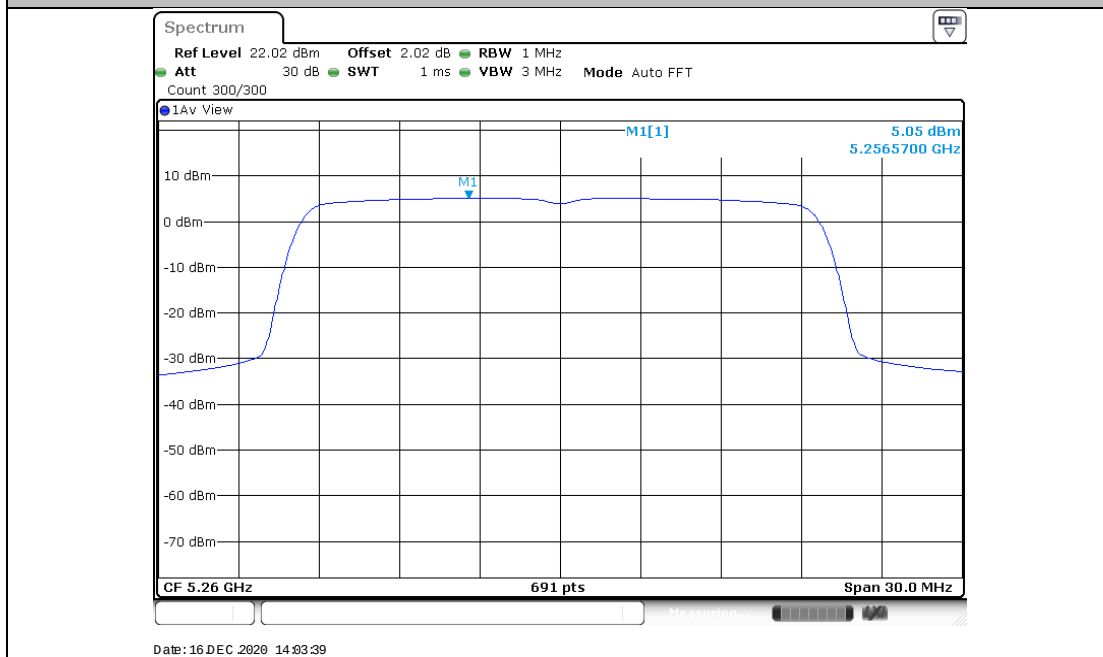
11AX20SISO_Ant1_5300
