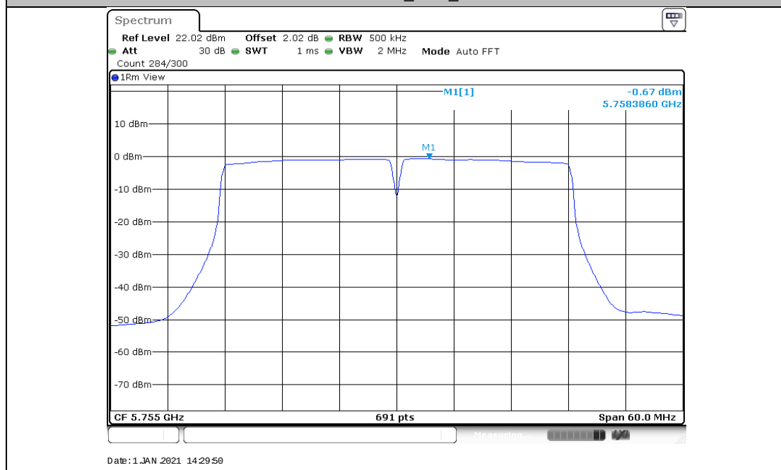
11AC40MIMO_Ant2_5755
