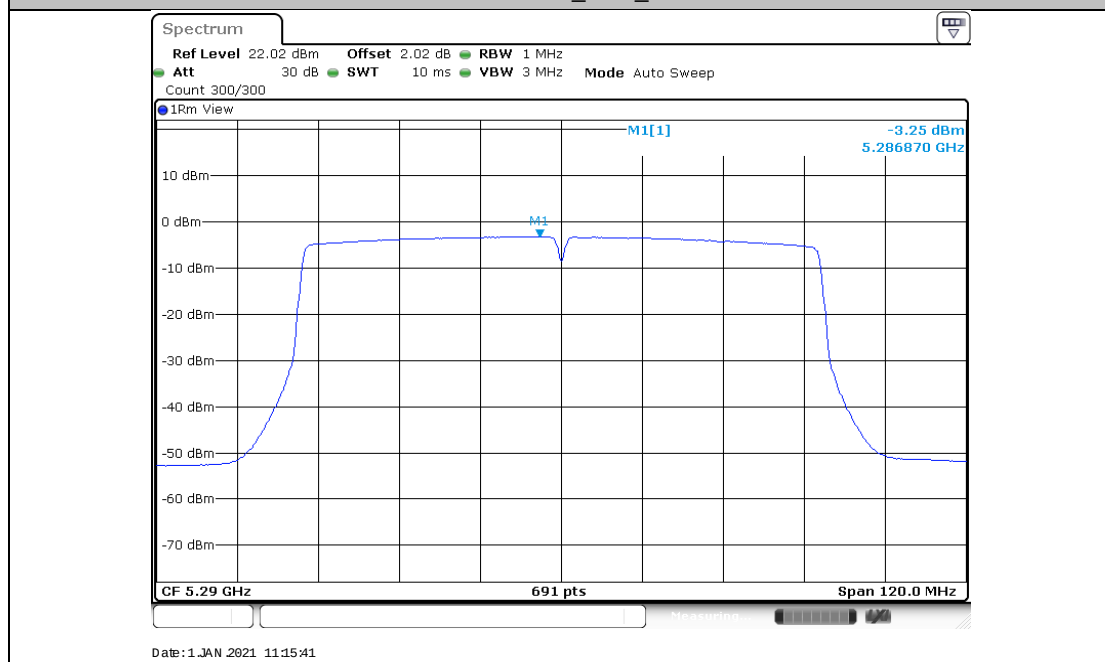
11AC80MIMO_Ant2_5290
