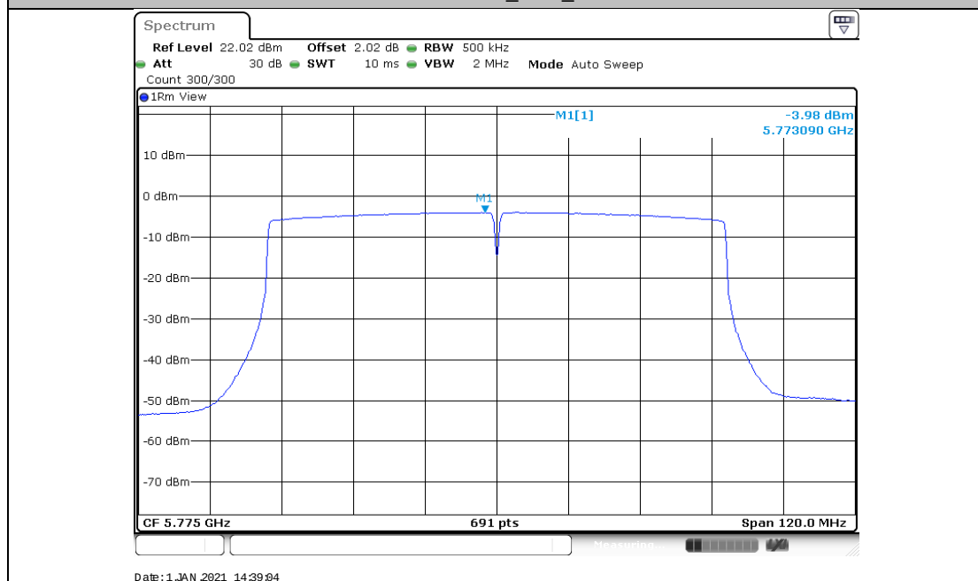
11AC80MIMO_Ant2_5775
