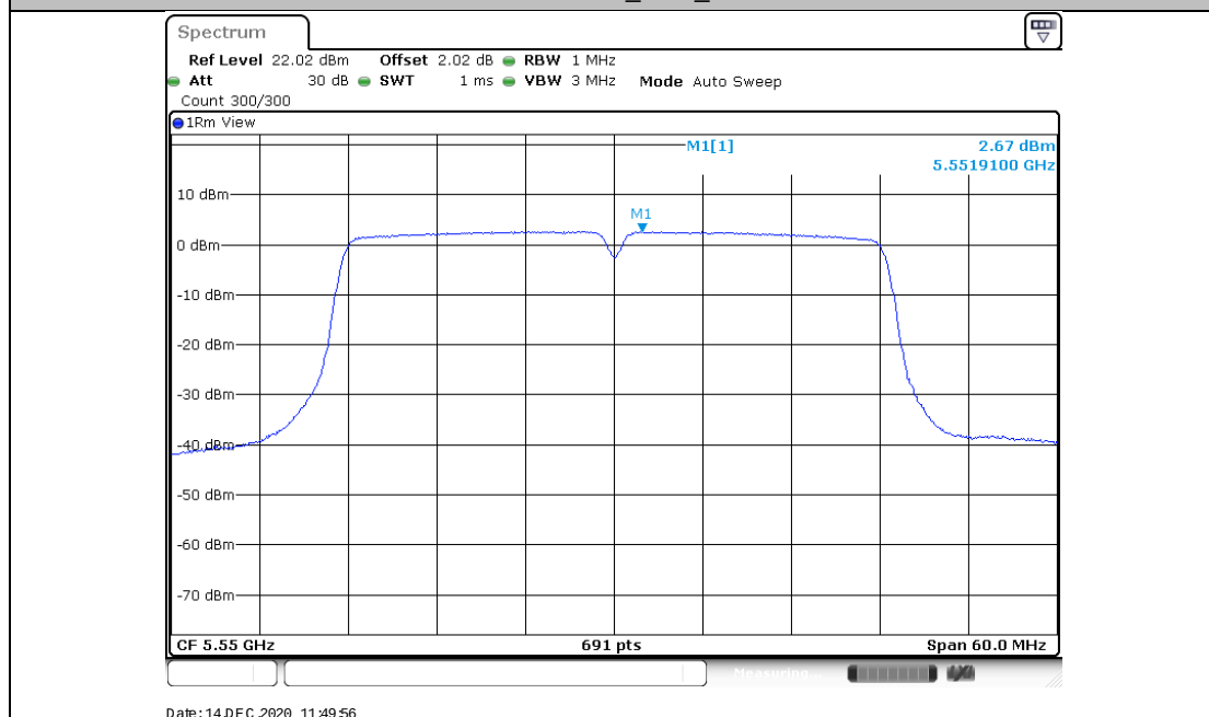
11AC40MIMO_Ant2_5550
