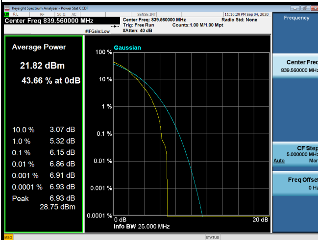
64QAM-20600
