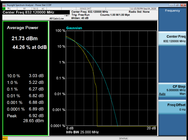
64QAM-20525
