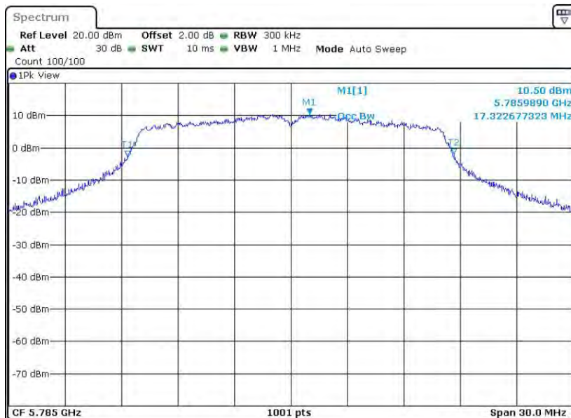
11A_Ant2_5785
