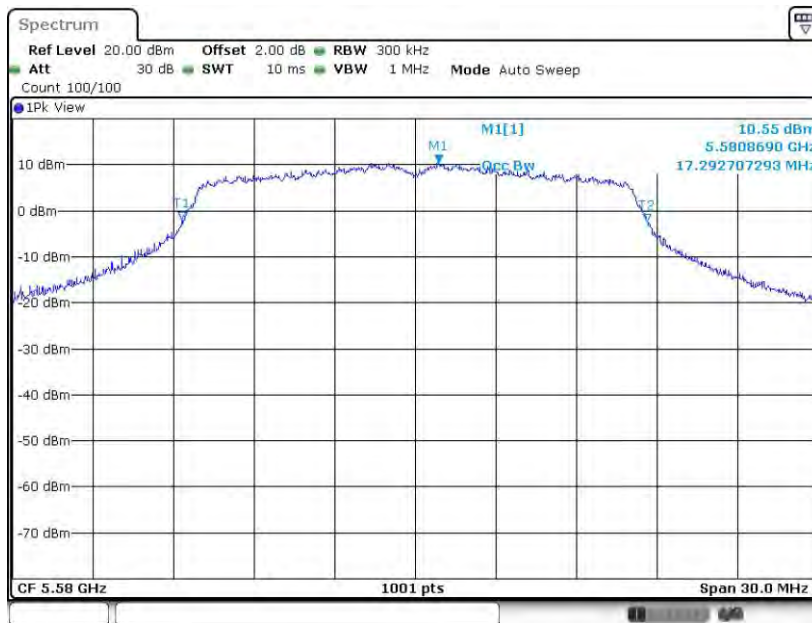
11A_Ant2_5580
