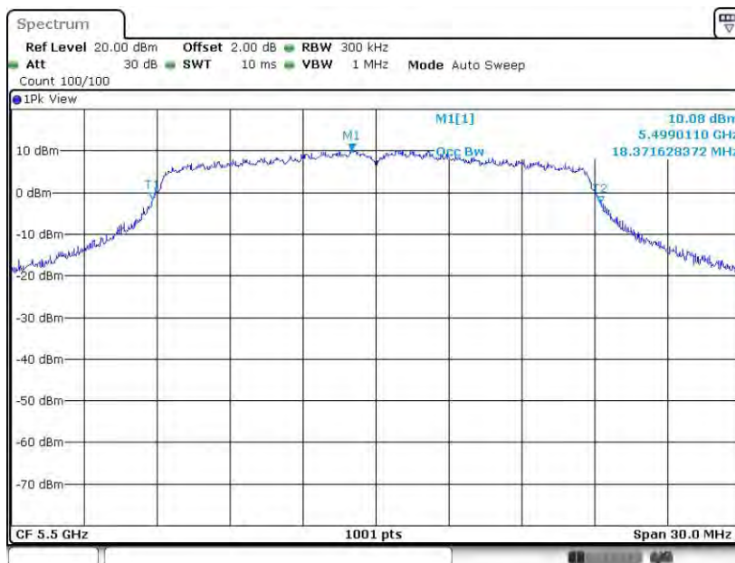
11N20SISO_Ant2_5500
