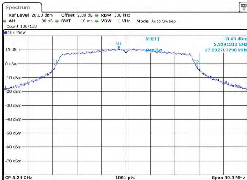
11A_Ant2_5240
