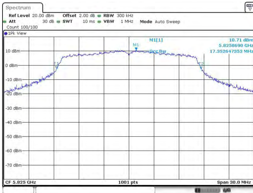
11A_Ant2_5825
