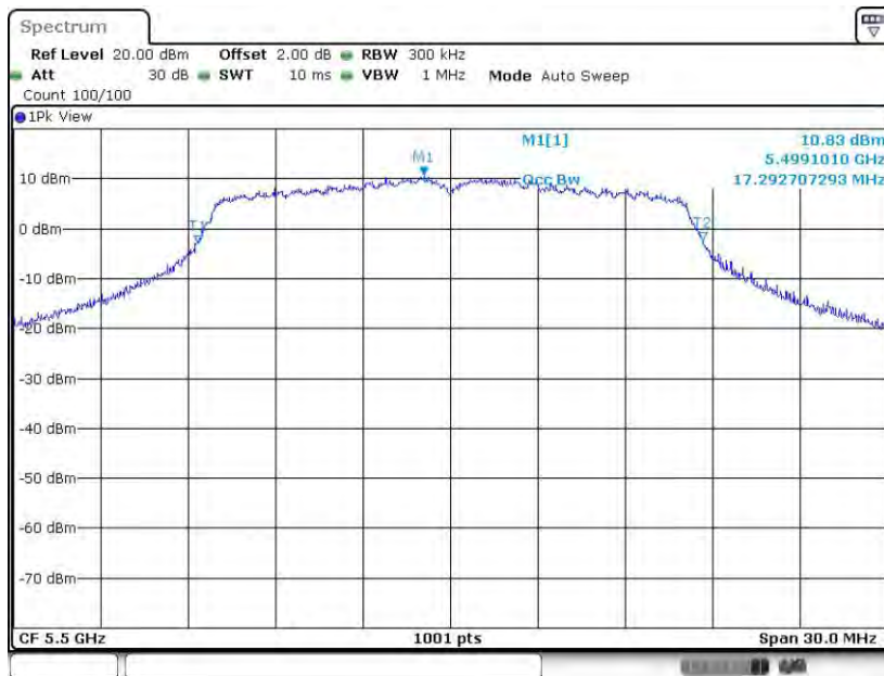
11A_Ant2_5500
