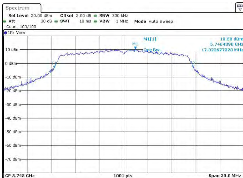
11A_Ant2_5745
