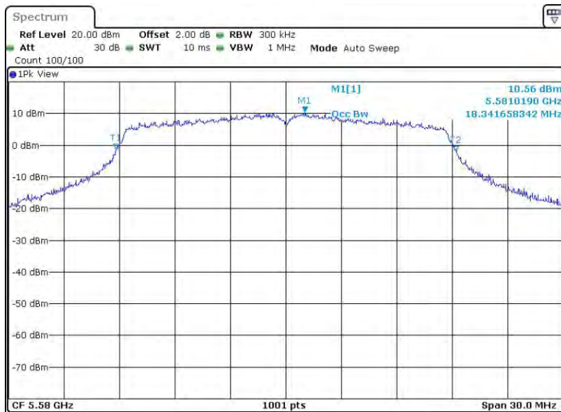
11N20SISO_Ant2_5580
