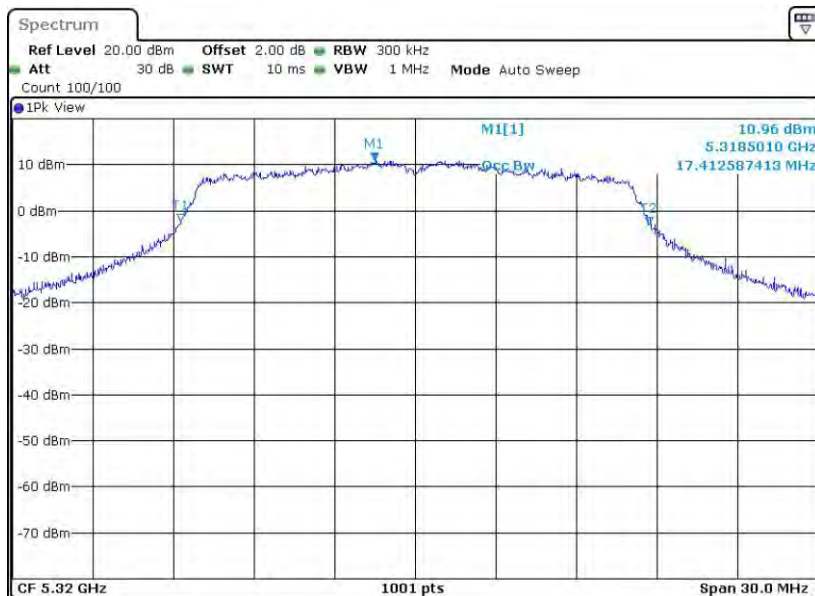
11A_Ant2_5320
