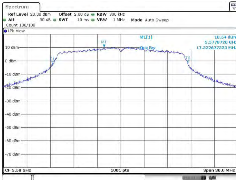
11A_Ant8_5580
