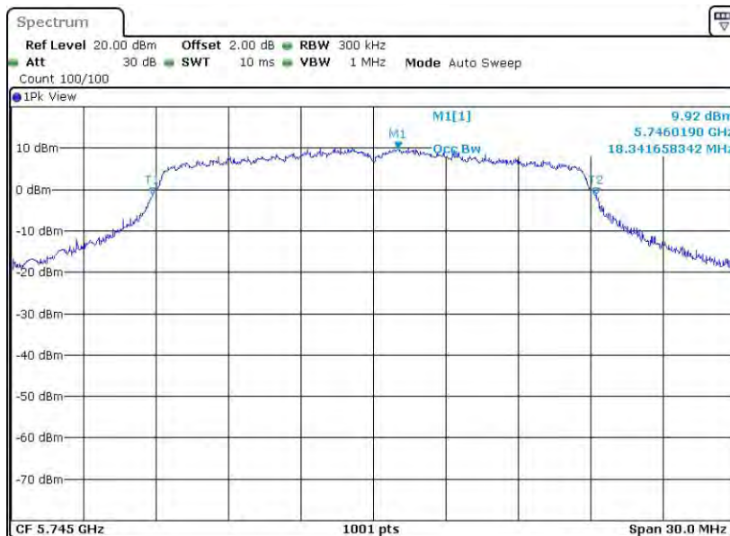
11N20SISO_Ant2_5745
