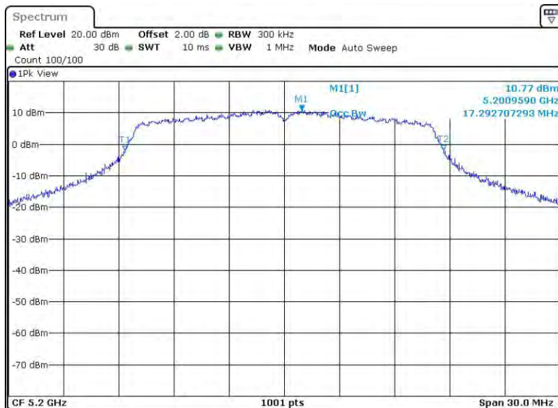
11A_Ant2_5200
