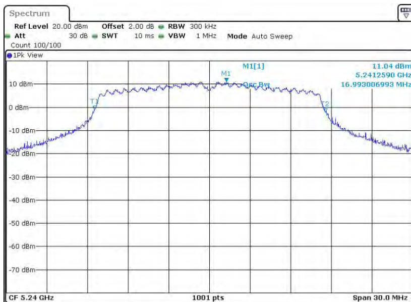
11A-CDD_Ant8_5240
