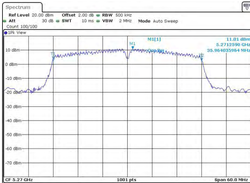
11N40MIMO_Ant8_5270
