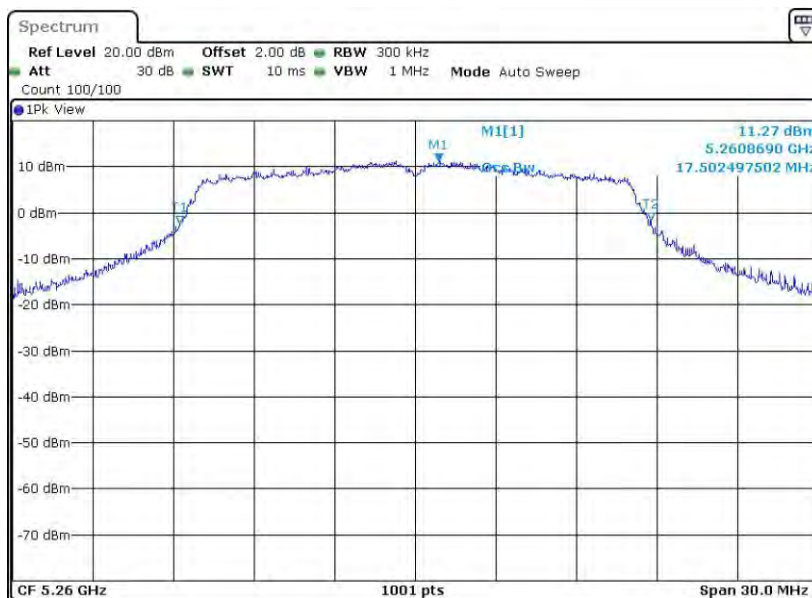
11A-CDD_Ant2_5260
