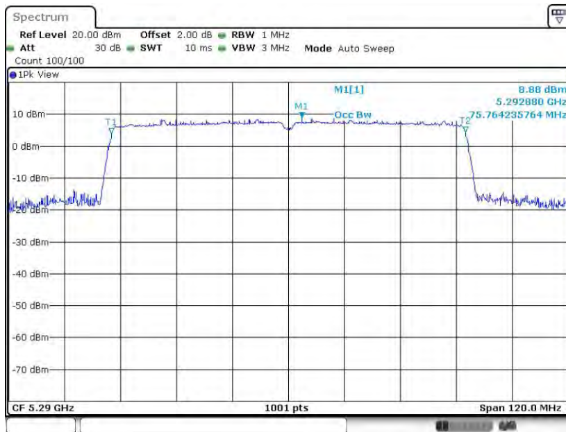
11AC80MIMO_Ant2_5290
