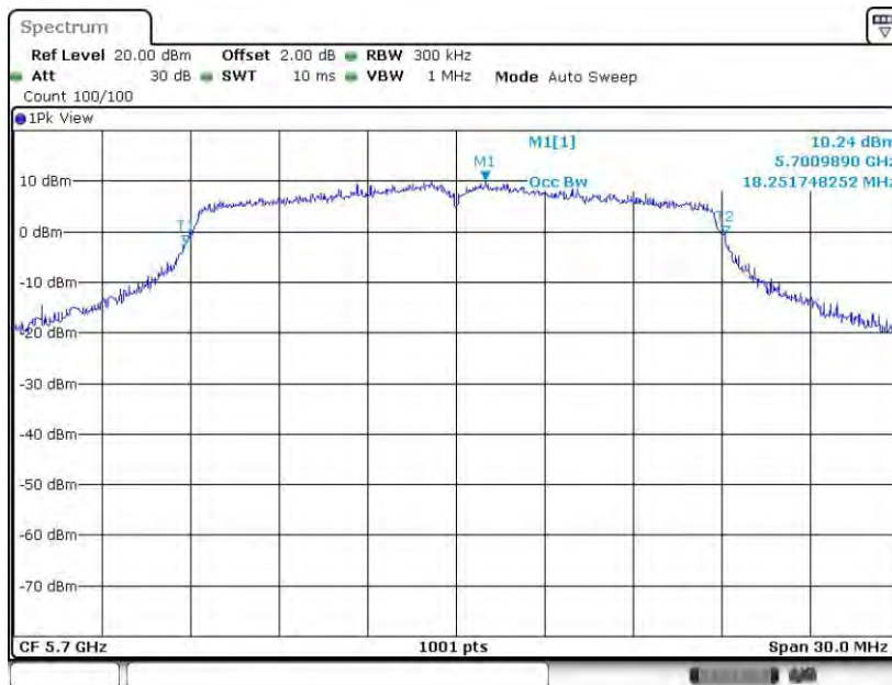
11N20MIMO_Ant2_5700
