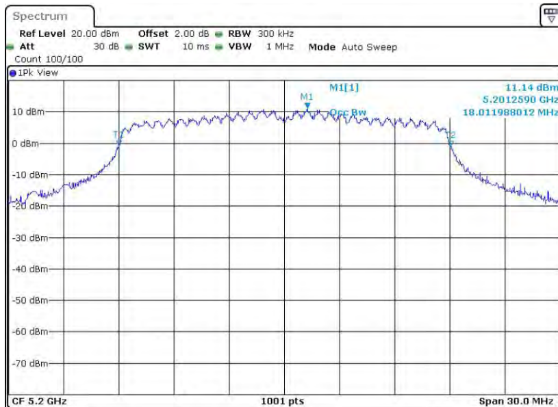
11N20MIMO_Ant8_5200
