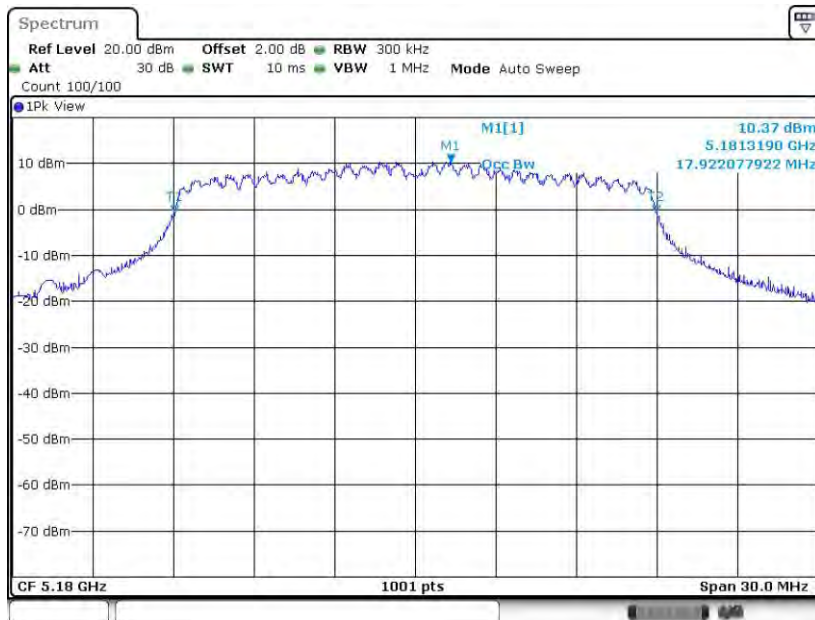
11N20MIMO_Ant8_5180
