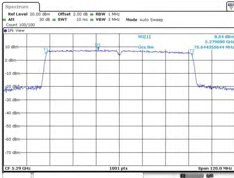
11AC80MIMO_Ant8_5290
