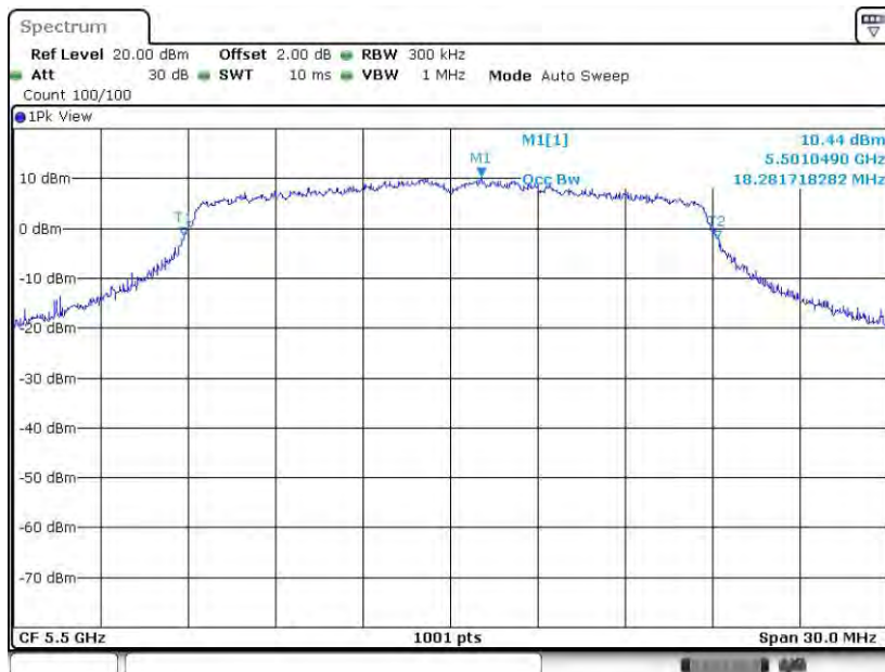
11N20MIMO_Ant2_5500
