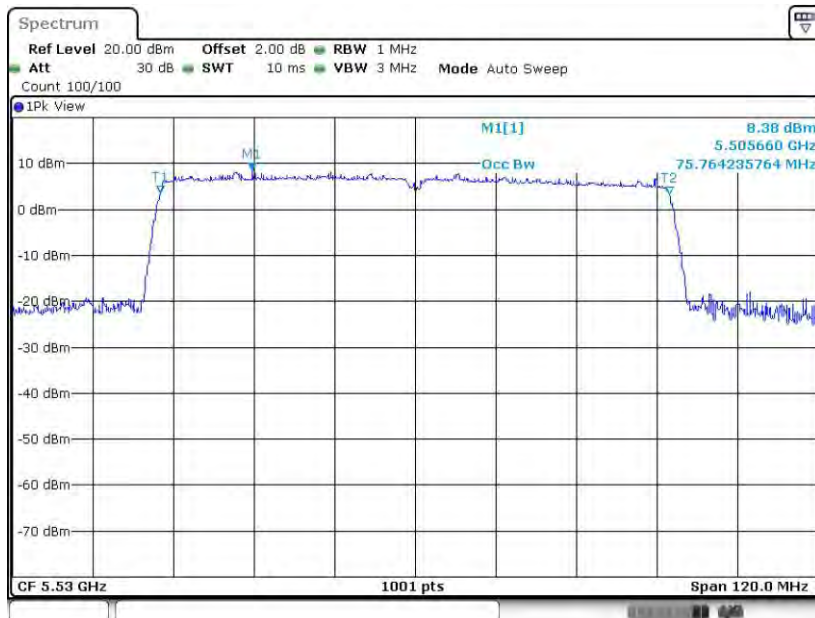
11AC80SISO_Ant8_5530
