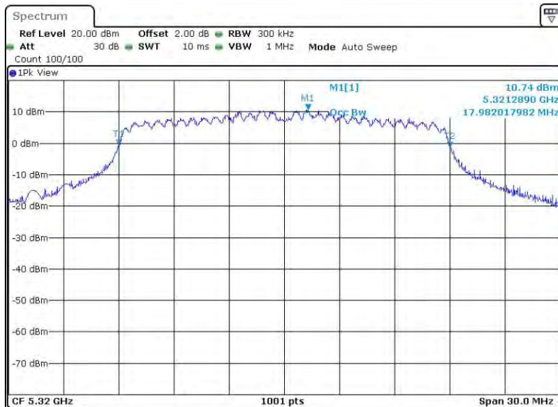
11N20MIMO_Ant8_5320
