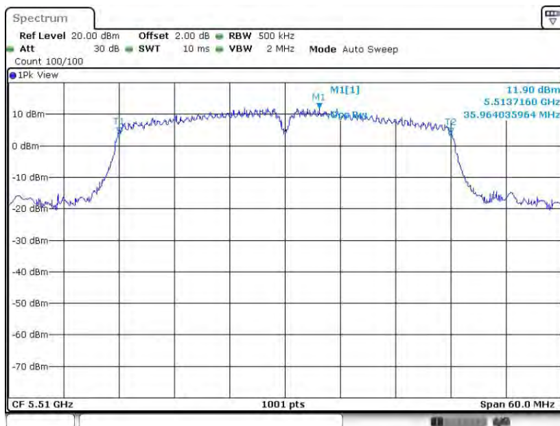
11N40MIMO_Ant8_5510
