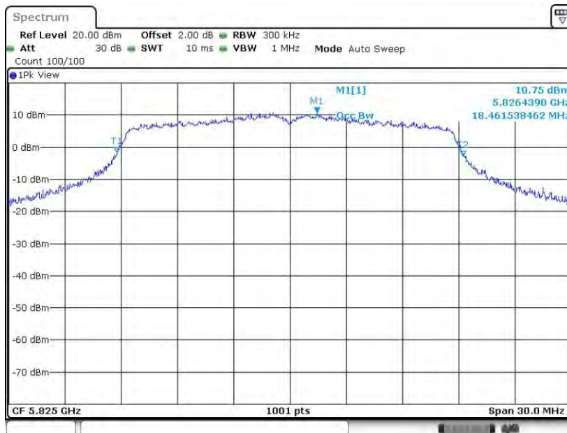
11AC20MIMO_Ant2_5825
