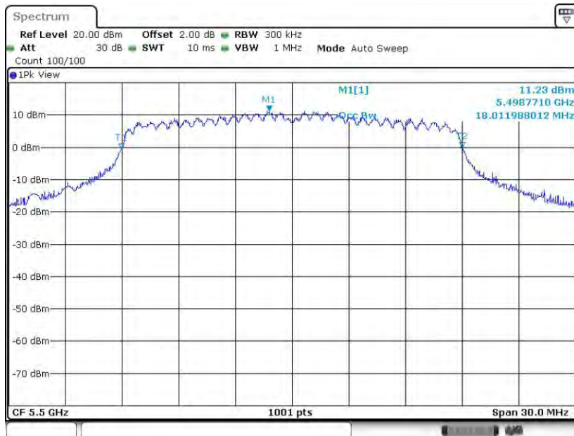
11N20MIMO_Ant8_5500
