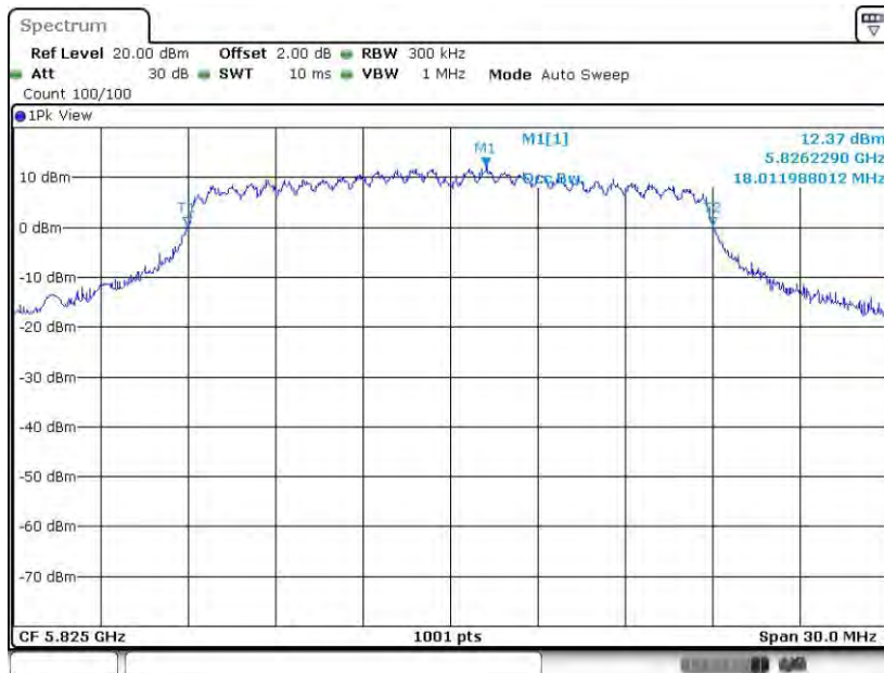
11N20MIMO_Ant8_5825
