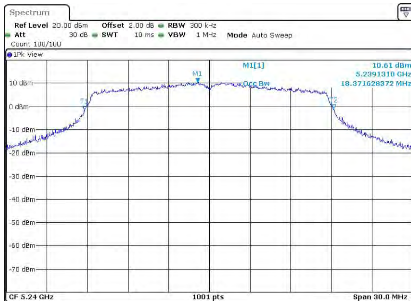
11N20MIMO_Ant2_5240
