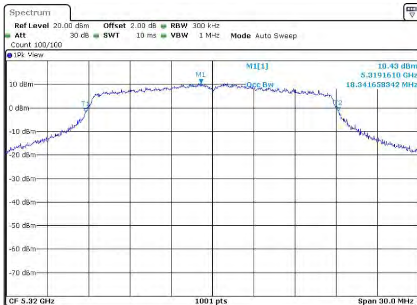
11N20MIMO_Ant2_5320
