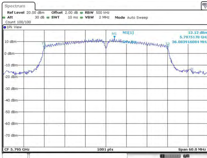
11N40MIMO_Ant8_5795
