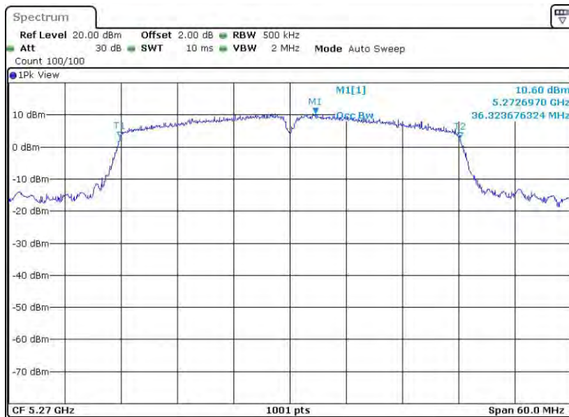
11N40MIMO_Ant2_5270
