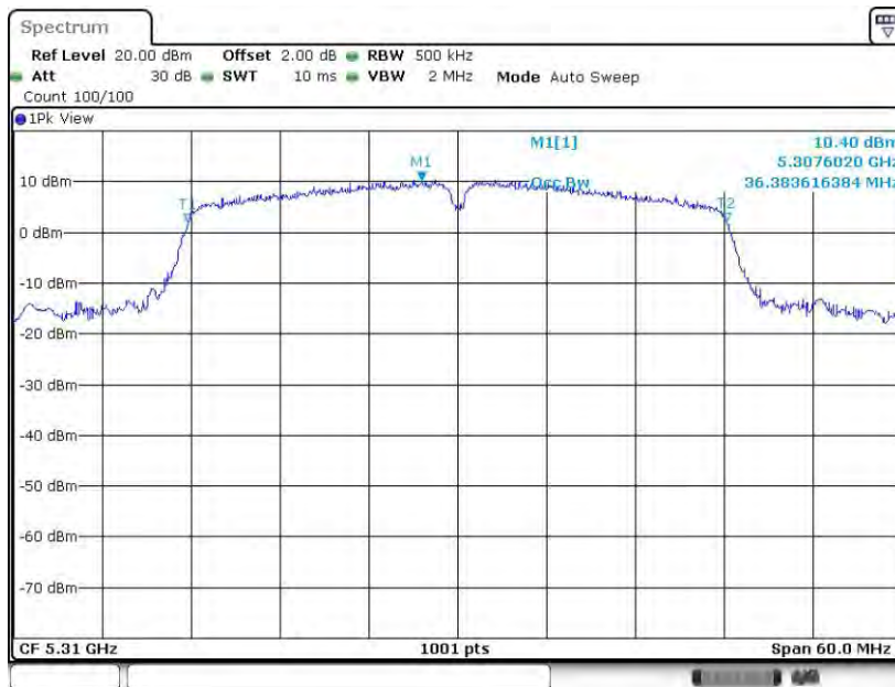
11N40MIMO_Ant2_5310
