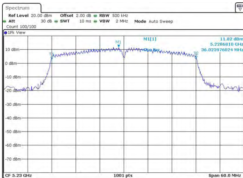
11N40MIMO_Ant8_5230
