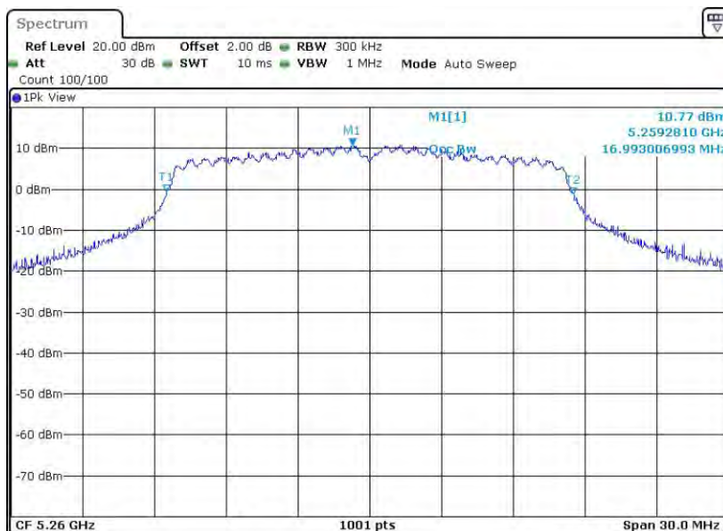
11A-CDD_Ant8_5260
