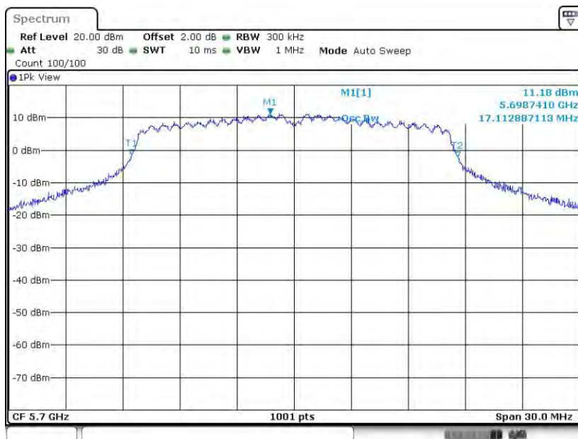
11A-CDD_Ant8_5700
