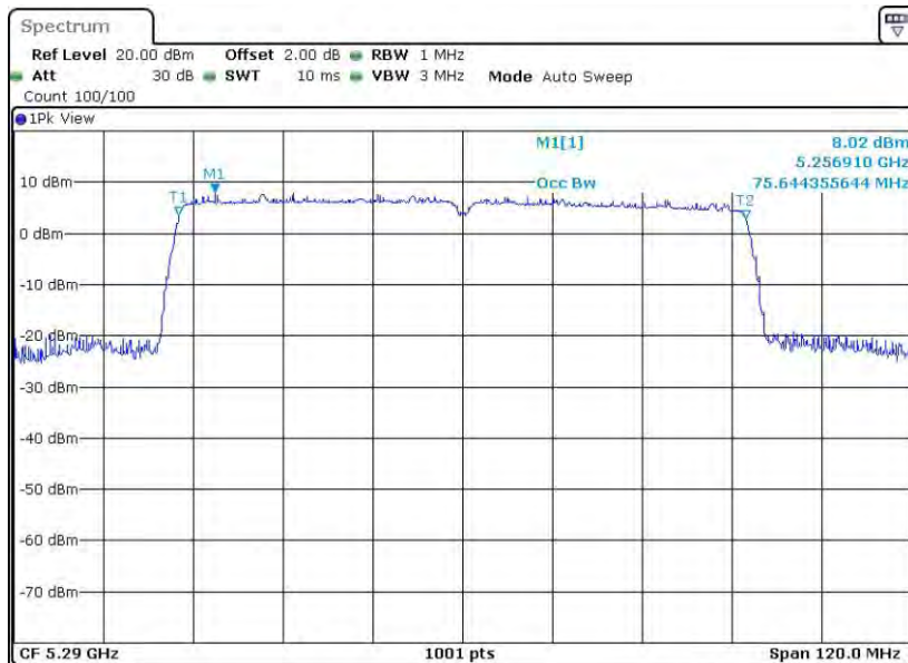
11AC80SISO_Ant8_5290
