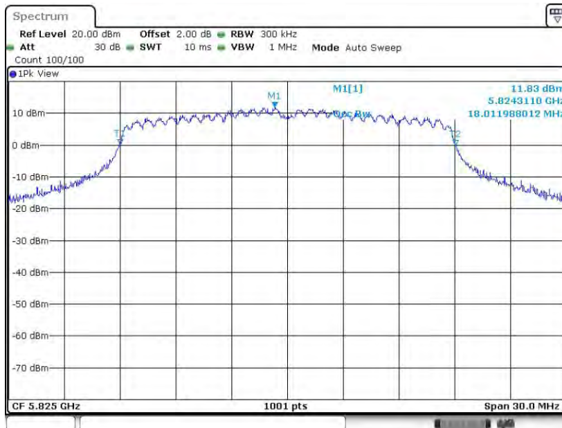
11AC20MIMO_Ant8_5825
