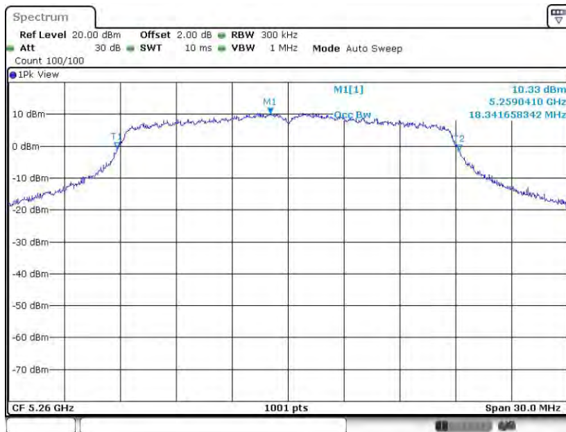
11N20MIMO_Ant2_5260
