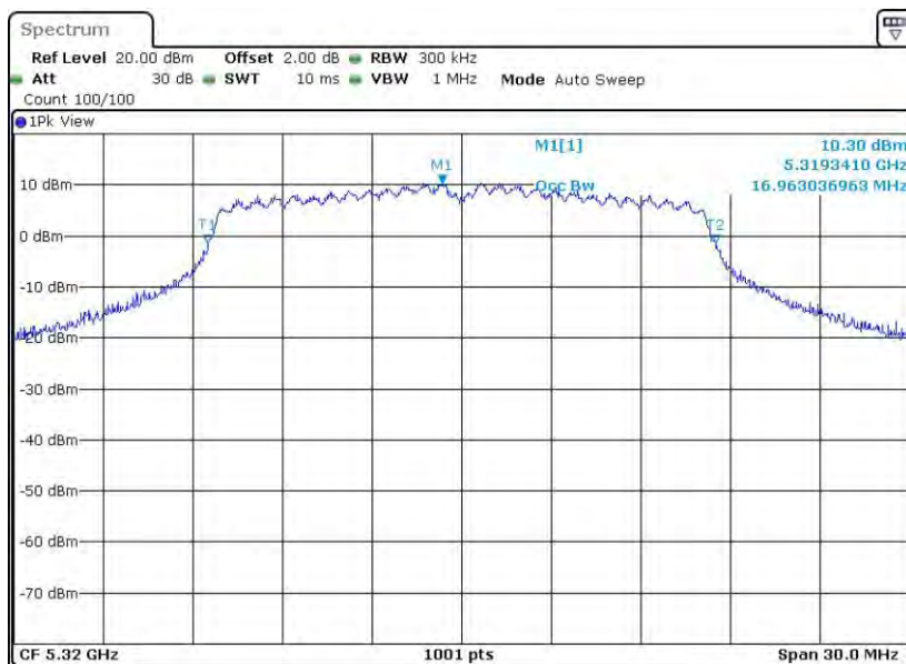
11A-CDD_Ant8_5320
