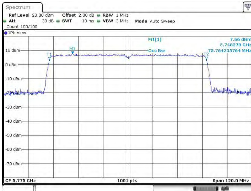
11AC80SISO_Ant8_5775
