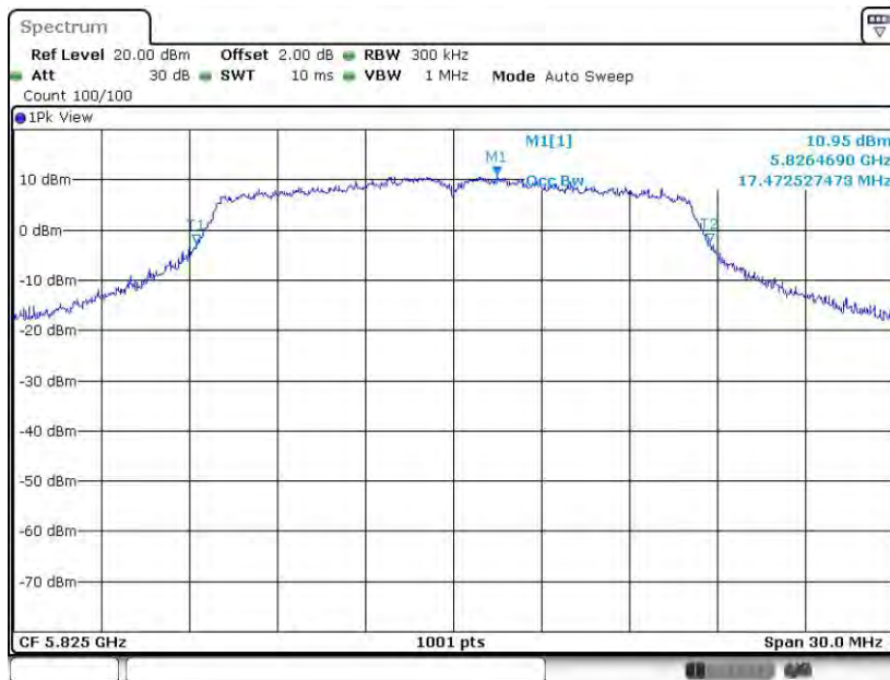
11A-CDD_Ant2_5825
