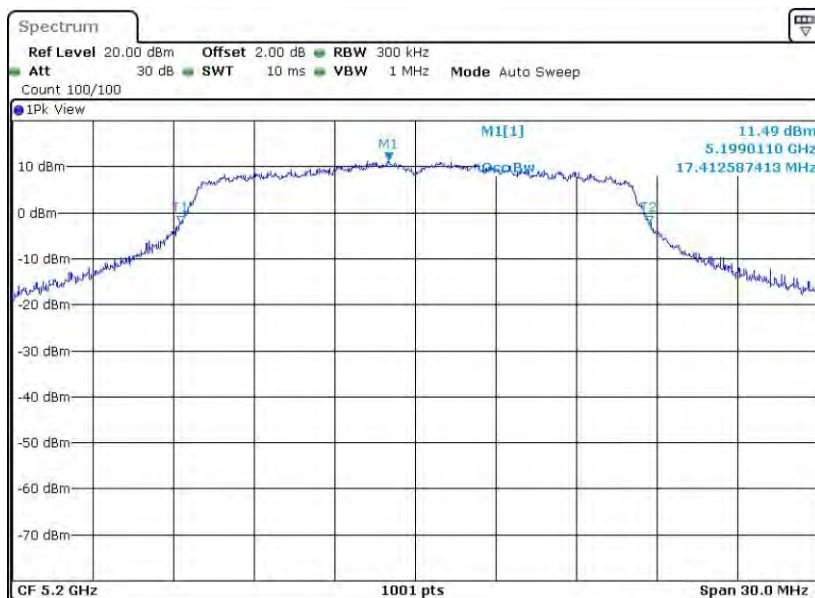
11A-CDD_Ant2_5200
