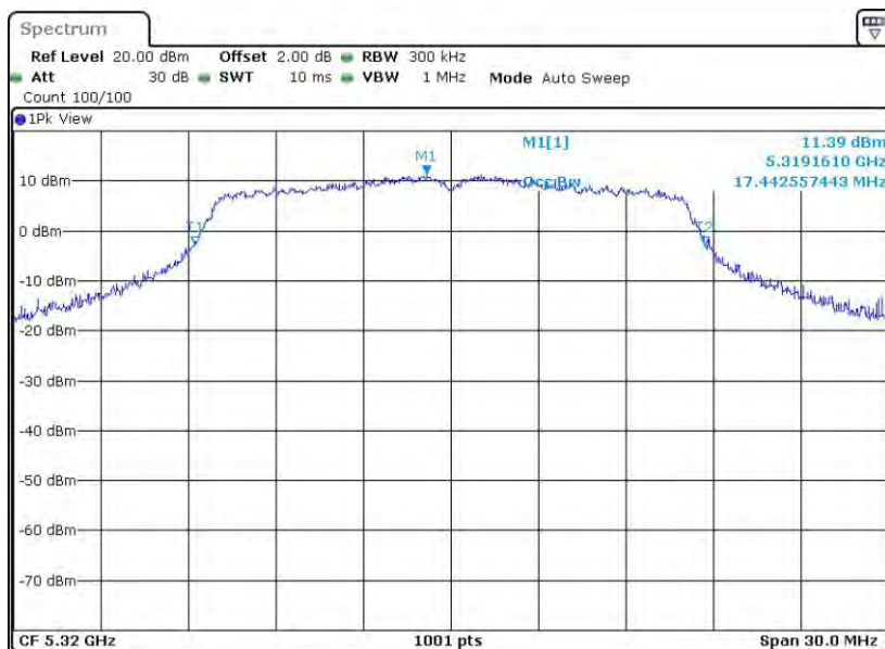
11A-CDD_Ant2_5320
