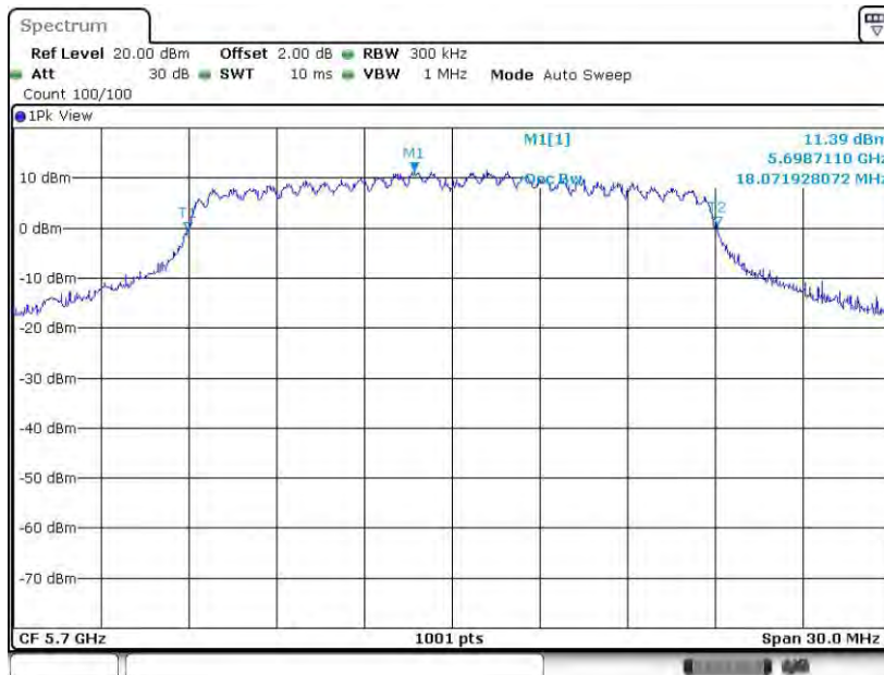
11N20MIMO_Ant8_5700
