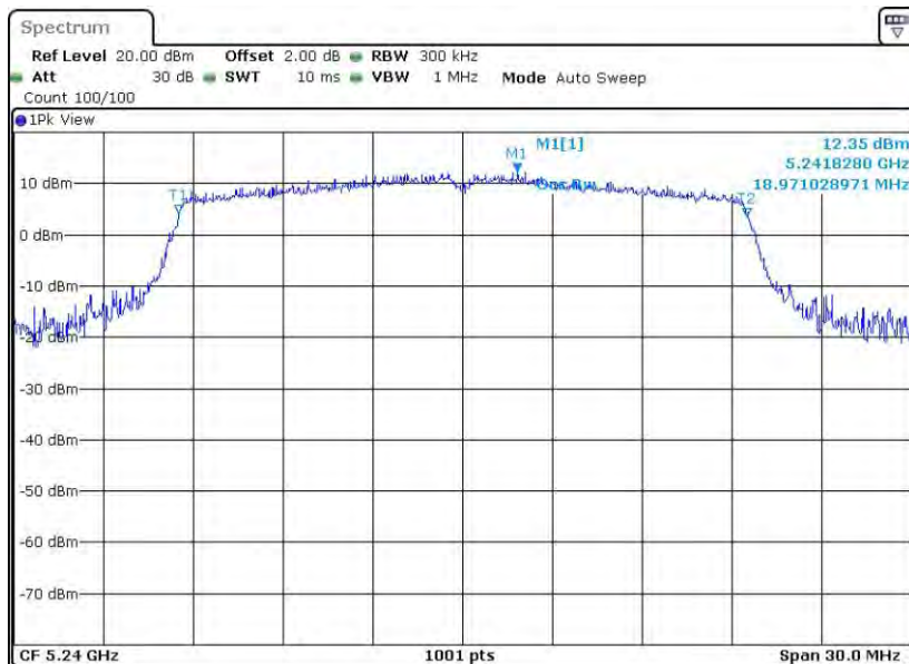
11AX20SISO_Ant2_5240
