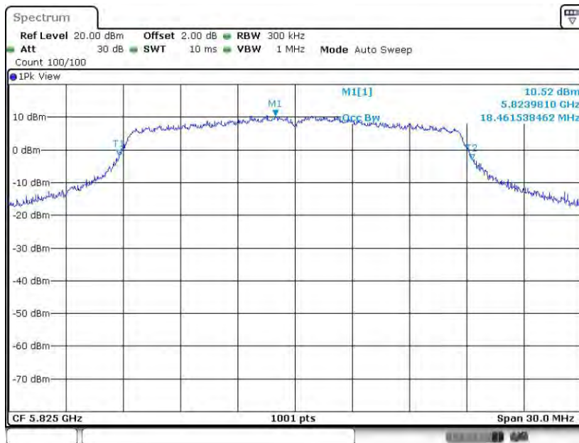
11N20MIMO_Ant2_5825
