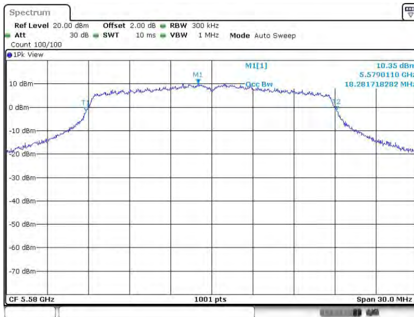
11N20MIMO_Ant2_5580
