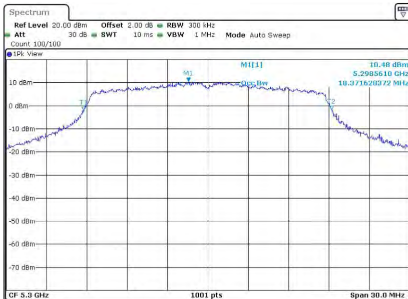
11N20MIMO_Ant2_5300
