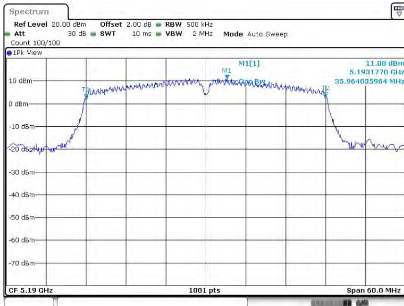
11N40MIMO_Ant8_5190
