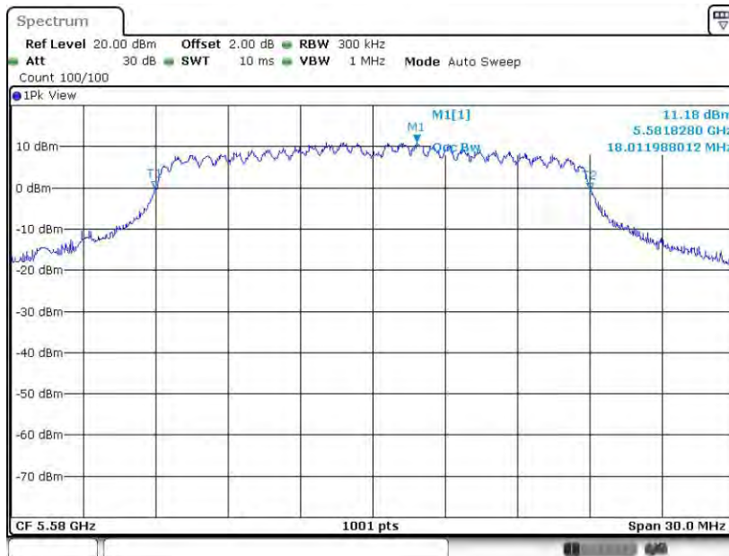
11N20MIMO_Ant8_5580
