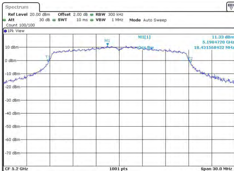
11N20MIMO_Ant2_5200
