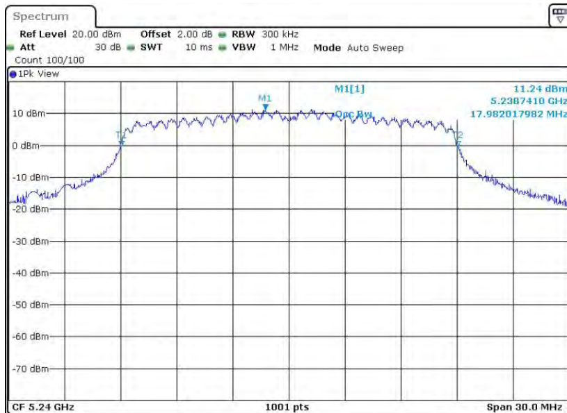
11N20MIMO_Ant8_5240
