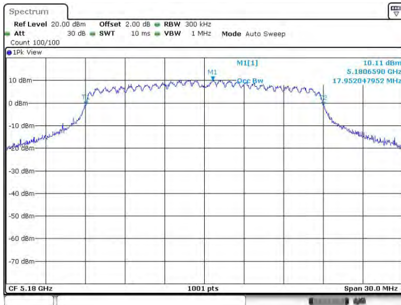
11AC20MIMO_Ant8_5180
