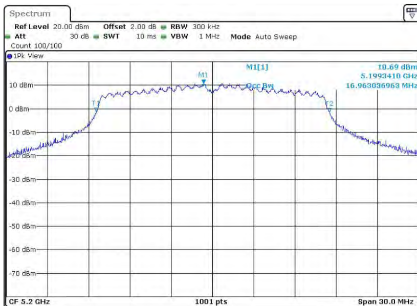
11A-CDD_Ant8_5200
