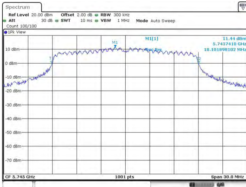
11N20MIMO_Ant8_5745
