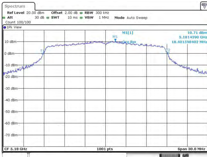
11AC20MIMO_Ant2_5180
