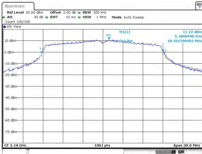
11N20MIMO_Ant2_5180
