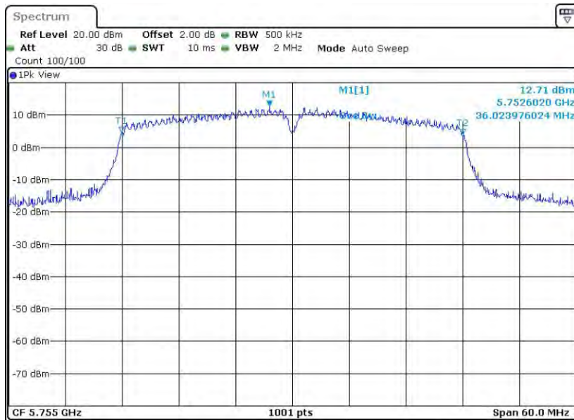
11AC40MIMO_Ant8_5755
