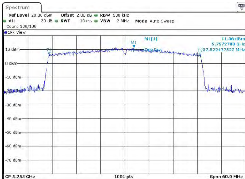
11AX40SISO_Ant2_5755
