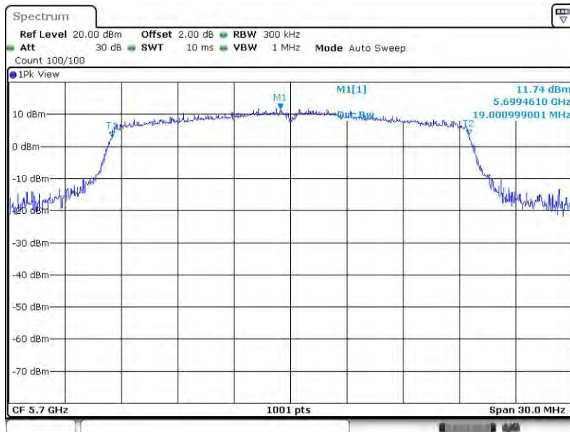
11AX20SISO_Ant8_5700
