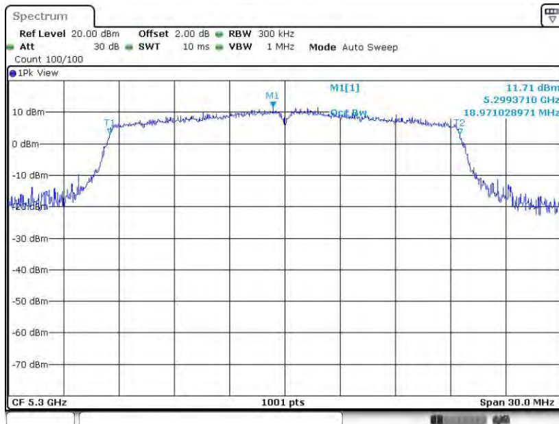
11AX20SISO_Ant8_5300
