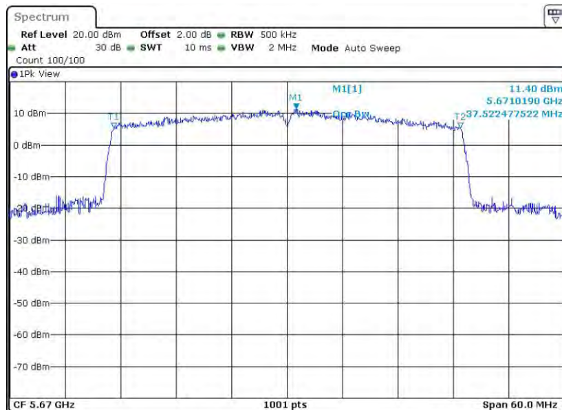
11AX40SISO_Ant2_5670
