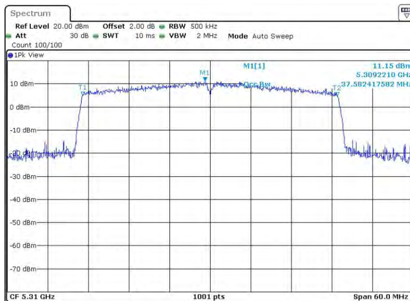
11AX40SISO_Ant8_5310
