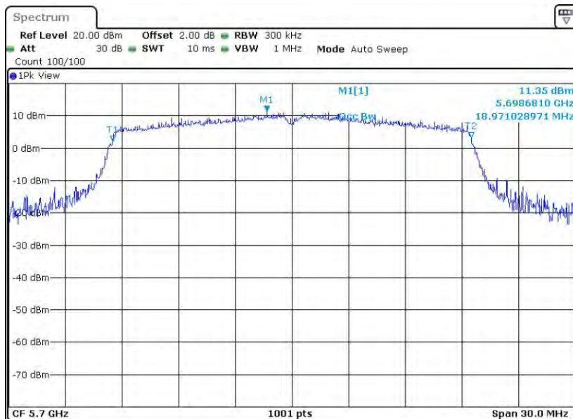
11AX20SISO_Ant2_5700
