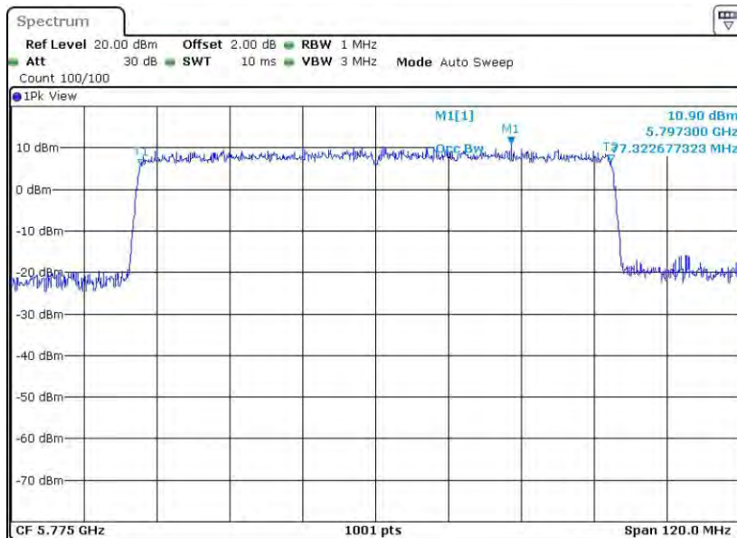
11AX80SISO_Ant8_5775
