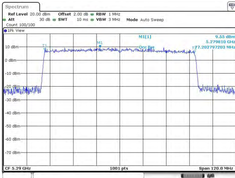
11AX80SISO_Ant8_5290
