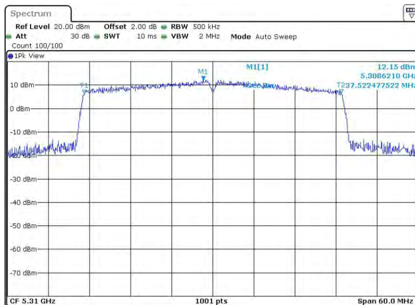
11AX40SISO_Ant2_5310
