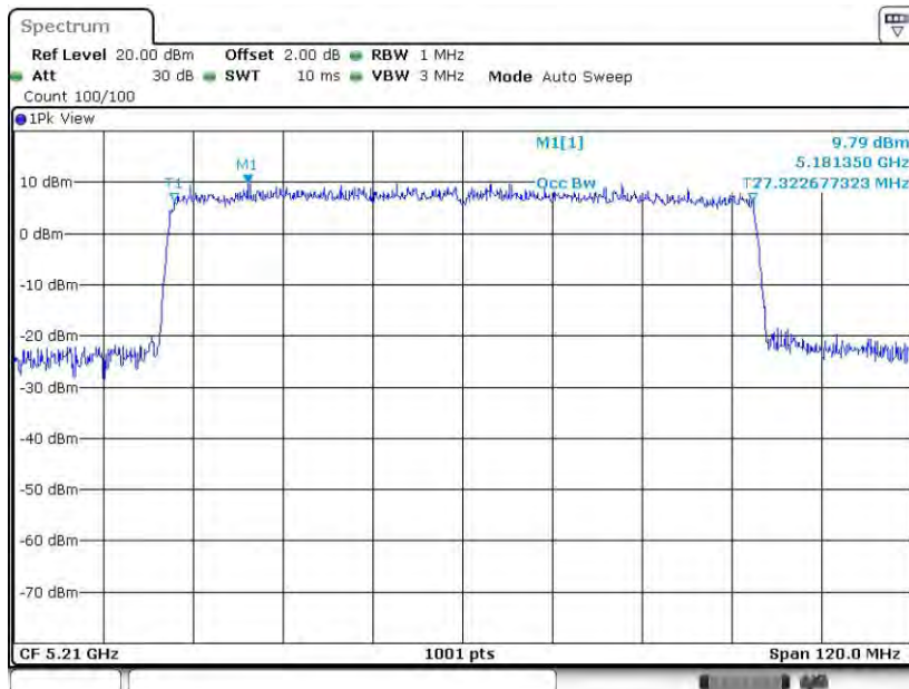
11AX80SISO_Ant8_5210
