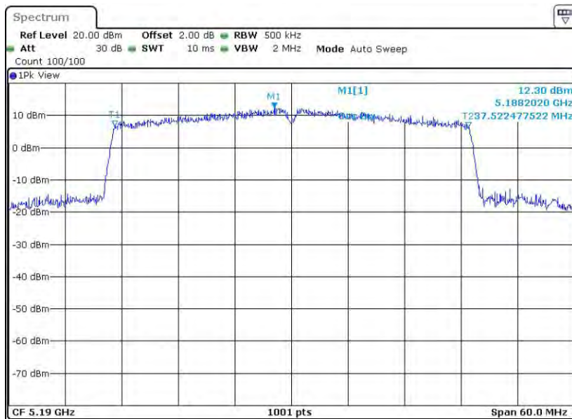
11AX40SISO_Ant2_5190
