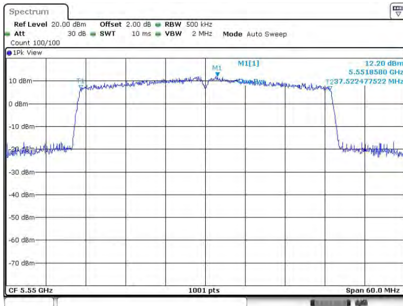
11AX40SISO_Ant8_5550
