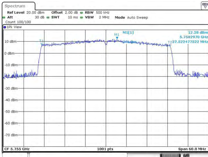
11AX40SISO_Ant8_5755
