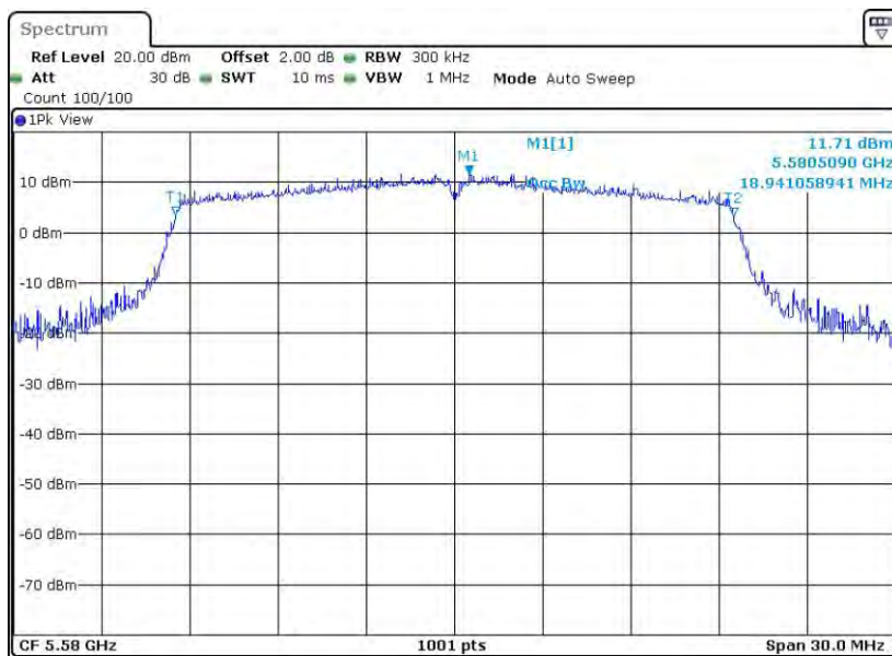
11AX20SISO_Ant2_5580
