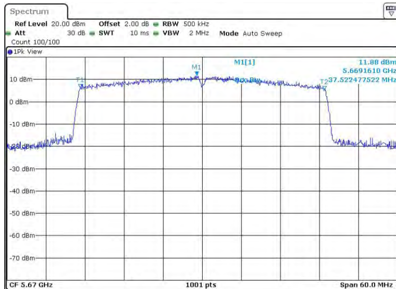
11AX40SISO_Ant8_5670
