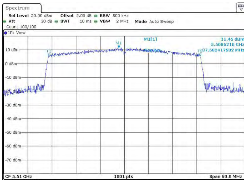
11AX40SISO_Ant2_5510
