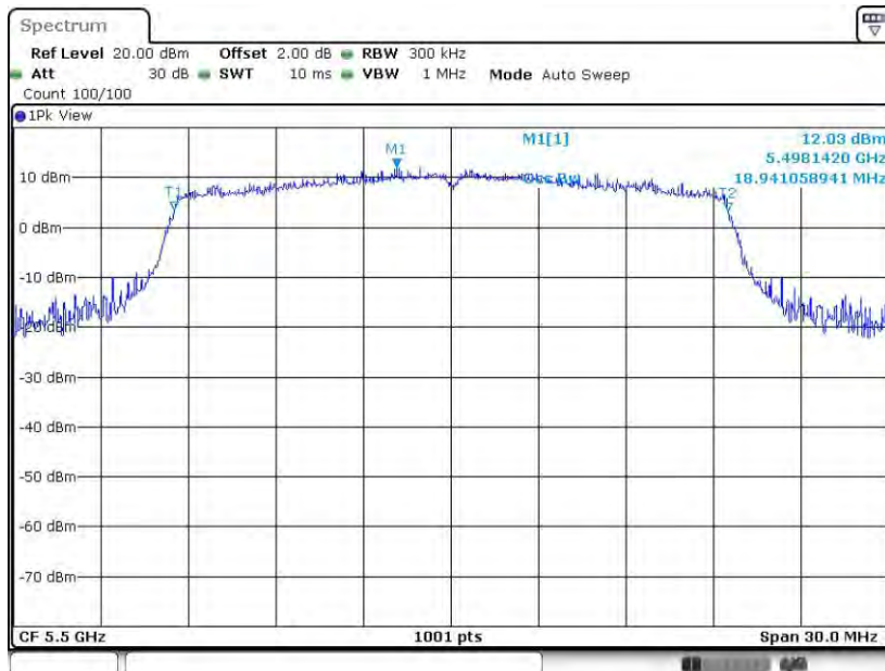
11AX20SISO_Ant8_5500
