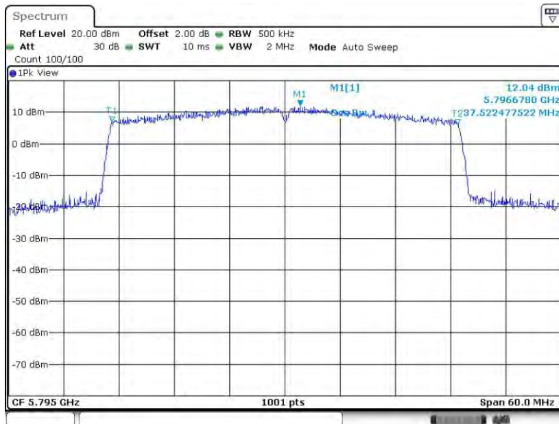
11AX40SISO_Ant8_5795
