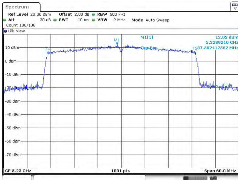
11AX40SISO_Ant8_5230
