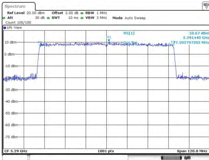
11AX80SISO_Ant2_5290
