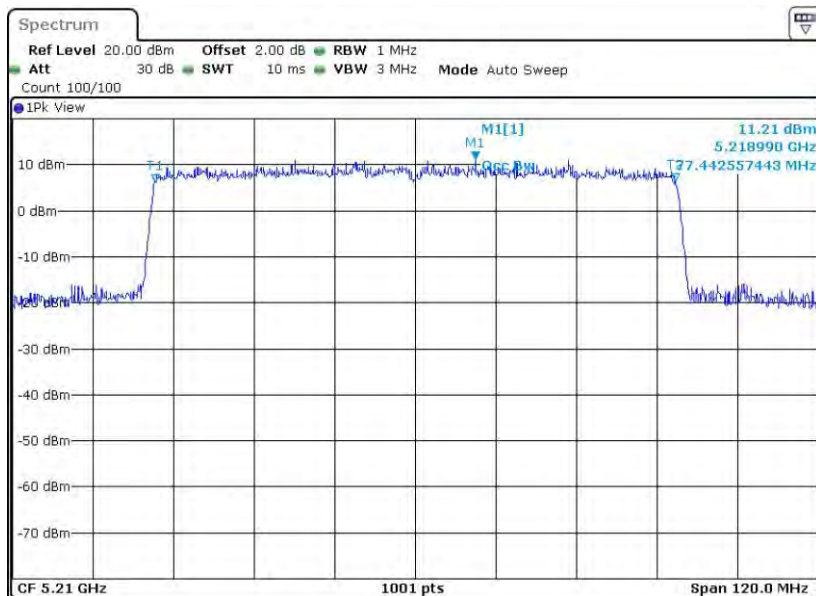
11AX80SISO_Ant2_5210
