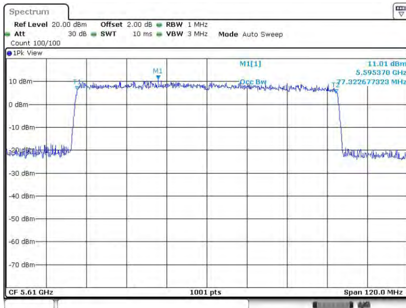
11AX80SISO_Ant8_5610
