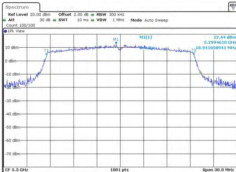
11AX20SISO_Ant2_5300
