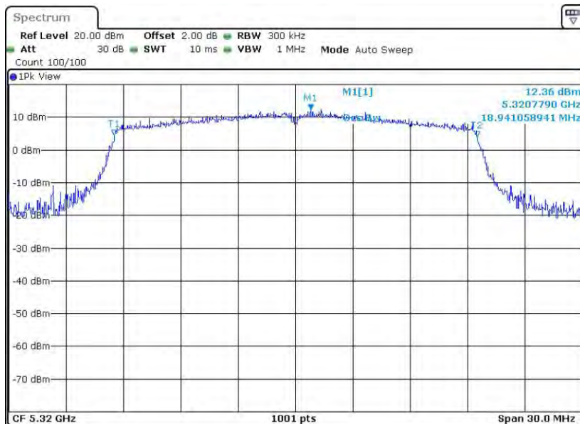
11AX20SISO_Ant2_5320
