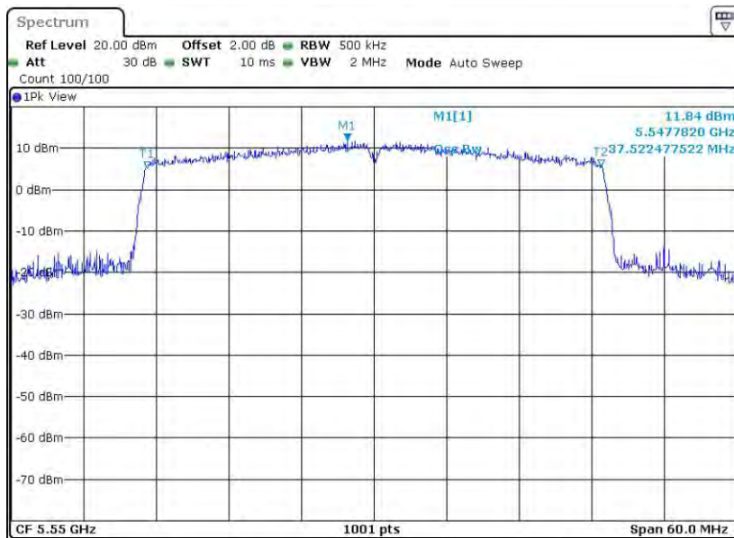
11AX40SISO_Ant2_5550
