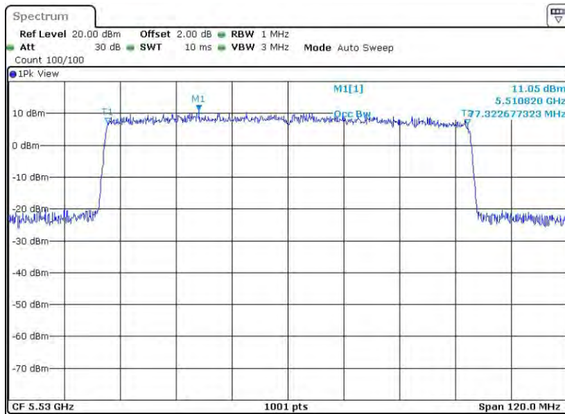
11AX80SISO_Ant8_5530
