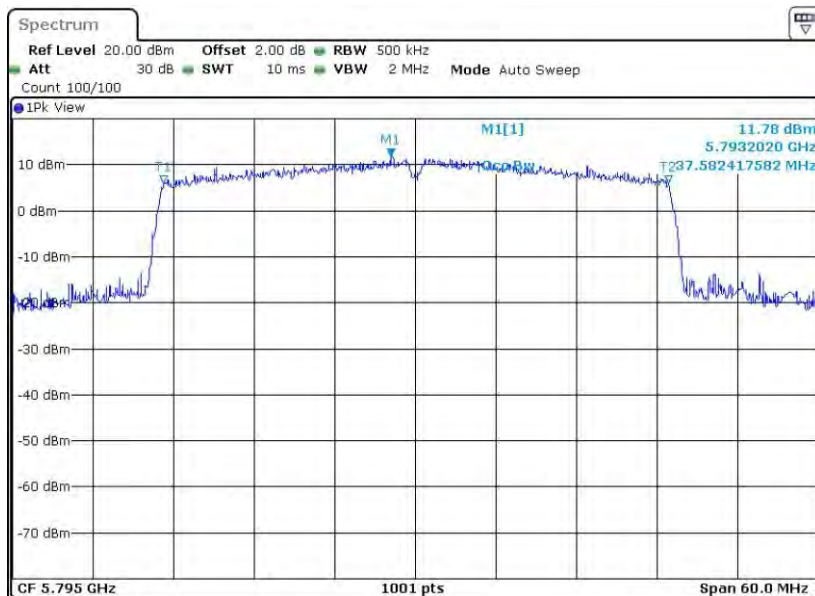
11AX40SISO_Ant2_5795
