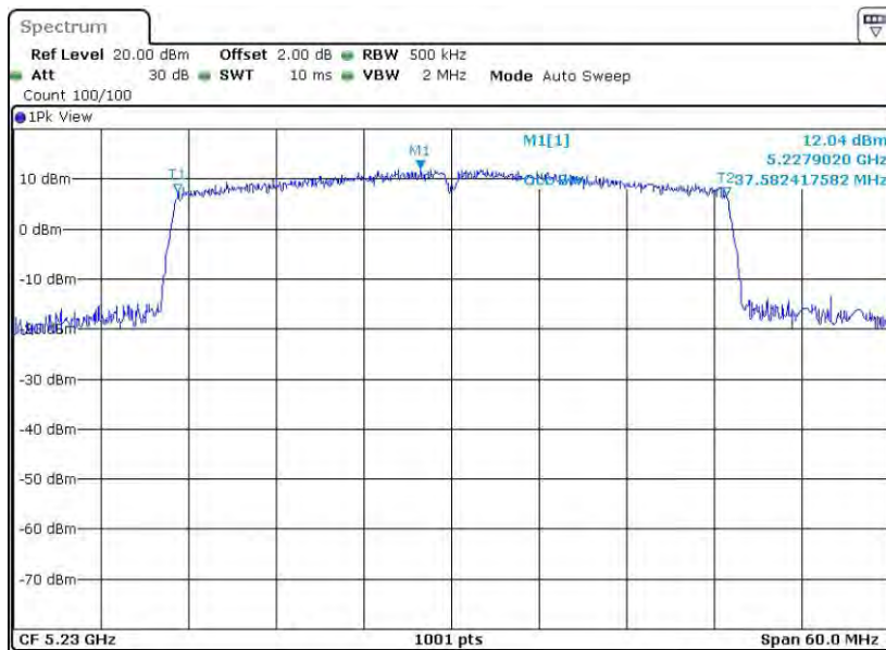
11AX40SISO_Ant2_5230
