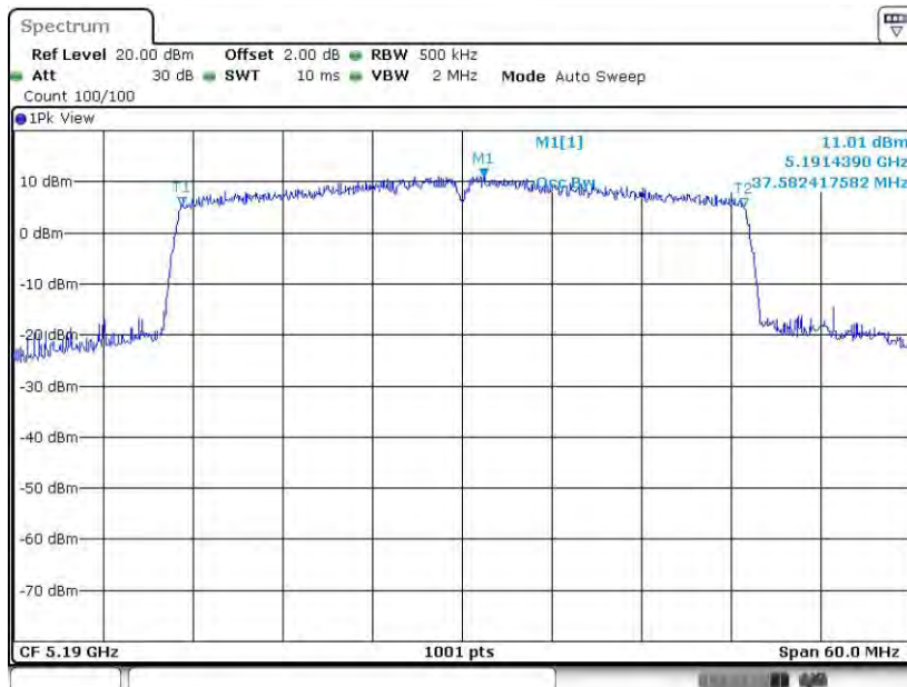
11AX40SISO_Ant8_5190
