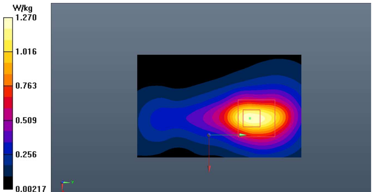
Fig.33 WLAN 5G
