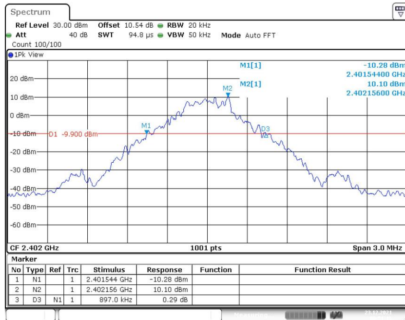
Fig. 67 20dB Bandwidth (GFSK, CH0)
