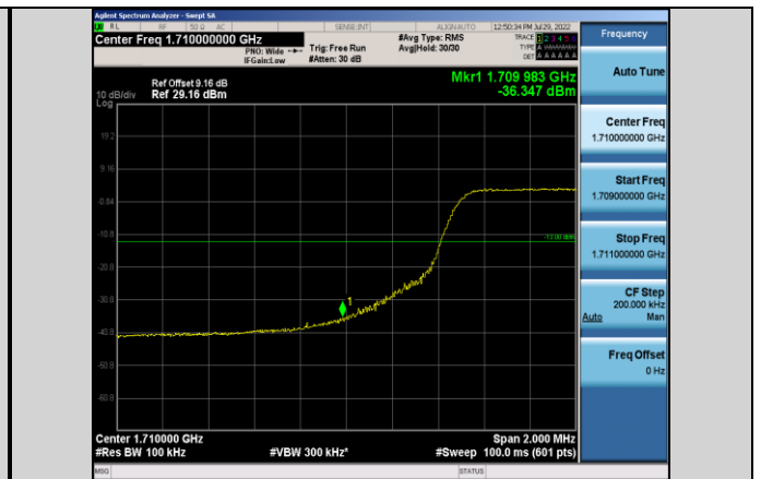
Band66-10MHz-QPSK-132022-50RB#0
