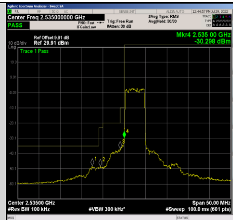
Band41-5MHz-QPSK-40065-25RB#0
