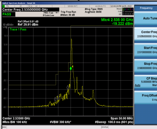
Band41-5MHz-QPSK-40065-1RB#0
