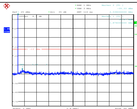
Band2-5MHz-QPSK-18900-1RB#0- Range2:1000~20000MHz
