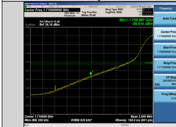
Band66-20MHz-QPSK-132072-1RB#0
