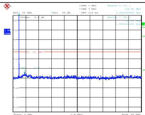
Band2-20MHz-16QAM-18900-1RB#0- Range2:1000~20000MHz
