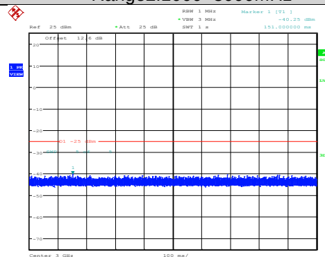
Band7-5MHz-QPSK-21100-1RB#0-Range2:1000~3000MHz
