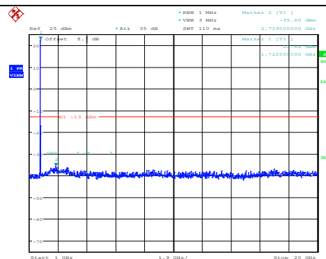
Band4-10MHz-QPSK-20175-1RB#0- Range2:1000~20000MHz
