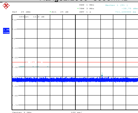
Band7-5MHz-QPSK-21425-1RB#0- Range2:1000~3000MHz
