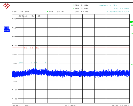
Band5-10MHz-QPSK-20525-1RB#0- Range2:1000~10000MHz
