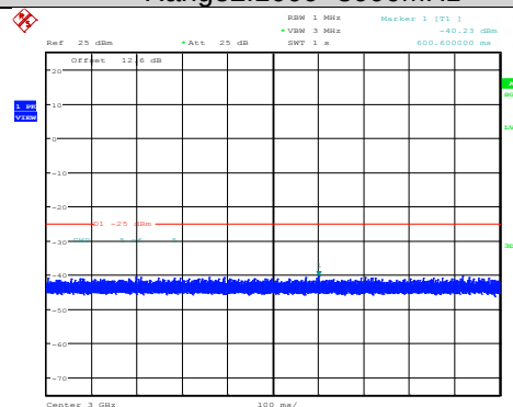
Band7-20MHz-QPSK-21350-1RB#0- Range2:1000~3000MHz
