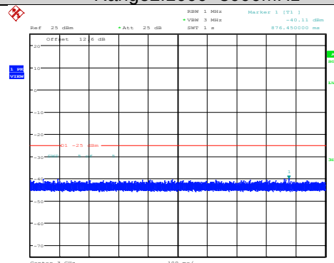
Band41-20MHz-QPSK-41140-1RB#0-Range2:1000~3000MHz
