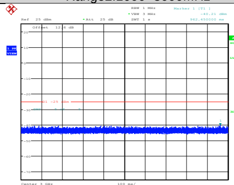
Band38-20MHz-QPSK-38150-1RB#0- Range2:1000~3000MHz
