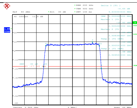
Band7-10MHz-QPSK-20800-50RB#0
