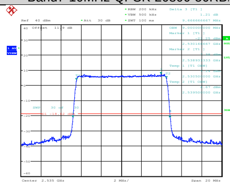
Band7-10MHz-QPSK-20800-50RB#0
