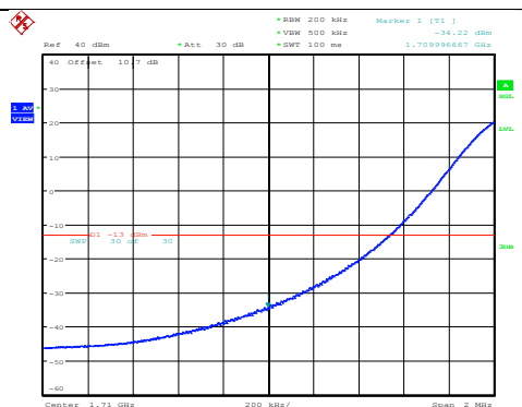
Band4-20MHz-QPSK-20050-1RB#0
