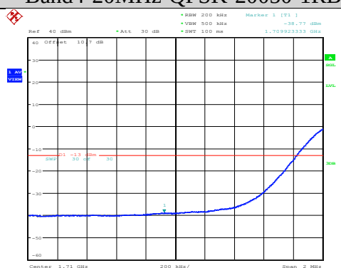
Band4-20MHz-QPSK-20050-1RB#0
