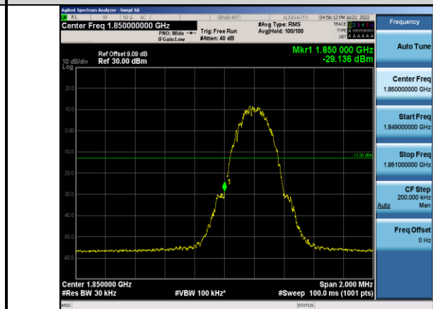
EGPRS1900-512-2
