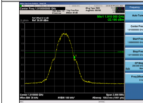
GSM1900-810-0
