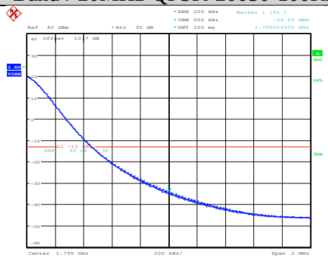
Band4-20MHz-QPSK-20050-100RB#0
