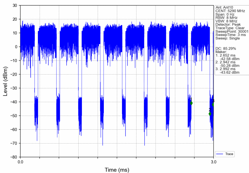
802.11ax(HEW80) MCH 5290MHz RU996 Left Ant10 NTN
