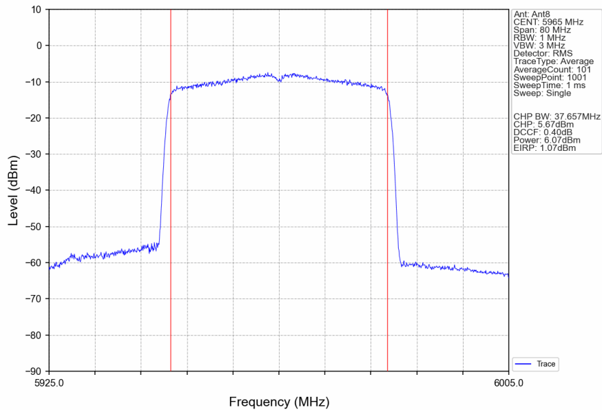
802.11ax(HEW40)_LCH_5965MHz_RU484_Left_Ant8_NTNV
