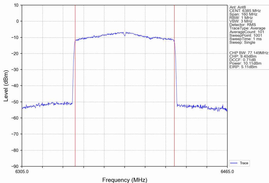
802.11ax(HEW80)_HCH_6385MHz_RU996_Left_Ant8_NTNV
