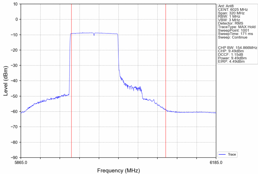
802.11ax(HEW160)_LCH_6025MHz_RU996_Left_Ant8_NTNV
