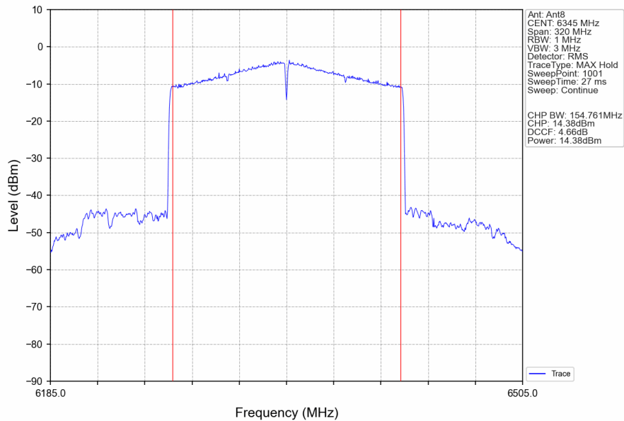
802.11ax(HEW160)_HCH_6345MHz_2xRU996_Left_Ant8_NTNV
