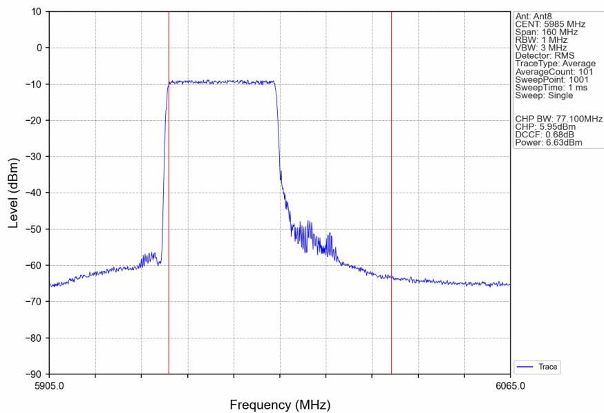
802.11ax(HEW80)_LCH_5985MHz_RU484_Left_Ant8_NTNV
