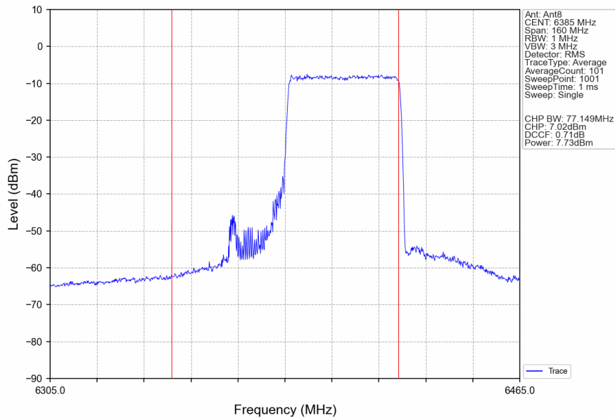
802.11ax(HEW80)_HCH_6385MHz_RU484_Right_Ant8_NTNV
