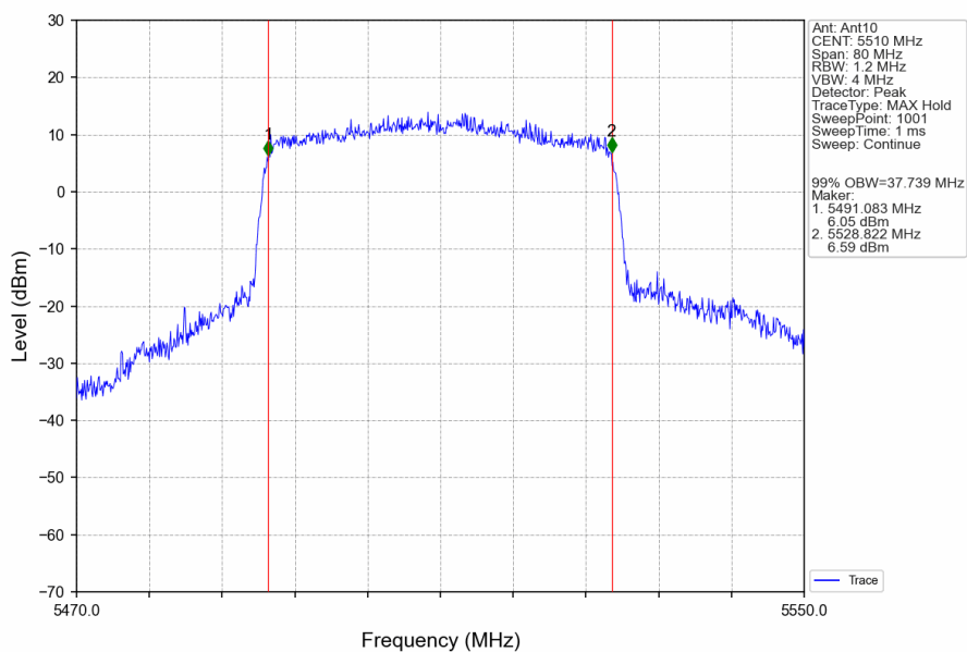
802.11be(EHT40) LCH 5510MHz RU484 Left Ant10 NTN
