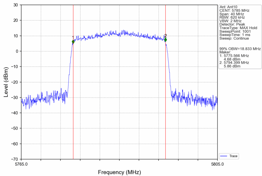
802.11be(EHT20) MCH 5785MHz RU242 Left Ant10 NTNV
