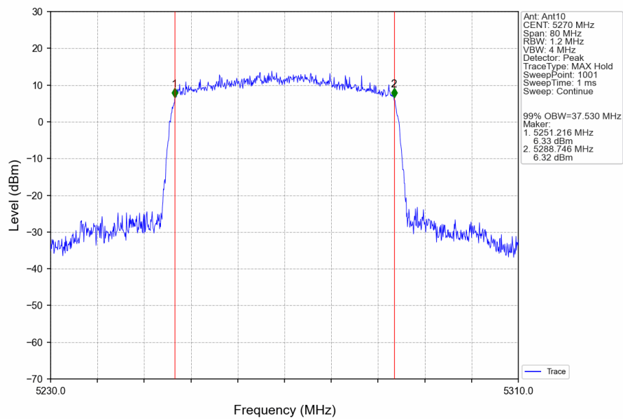
802.11be(EHT40) LCH 5270MHz RU484 Left Ant10 NTN
