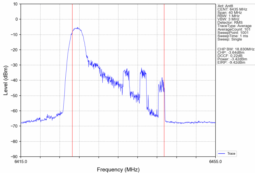
802.11ax(HEW20)_LCH_6435MHz_RU26_Left_Ant8_NTNV
