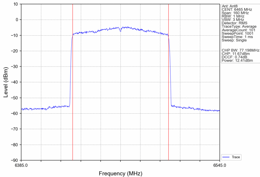
802.11ax(HEW80)_LCH_6465MHz_RU996_Left_Ant8_NTNV
