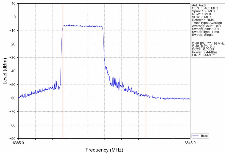
802.11ax(HEW80)_LCH_6465MHz_RU484_Left_Ant8_NTNV
