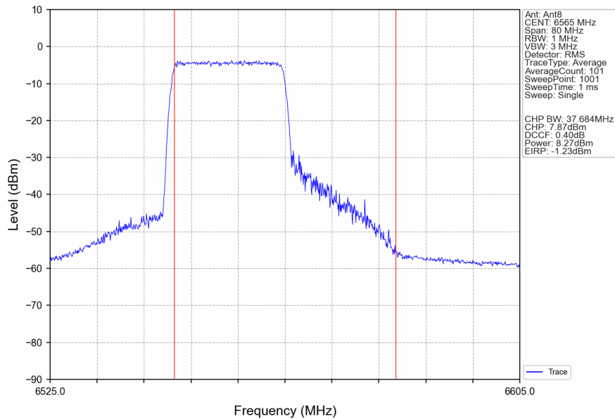
802.11ax(HEW40)_LCH_6565MHz_RU242_Left_Ant8_NTNV
