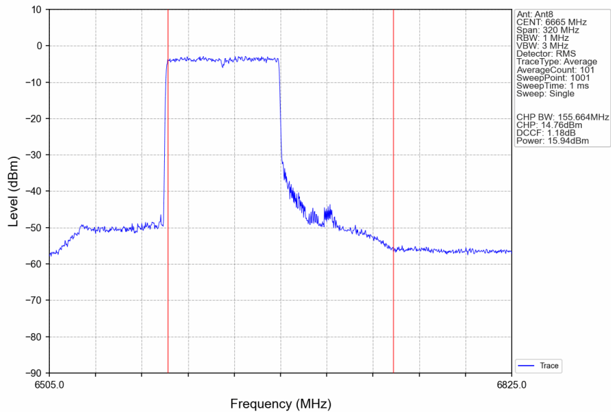
802.11ax(HEW160)_MCH_6665MHz_RU996_Left_Ant8_NTNV
