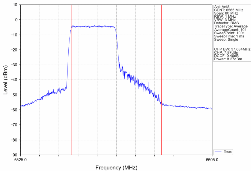
802.11ax(HEW40)_LCH_6565MHz_RU242_Left_Ant8_NTNV
