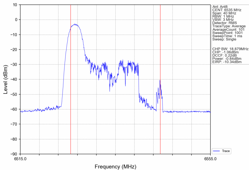
802.11ax(HEW20)_LCH_6535MHz_RU26_Left_Ant8_NTNV
