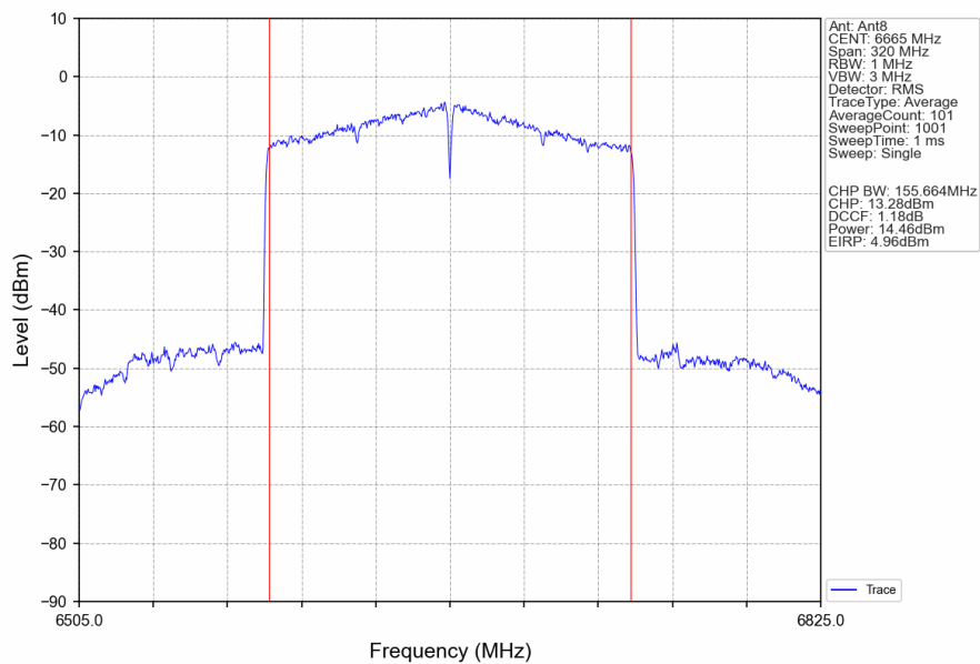
802.11ax(HEW160)_MCH_6665MHz_2xRU996_Left_Ant8_NTNV
