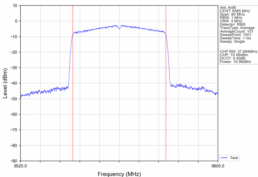
802.11ax(HEW40)_LCH_6565MHz_RU484_Left_Ant8_NTNV
