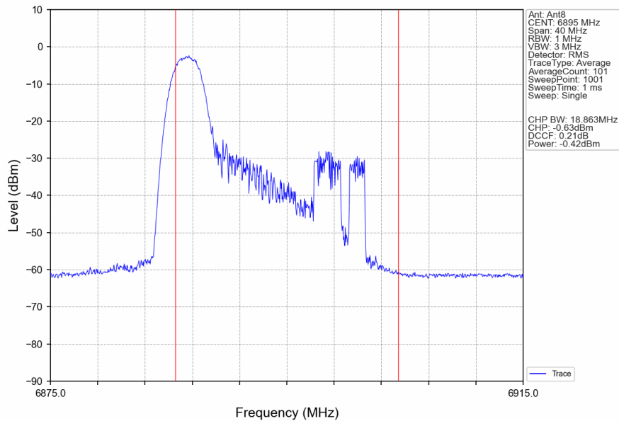
802.11ax(HEW20)_LCH_6895MHz_RU26_Left_Ant8_NTNV
