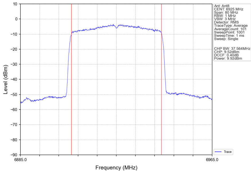
802.11ax(HEW40)_LCH_6925MHz_RU484_Left_Ant8_NTNV
