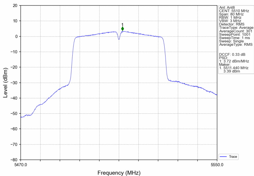
802.11ac(VHT40) LCH 5510MHz Ant8 NTN
