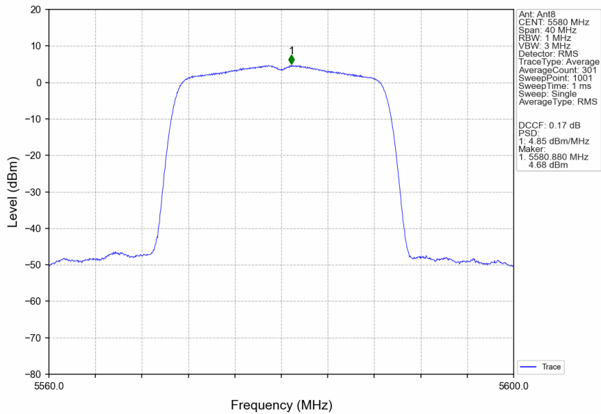
802.11ac(VHT20) MCH 5580MHz Ant8 NTN
