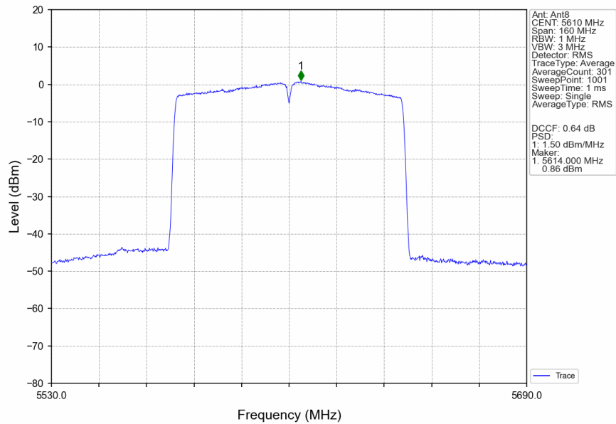
802.11ac(VHT80) HCH 5610MHz Ant8 NTN
