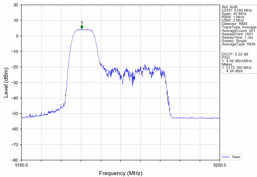
802.11ax(HEW20) LCH 5180MHz RU52 Left Ant8 NTN
