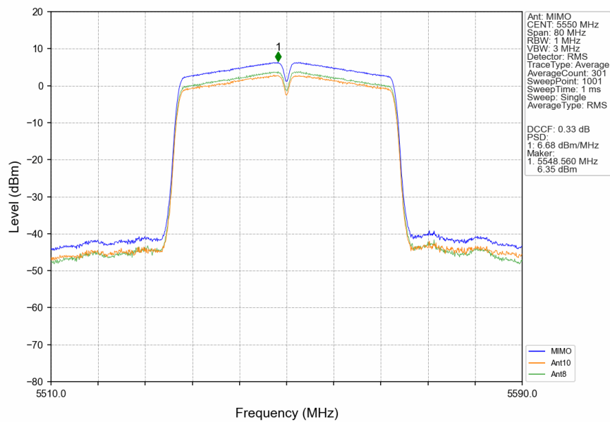
802.11ac(VHT40) MCH 5550MHz MIMO NTN
