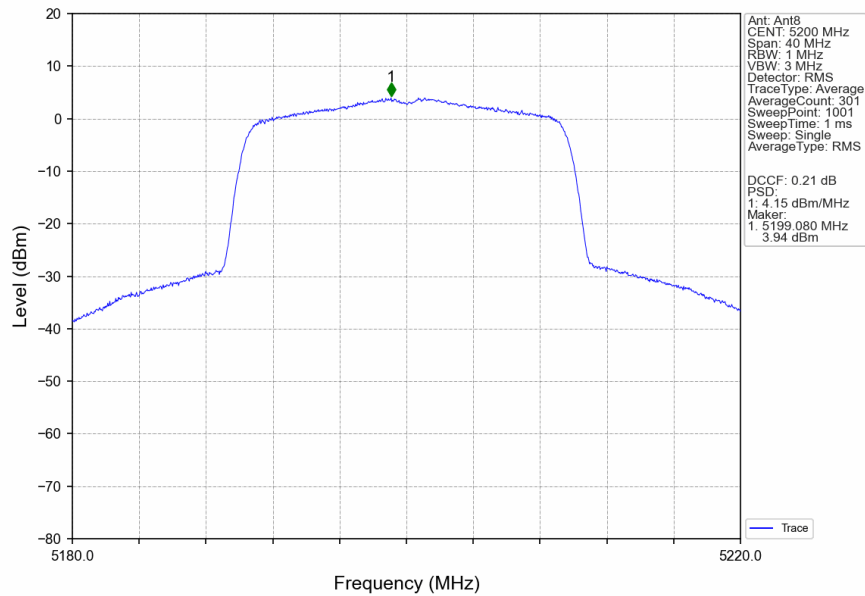
802.11ax(HEW20) MCH 5200MHz RU242 Left Ant8 NTN
