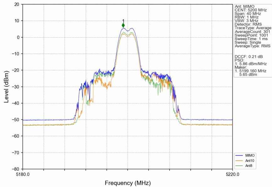
802.11ax(HEW20) MCH 5200MHz RU26 Mid MIMO NTN
