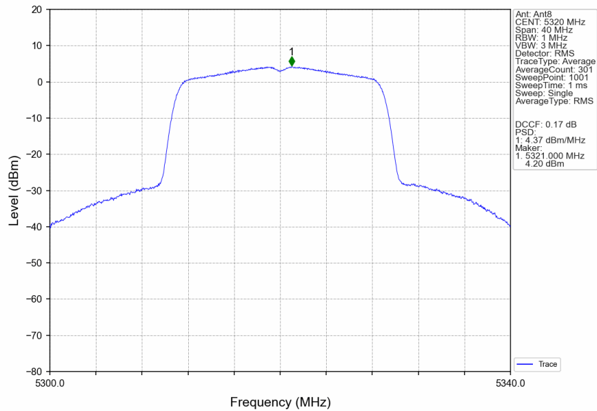
802.11ac(VHT20) HCH 5320MHz Ant8 NTN
