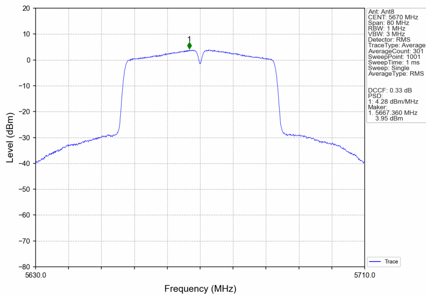
802.11ac(VHT40) HCH 5670MHz Ant8 NTN
