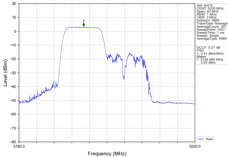
802.11ax(HEW20) MCH 5200MHz RU106 Left Ant10 NTN
