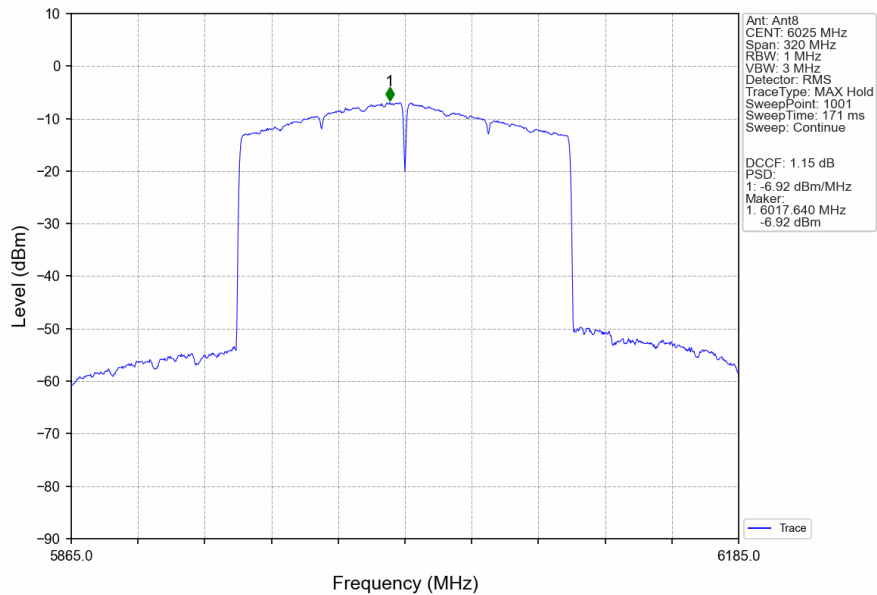
802.11ax(HEW160)_LCH_6025MHz_2xRU996_Left_Ant8_NTNV
