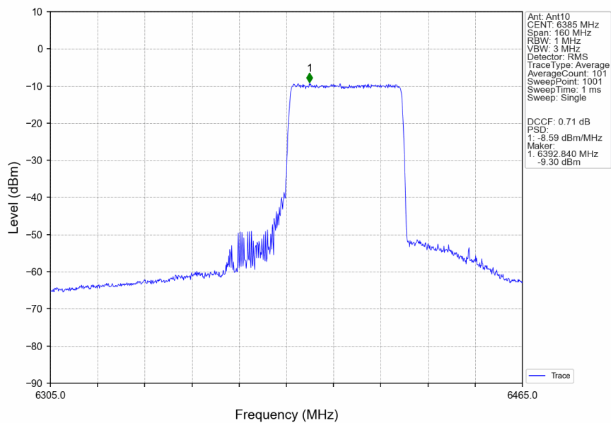
802.11ax(HEW80)_HCH_6385MHz_RU484_Right_Ant10_NTNV
