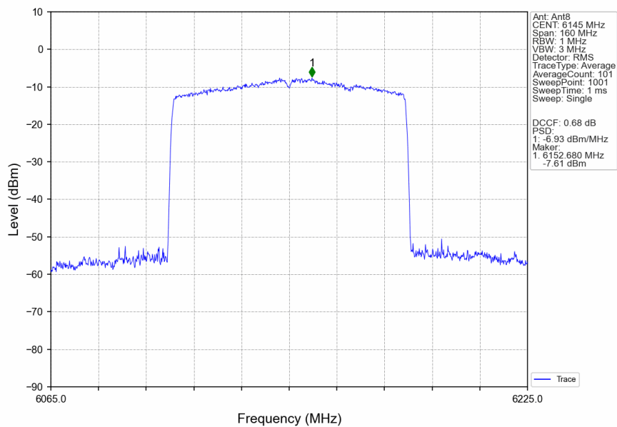
802.11ax(HEW80)_MCH_6145MHz_RU996_Left_Ant8_NTNV
