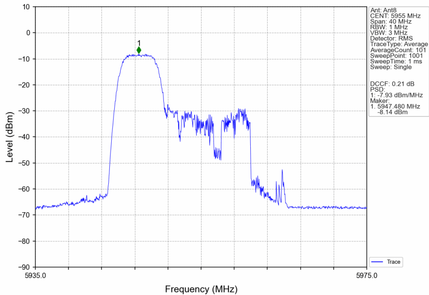
802.11ax(HEW20)_LCH_5955MHz_RU52_Left_Ant8_NTNV
