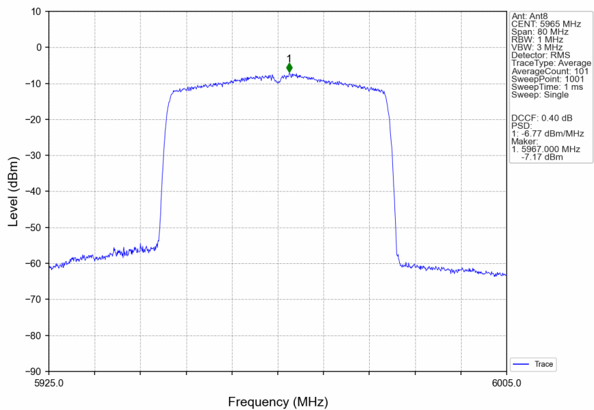
802.11ax(HEW40)_LCH_5965MHz_RU484_Left_Ant8_NTNV
