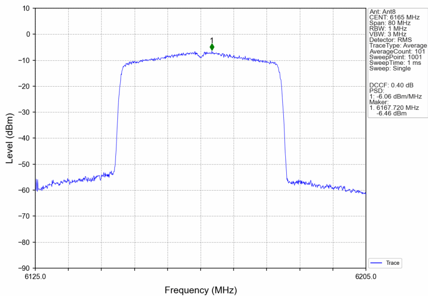
802.11ax(HEW40)_MCH_6165MHz_RU484_Left_Ant8_NTNV
