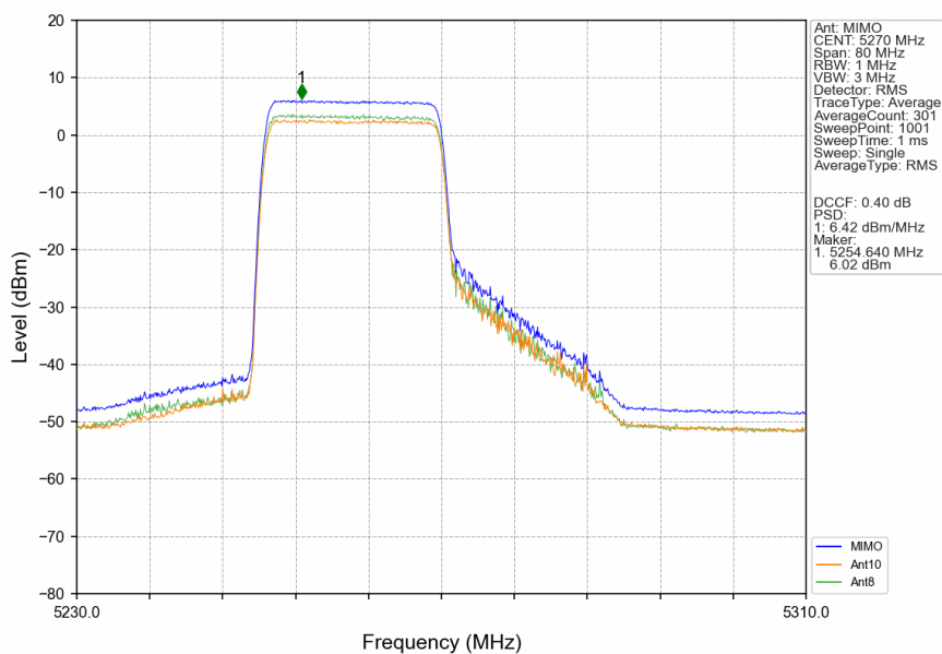
802.11ax(HEW40) LCH 5270MHz RU242 Left MIMO NTN
