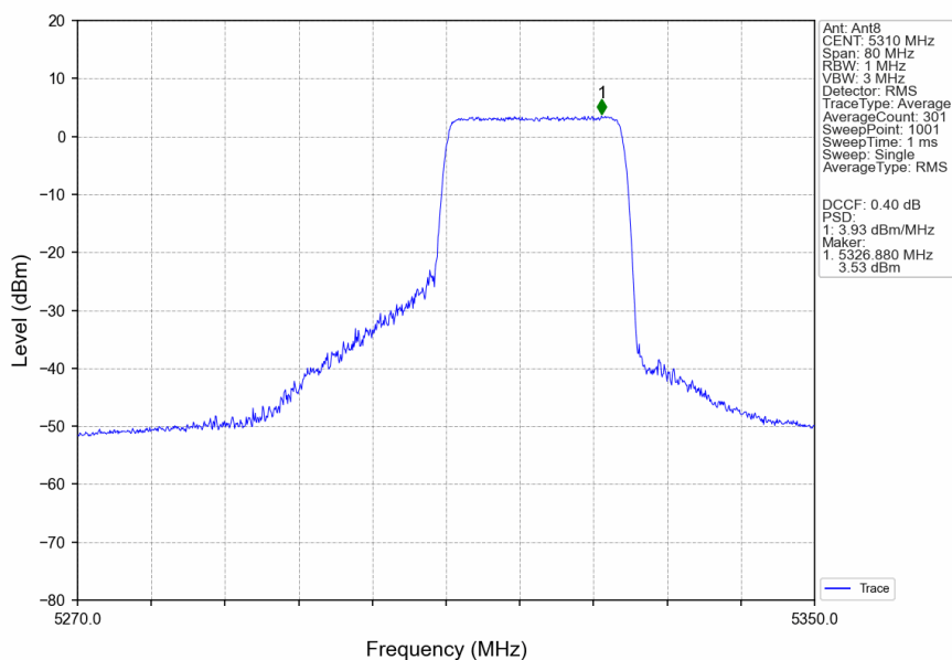
802.11ax(HEW40) HCH 5310MHz RU242 Right MIMO NTN
