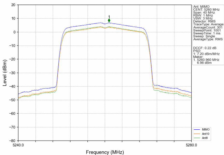
802.11be(EHT20) LCH 5260MHz RU242 Left MIMO NTN
