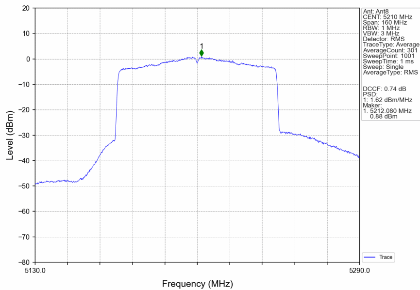
802.11ax(HEW80) MCH 5210MHz RU996 Left Ant8 NTN
