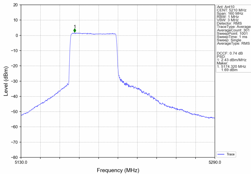
802.11ax(HEW80) MCH 5210MHz RU484 Left Ant10 NTN
