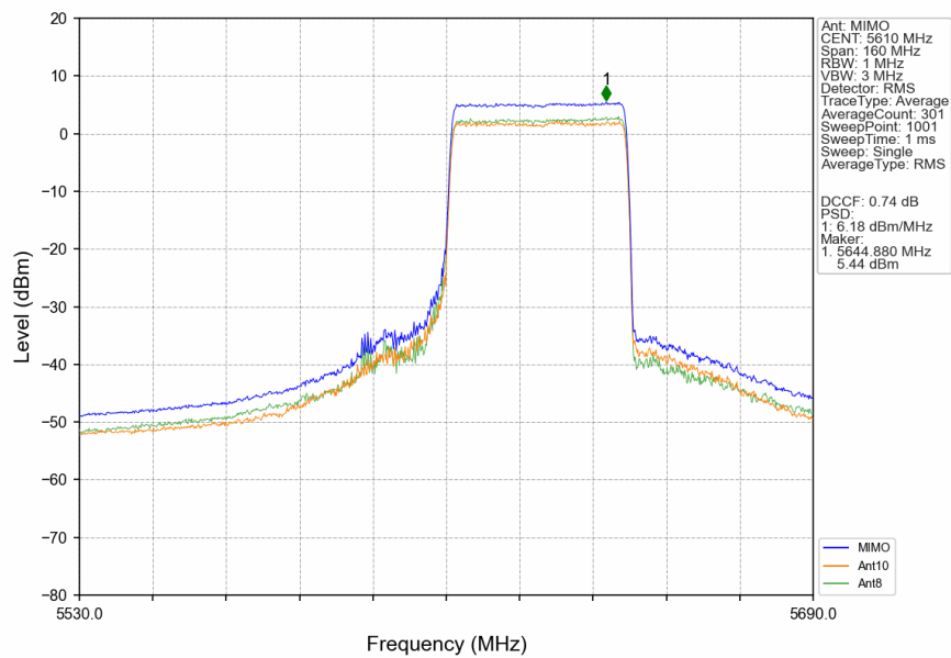
802.11ax(HEW80) HCH 5610MHz RU484 Right MIMO NTN
