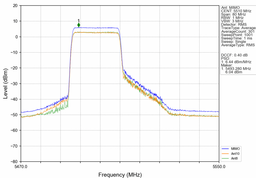
802.11ax(HEW40) LCH 5510MHz RU242 Left MIMO NTN
