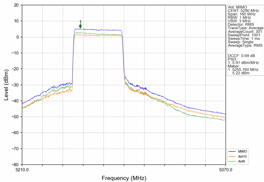
802.11ax(HEW80) MCH 5290MHz RU484 Left MIMO NTN
