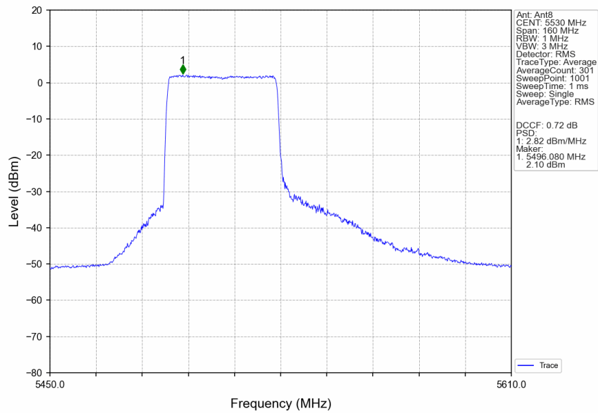
802.11ax(HEW80) LCH 5530MHz RU484 Left MIMO NTN
