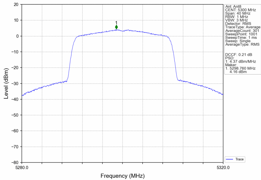
802.11be(EHT20) MCH 5300MHz RU242 Left MIMO NTN
