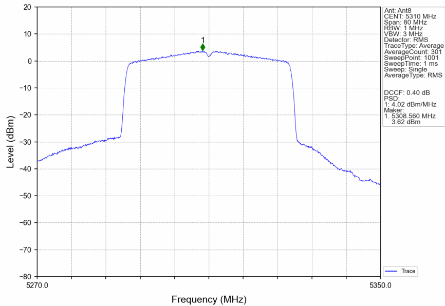
802.11ax(HEW40) HCH 5310MHz RU484 Left Ant8 NTN
