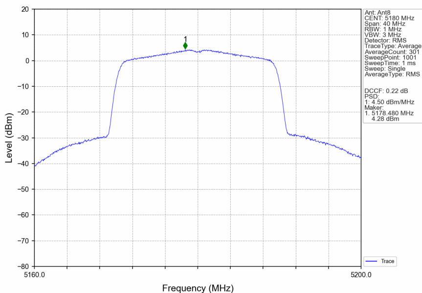
802.11be(EHT20) LCH 5180MHz RU242 Left MIMO NTN
