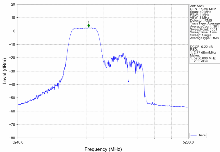
802.11be(EHT20) LCH 5260MHz 26+52 / Ant8 NTN
