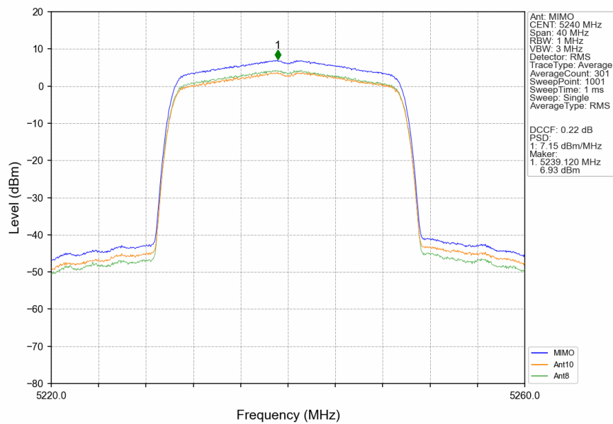
802.11be(EHT20) HCH 5240MHz RU242 Left MIMO NTN
