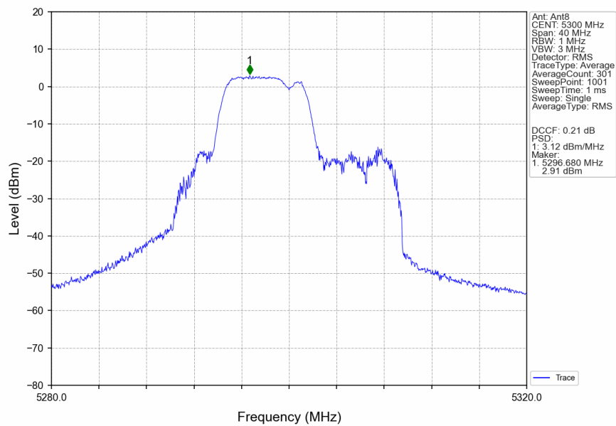
802.11be(EHT20) MCH 5300MHz 26+52 / Ant8 NTN
