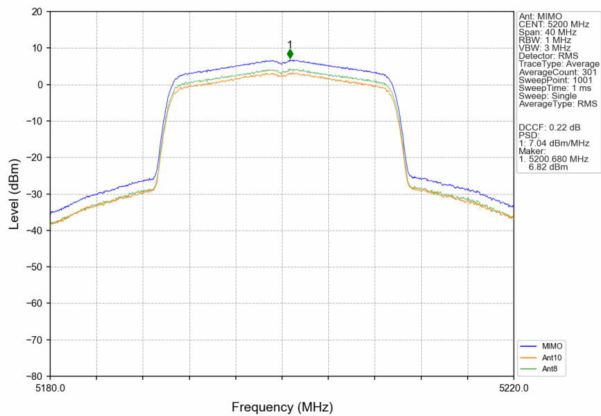
802.11be(EHT20) MCH 5200MHz RU242 Left MIMO NTN
