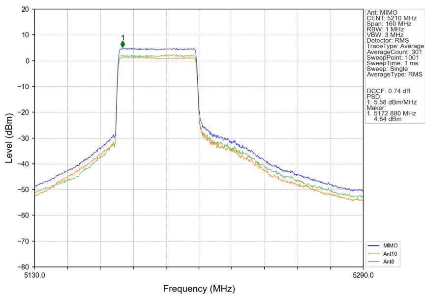
802.11ax(HEW80) MCH 5210MHz RU484 Left MIMO NTN
