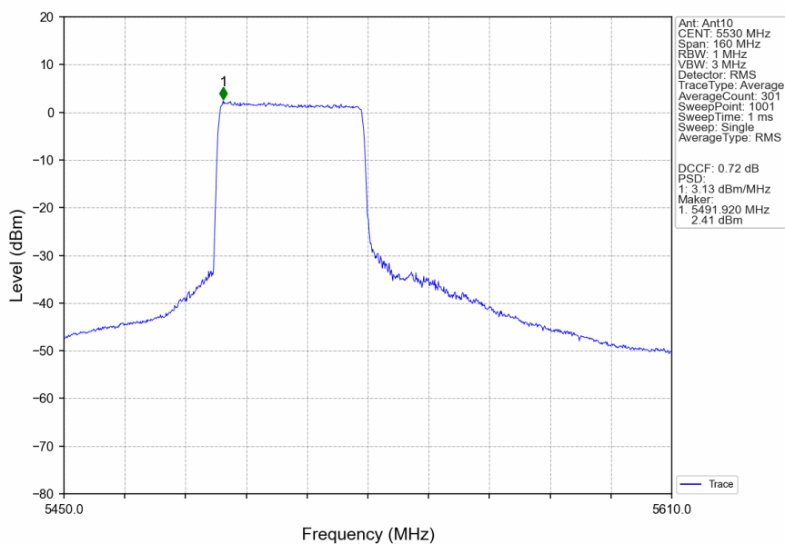
802.11ax(HEW80) LCH 5530MHz RU484 Left Ant10 NTN
