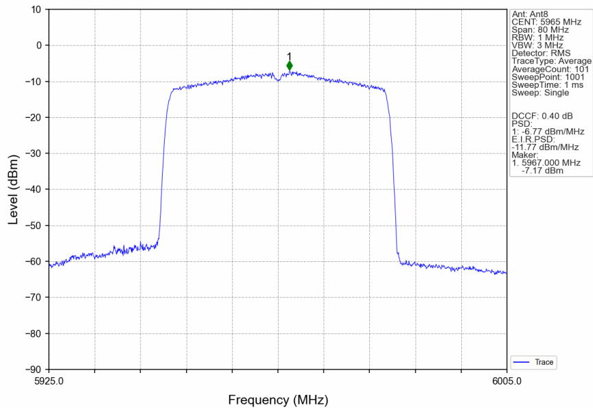
802.11ax(HEW40)_LCH_5965MHz_RU484_Left_Ant8_NTNV
