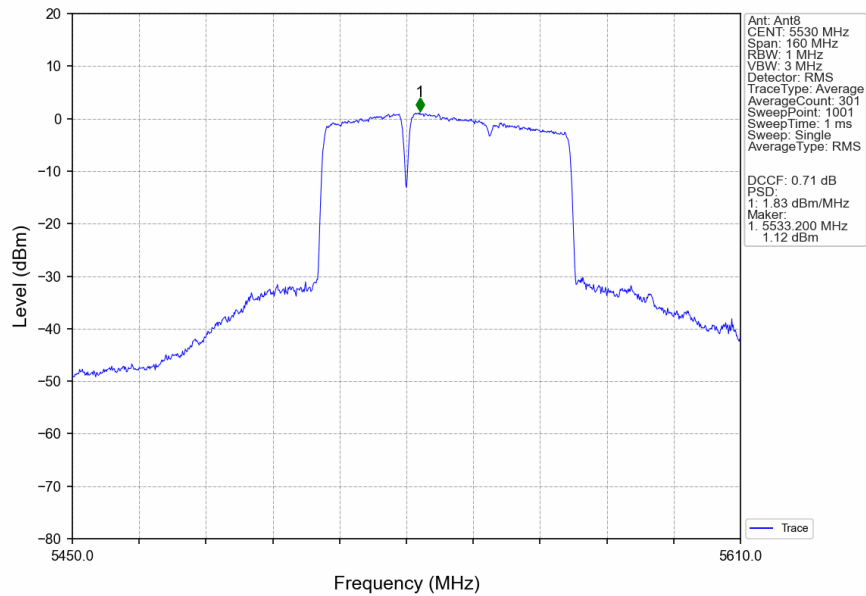
802.11be(EHT80) LCH 5530MHz 242+484 / Ant8 NTNV
