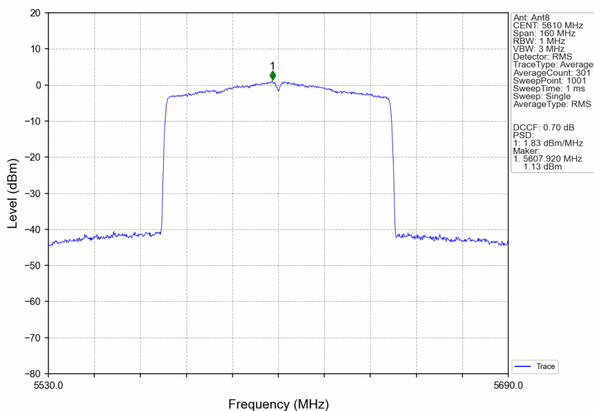
802.11be(EHT80) HCH 5610MHz RU996 Left MIMO NTN
