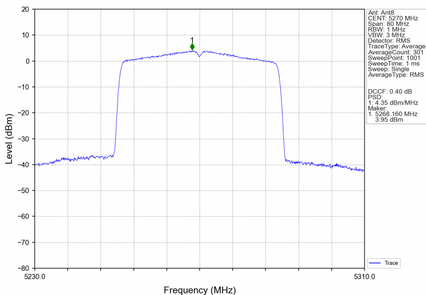
802.11be(EHT40) LCH 5270MHz RU484 Left MIMO NTN
