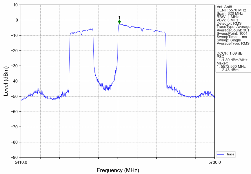
802.11be(EHT160) MCH 5570MHz 484+996 / Ant8 NTN
