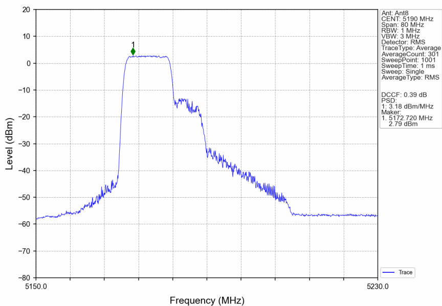
802.11be(EHT40) LCH 5190MHz 26+106 / Ant8 NTN
