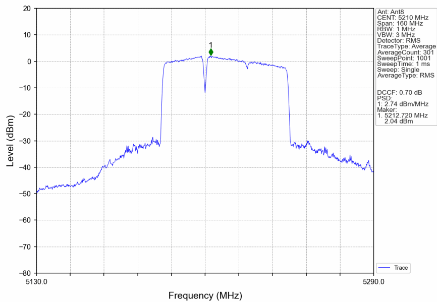
802.11be(EHT80) MCH 5210MHz 242+484 / Ant8 NTN
