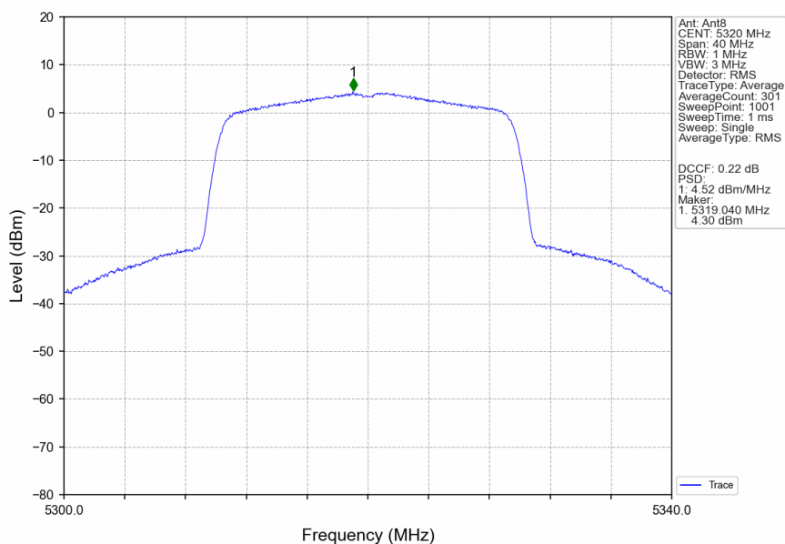
802.11be(EHT20) HCH 5320MHz RU242 Left MIMO NTN
