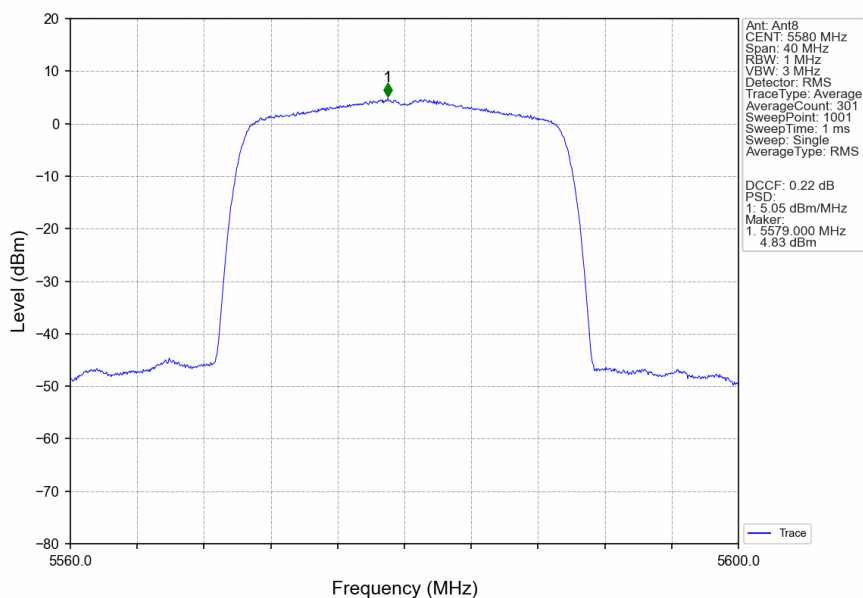
802.11be(EHT20) MCH 5580MHz RU242 Left MIMO NTN
