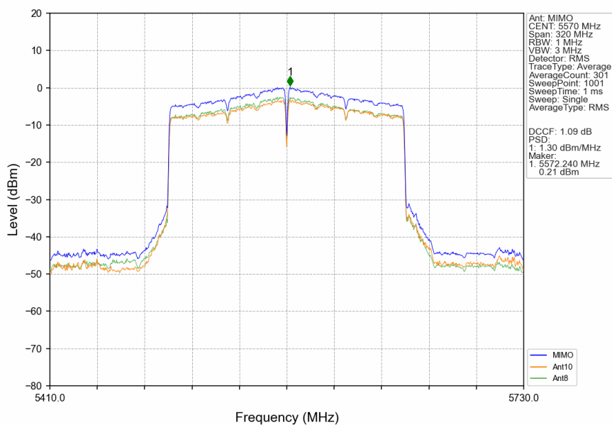
802.11be(EHT160) MCH 5570MHz 2xRU996 Left MIMO NTN
