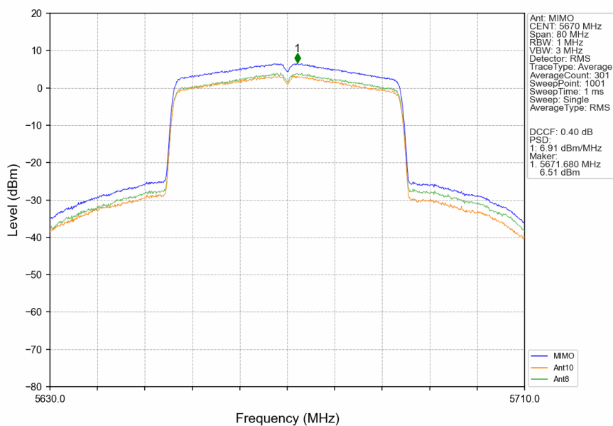
802.11be(EHT40) HCH 5670MHz RU484 Left MIMO NTN
