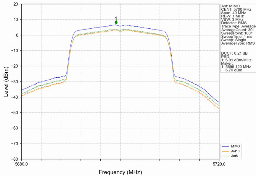
802.11be(EHT20) HCH 5700MHz RU242 Left MIMO NTN
