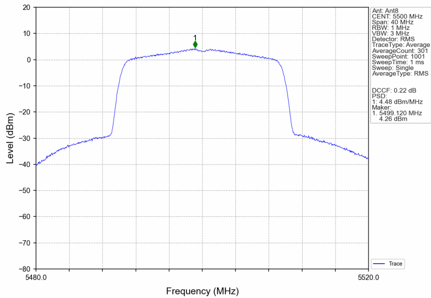
802.11be(EHT20) LCH 5500MHz RU242 Left MIMO NTN
