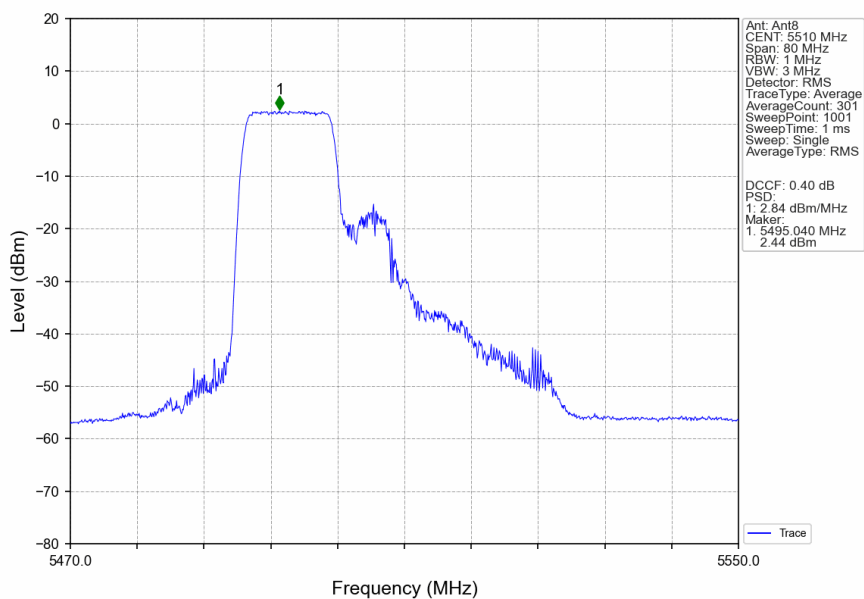
802.11be(EHT40) LCH 5510MHz 26+106 / Ant8 NTN
