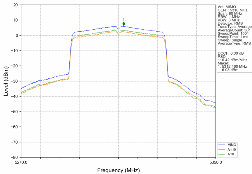
802.11be(EHT40) HCH 5310MHz RU484 Left MIMO NTN
