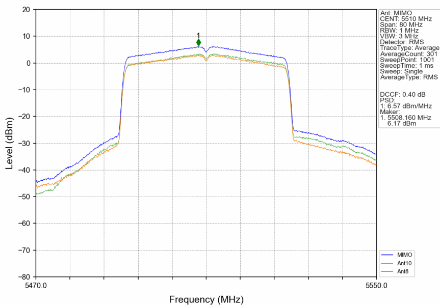
802.11be(EHT40) LCH 5510MHz RU484 Left MIMO NTN
