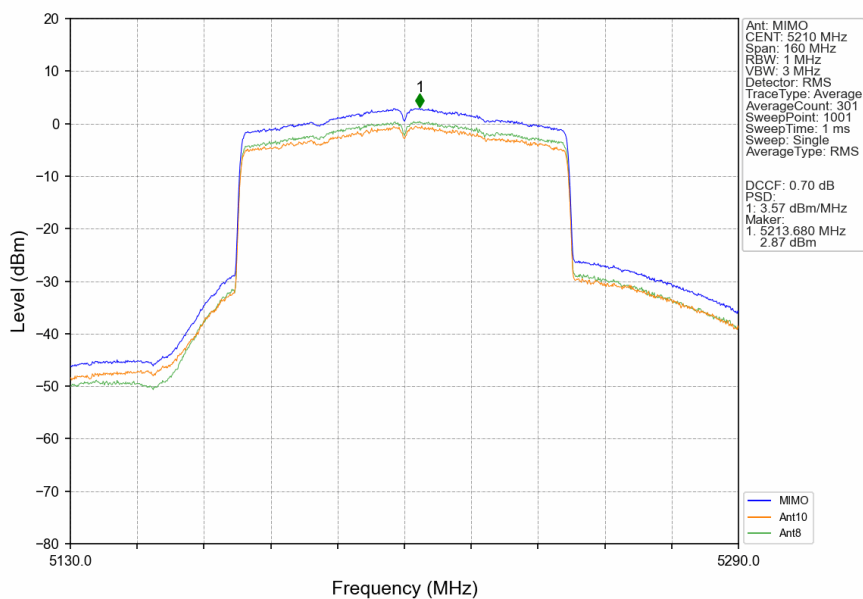
802.11be(EHT80) MCH 5210MHz RU996 Left MIMO NTN
