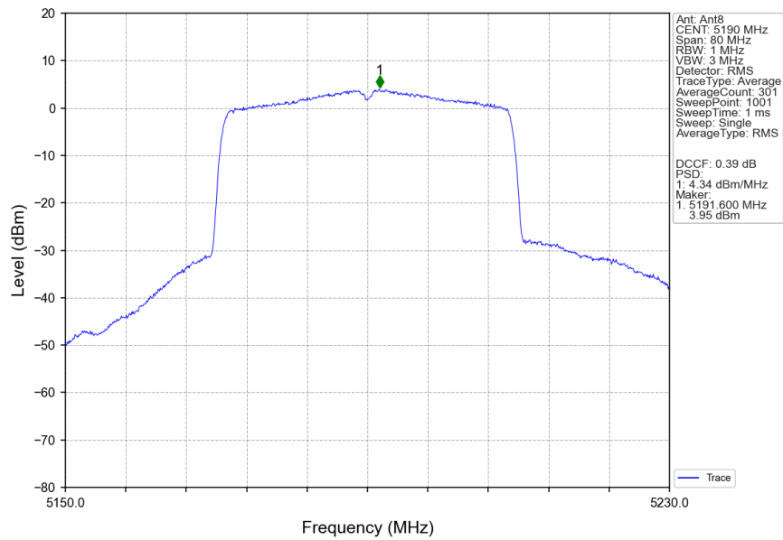
802.11be(EHT40) LCH 5190MHz RU484 Left MIMO NTN
