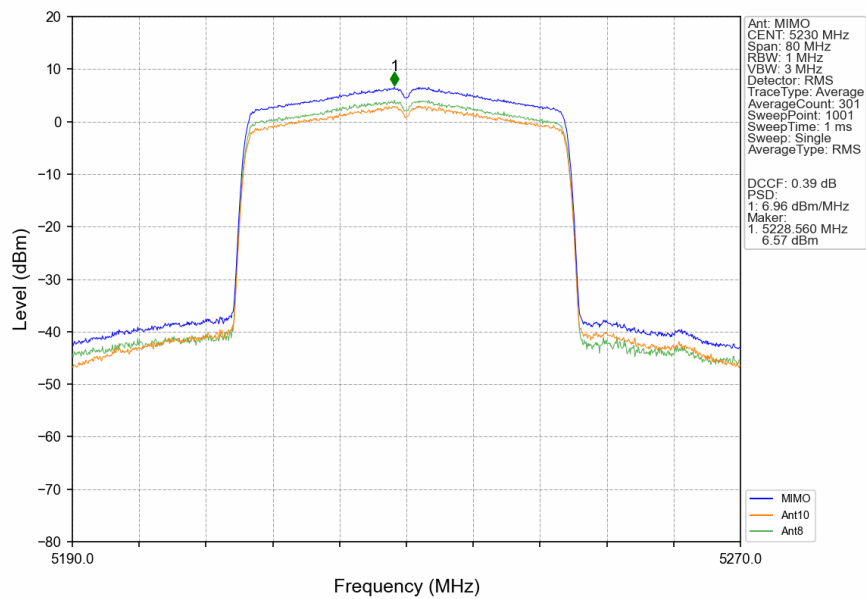
802.11be(EHT40) HCH 5230MHz RU484 Left MIMO NTN
