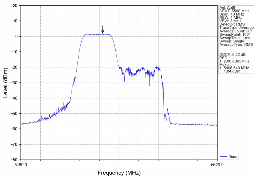
802.11be(EHT20) LCH 5500MHz 26+52 / Ant8 NTN
