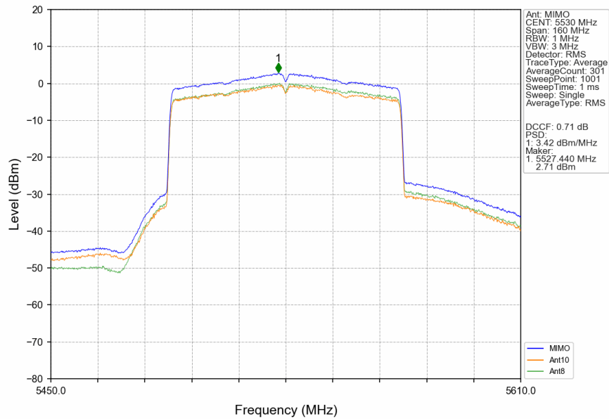
802.11be(EHT80) LCH 5530MHz RU996 Left MIMO NTN
