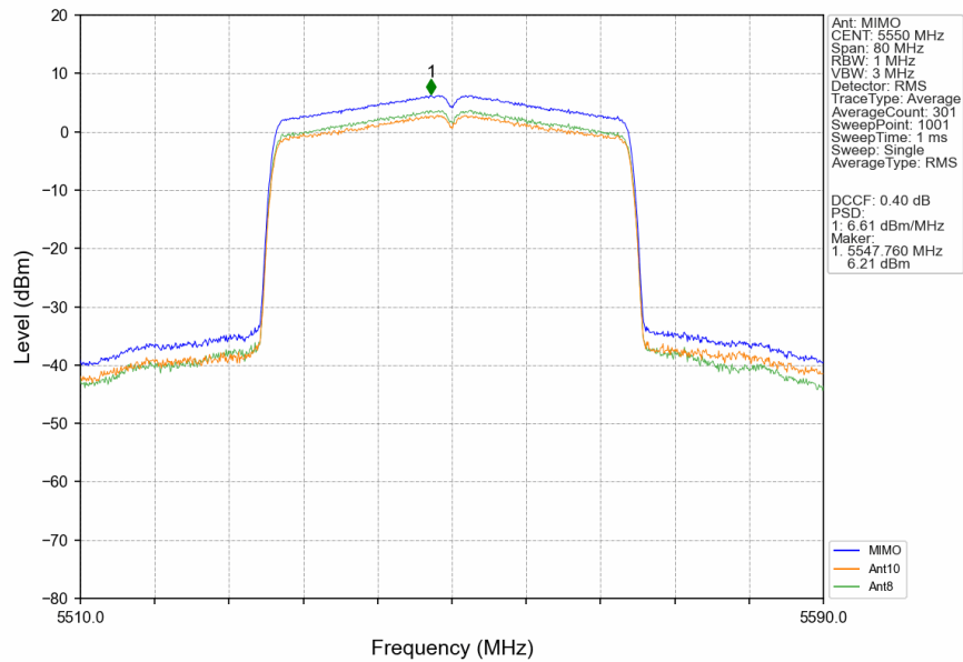
802.11be(EHT40) MCH 5550MHz RU484 Left MIMO NTN
