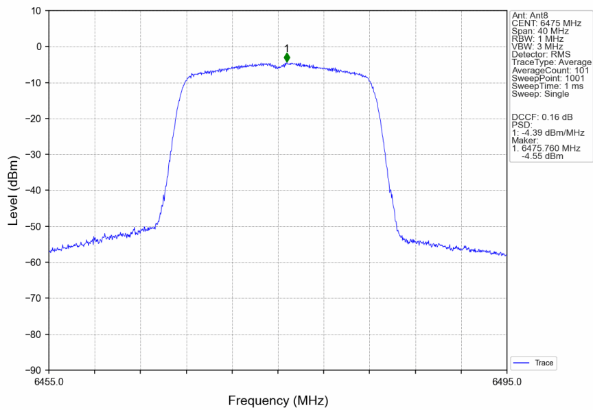
802.11a_MCH_6475MHz_MIMO_NTNV
