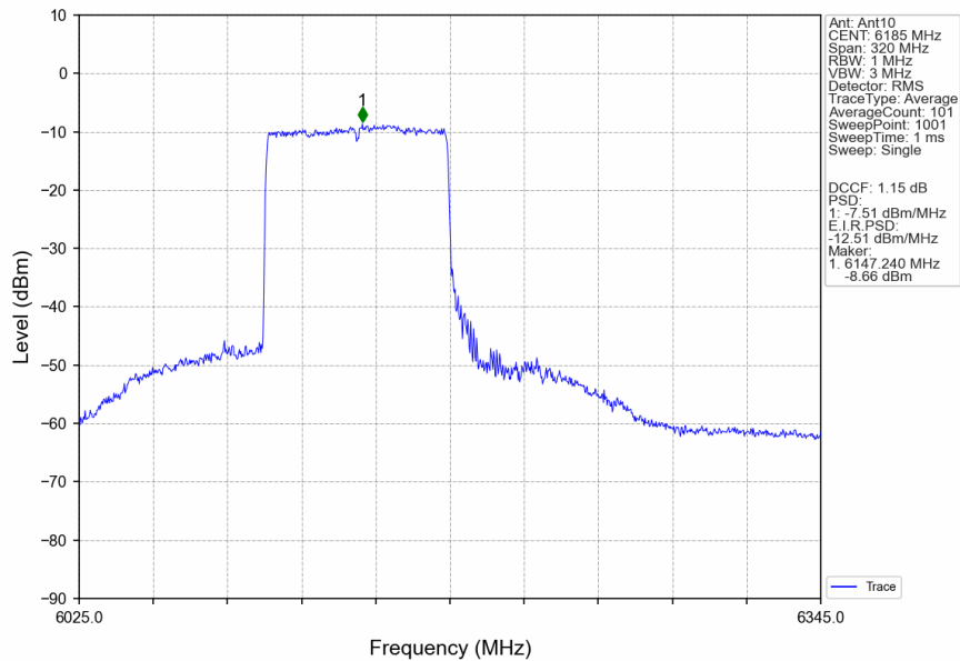
802.11ax(HEW160)_MCH_6185MHz_RU996_Left_Ant10_NTNV
