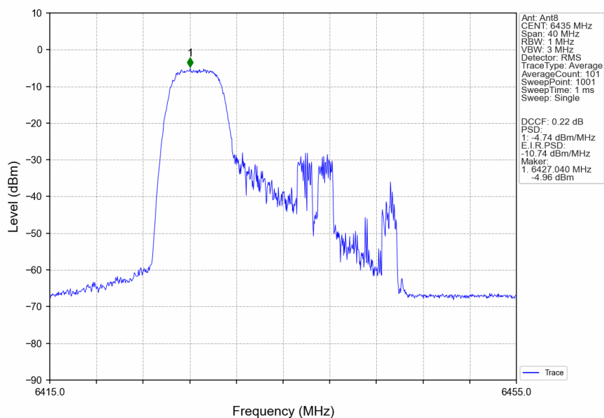
802.11ax(HEW20)_LCH_6435MHz_RU52_Left_Ant8_NTNV
