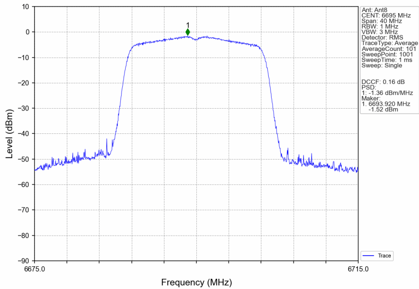
802.11a_MCH_6695MHz_MIMO_NTNV
