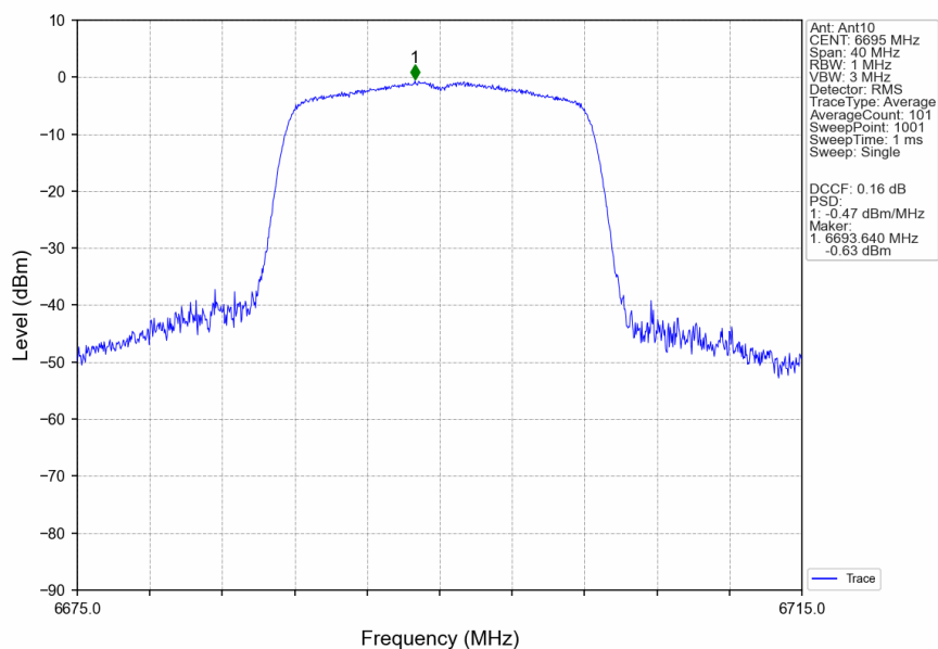
802.11a_MCH_6695MHz_Ant10_NTNV
