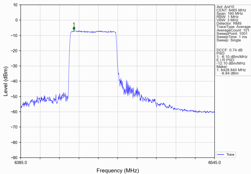
802.11ax(HEW80)_LCH_6465MHz_RU484_Left_Ant10_NTNV
