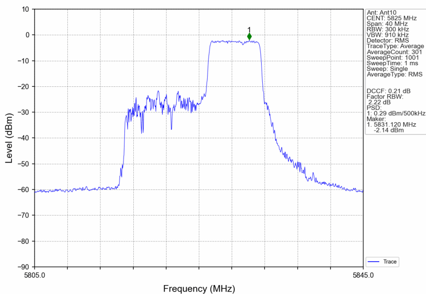
802.11be(EHT20) HCH 5825MHz 26+52 / Ant10 NTN
