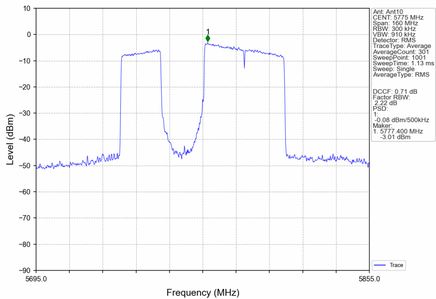
802.11be(EHT80) MCH 5775MHz 242+484 / Ant10 NTN
