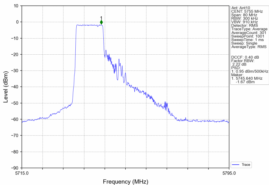
802.11be(EHT40) LCH 5755MHz 26+106 / Ant10 NTN
