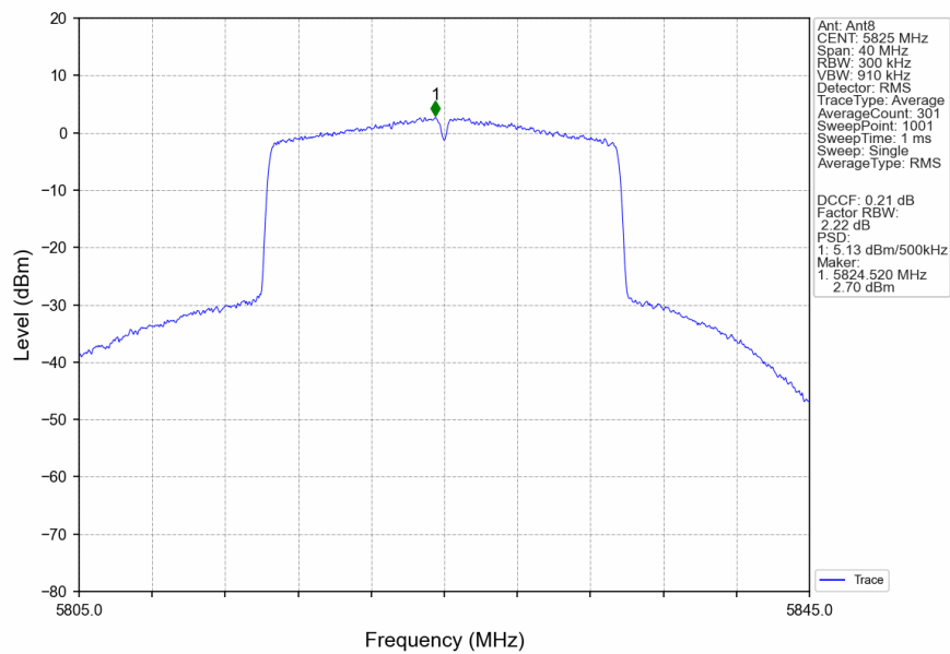
802.11be(EHT20) HCH 5825MHz RU242 Left Ant8 NTN
