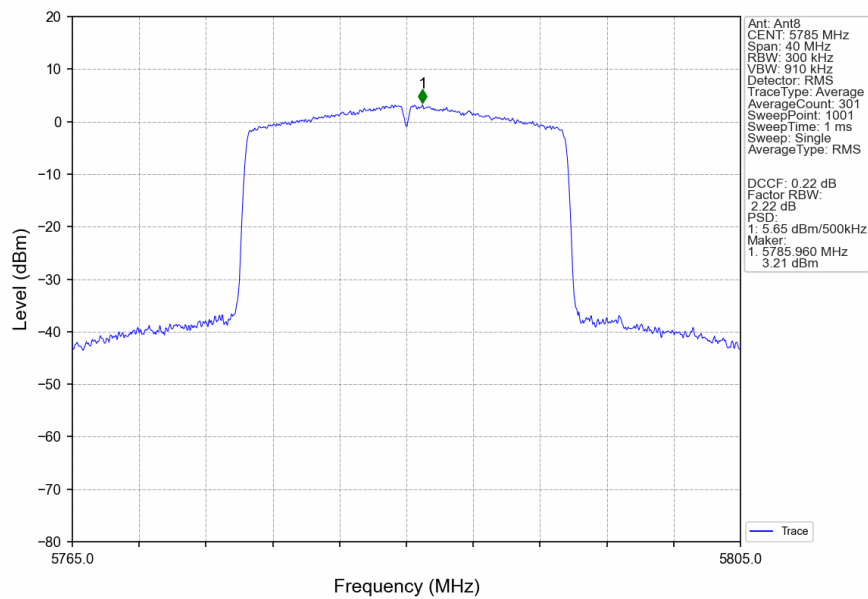
802.11be(EHT20) MCH 5785MHz RU242 Left Ant8 NTN
