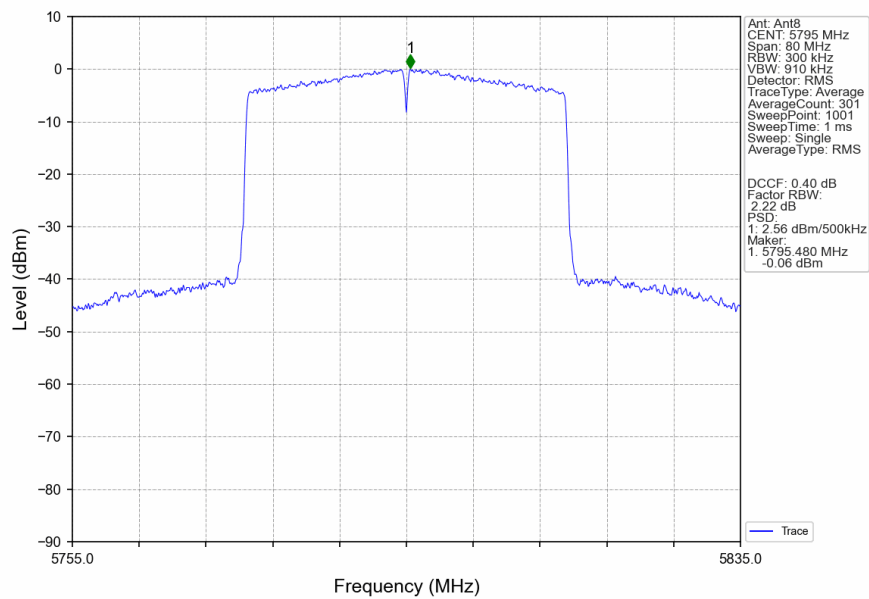
802.11be(EHT40) HCH 5795MHz RU484 Left Ant8 NTN
