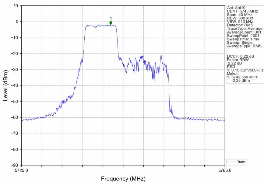
802.11be(EHT20) LCH 5745MHz 26+52 / Ant10 NTN
