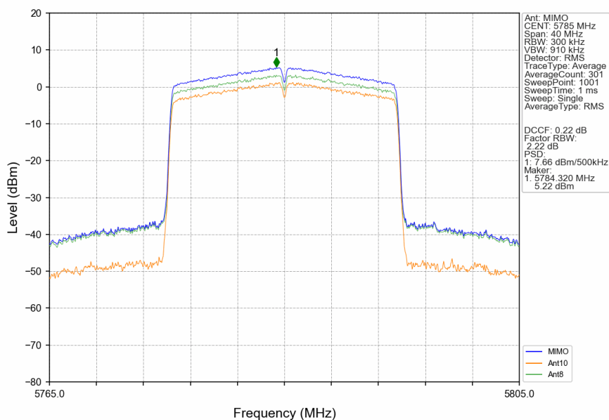
802.11be(EHT20) MCH 5785MHz 26+52 / Ant10 NTN
