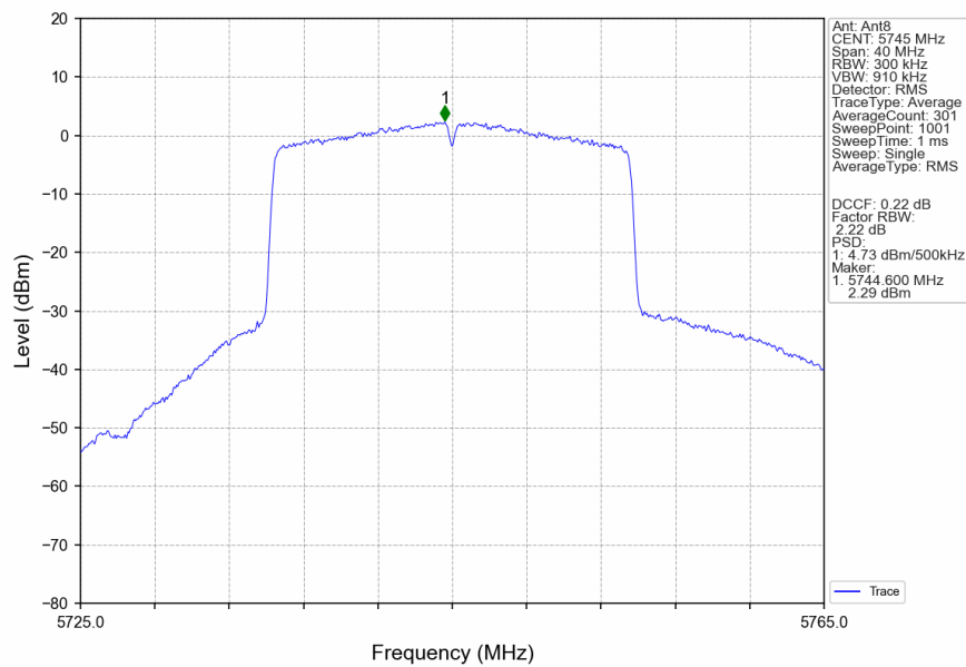
802.11be(EHT20) LCH 5745MHz RU242 Left Ant8 NTN
