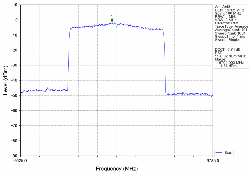
802.11ax(HEW80)_MCH_6705MHz_RU996_Left_Ant8_NTNV
