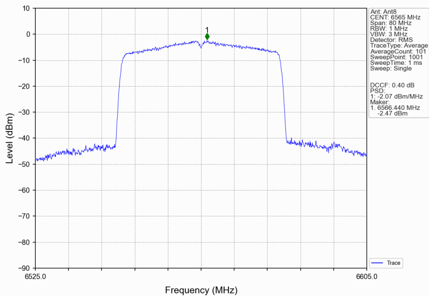
802.11ax(HEW40)_LCH_6565MHz_RU484_Left_Ant8_NTNV
