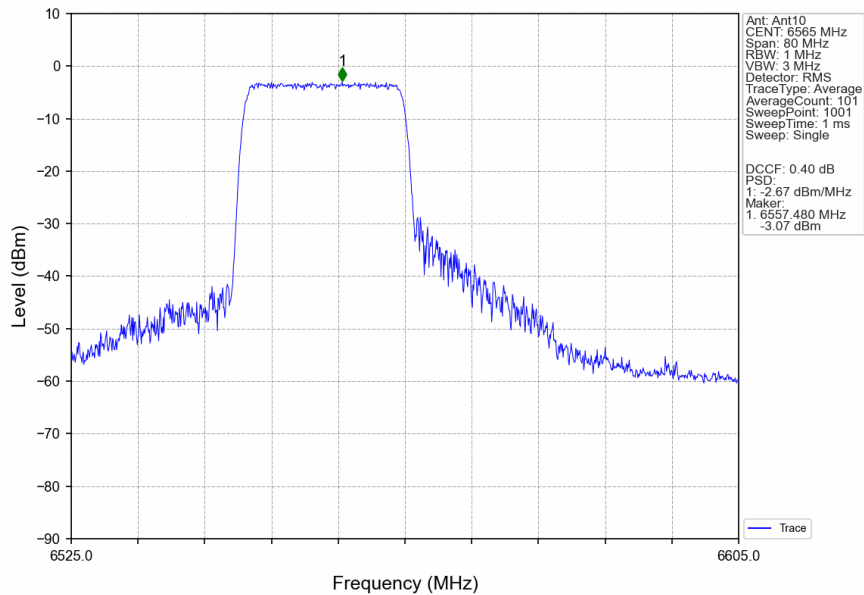
802.11ax(HEW40)_LCH_6565MHz_RU242_Left_Ant10_NTNV
