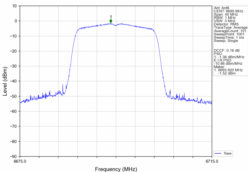
802.11a_MCH_6695MHz_MIMO_NTNV
