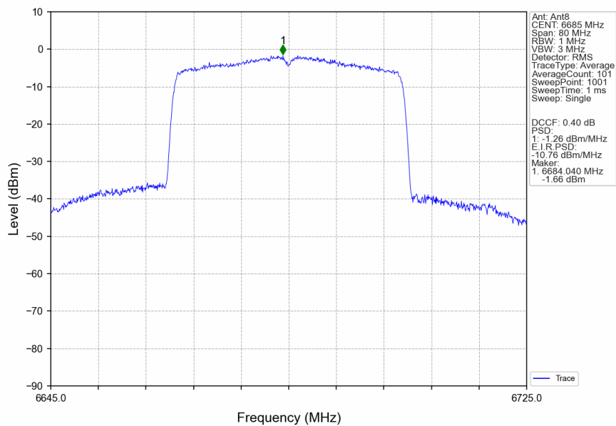
802.11ax(HEW40)_MCH_6685MHz_RU484_Left_Ant8_NTNV
