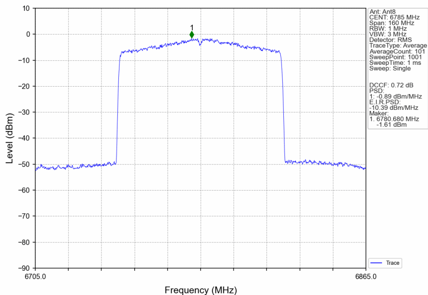
802.11ax(HEW80)_HCH_6785MHz_RU996_Left_Ant8_NTNV
