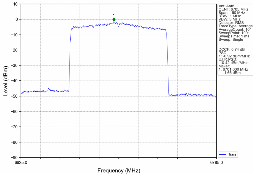
802.11ax(HEW80)_MCH_6705MHz_RU996_Left_Ant8_NTNV
