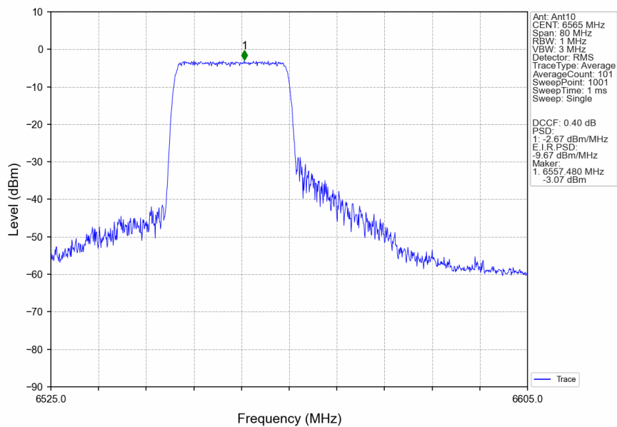
802.11ax(HEW40)_LCH_6565MHz_RU242_Left_Ant10_NTNV
