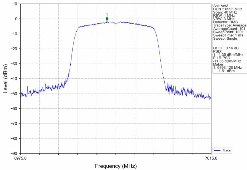
802.11a_MCH_6995MHz_MIMO_NTNV
