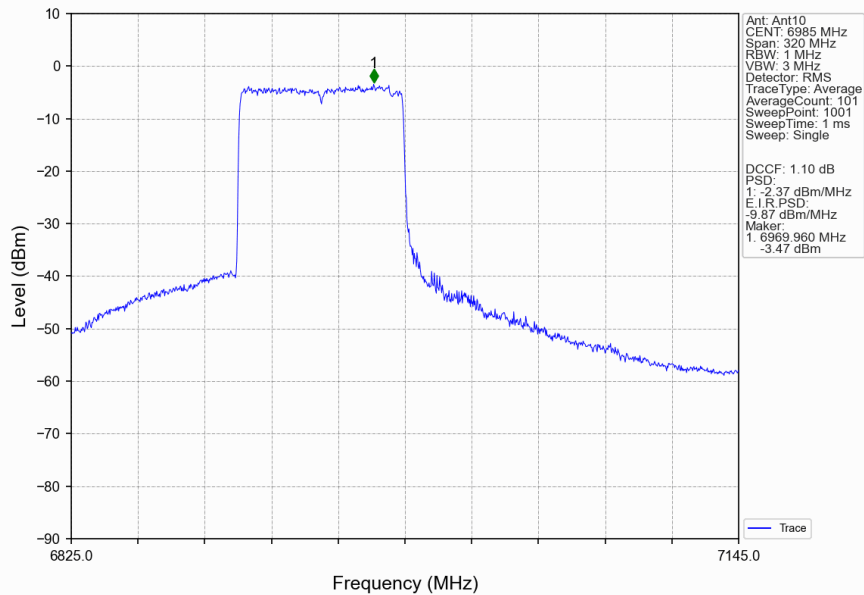
802.11ax(HEW160)_MCH_6985MHz_RU996_Left_Ant10_NTNV
