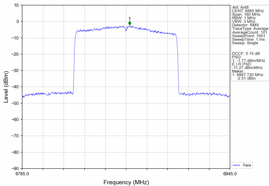
802.11ax(HEW80)_HCH_6865MHz_RU996_Left_Ant8_NTNV
