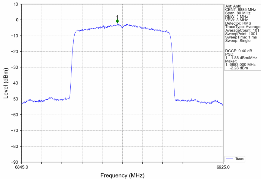
802.11ax(HEW40)_HCH_6885MHz_RU484_Left_Ant8_NTNV
