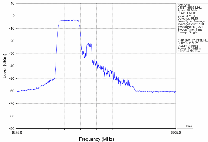
802.11be(EHT40)_LCH_6565MHz_26+106_/_Ant8_NTNV
