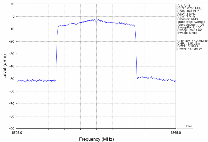
802.11be(EHT80)_HCH_6785MHz_RU996_Left_Ant8_NTNV
