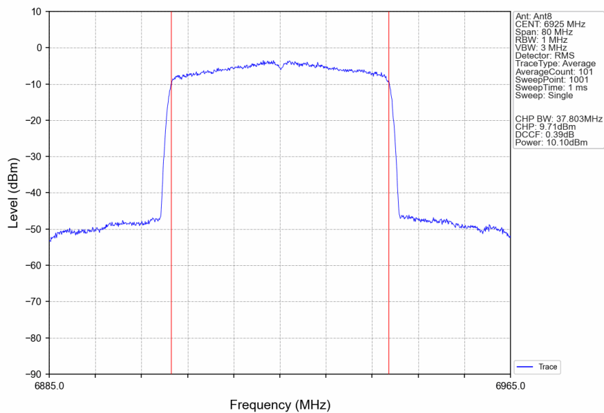
802.11be(EHT40)_LCH_6925MHz_RU484_Left_Ant8_NTNV
