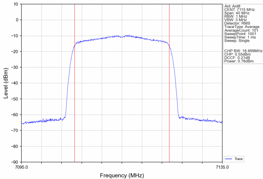
802.11be(EHT20)_HCH_7115MHz_RU242_Left_Ant8_NTNV
