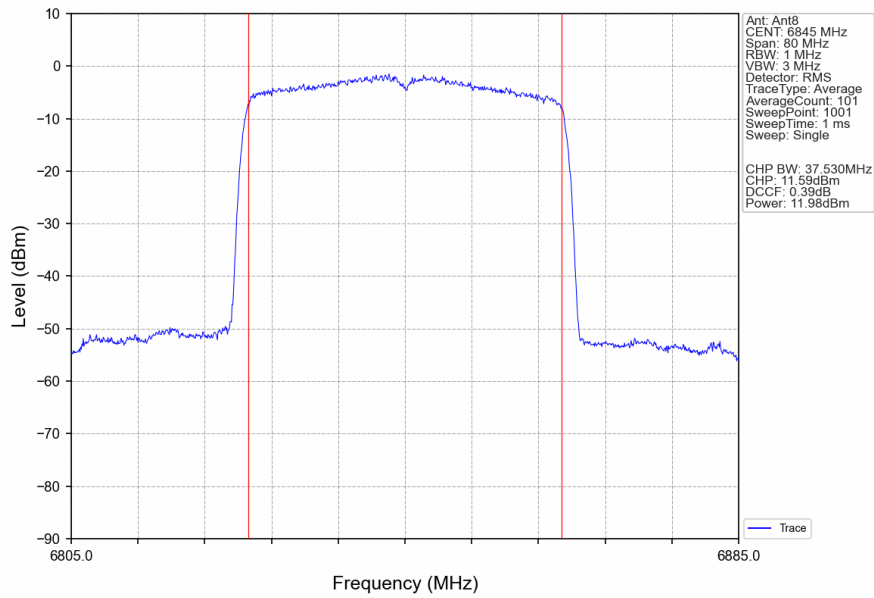
802.11be(EHT40)_HCH_6845MHz_RU484_Left_Ant8_NTNV
