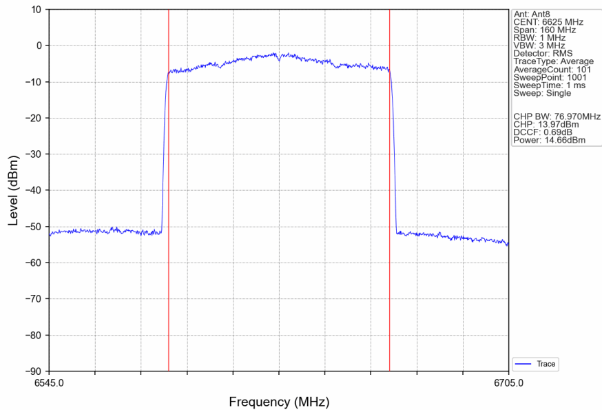
802.11be(EHT80)_LCH_6625MHz_RU996_Left_Ant8_NTNV
