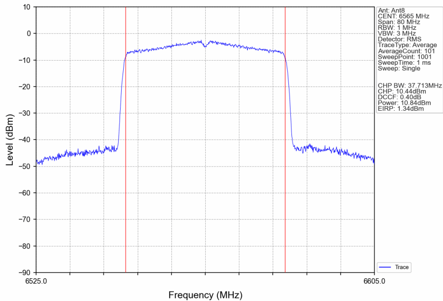
802.11be(EHT40)_LCH_6565MHz_RU484_Left_Ant8_NTNV
