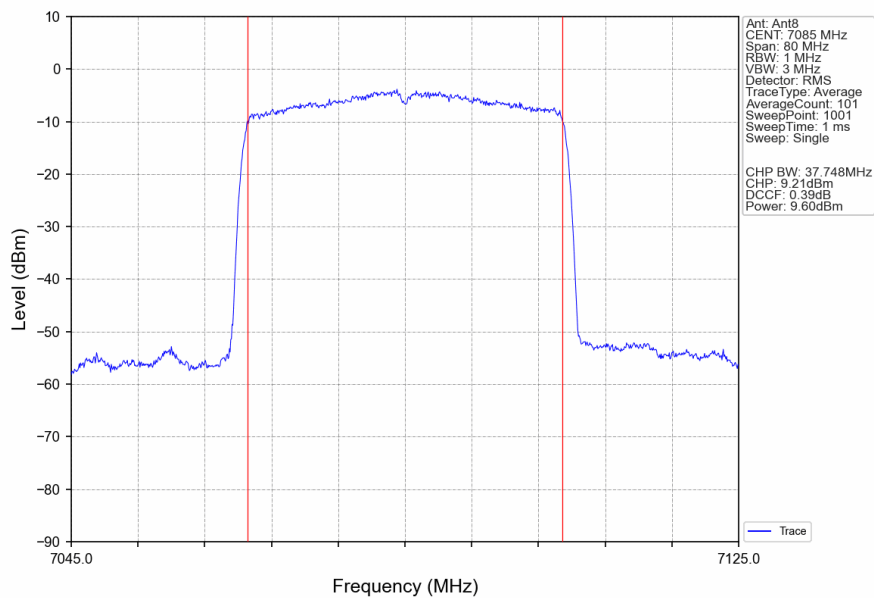
802.11be(EHT40)_HCH_7085MHz_RU484_Left_Ant8_NTNV
