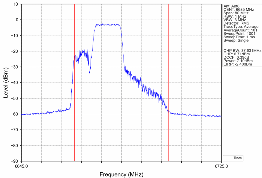
802.11be(EHT40)_MCH_6685MHz_26+106_/_Ant8_NTNV
