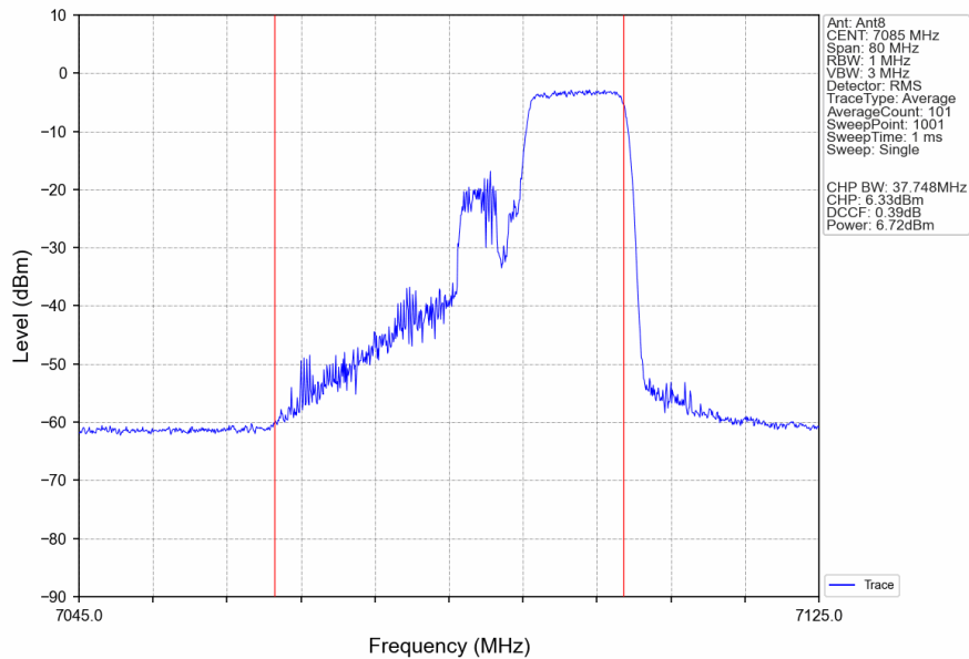
802.11be(EHT40)_HCH_7085MHz_26+106_/_Ant8_NTNV
