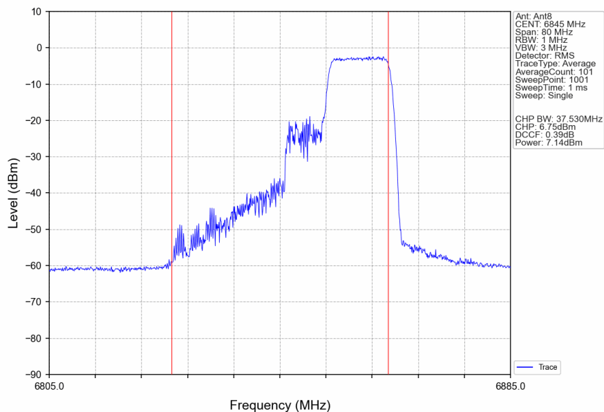
802.11be(EHT40)_HCH_6845MHz_26+106_/_Ant8_NTNV
