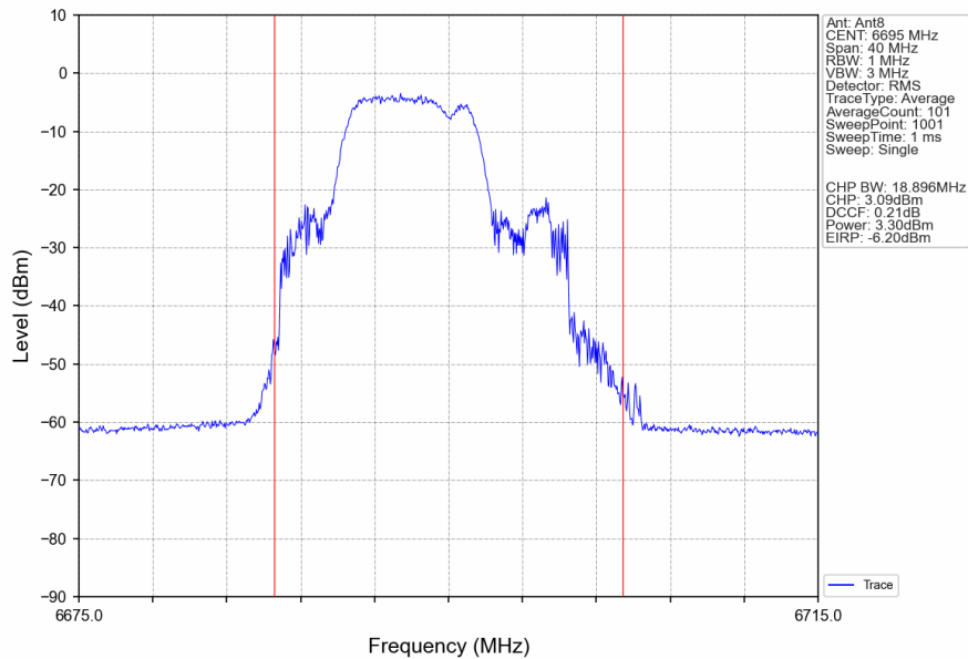
802.11be(EHT20)_MCH_6695MHz_26+52_ / Ant8_NTNV
