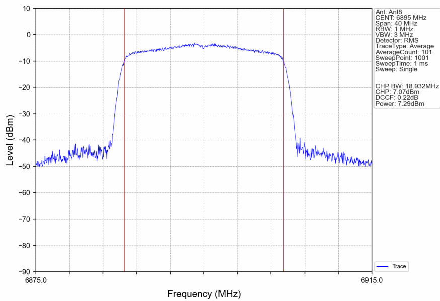
802.11be(EHT20)_LCH_6895MHz_RU242_Left_Ant8_NTNV
