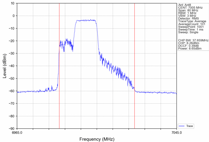
802.11be(EHT40)_MCH_7005MHz_26+106_/_Ant8_NTNV
