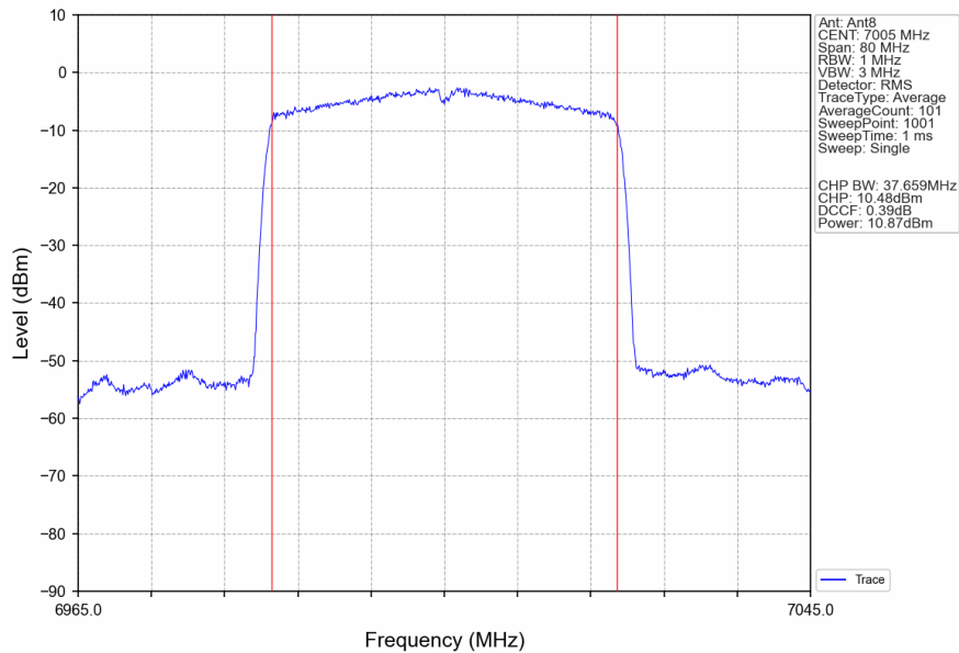
802.11be(EHT40)_MCH_7005MHz_RU484_Left_Ant8_NTNV
