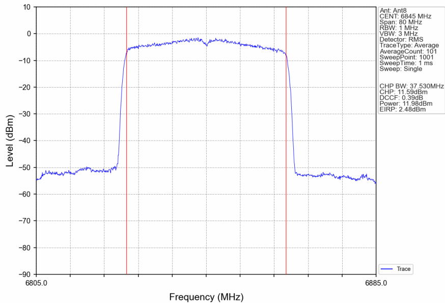
802.11be(EHT40)_HCH_6845MHz_RU484_Left_Ant8_NTNV
