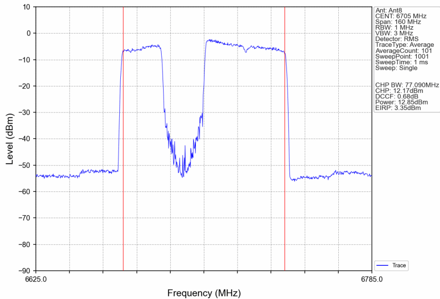
802.11be(EHT80)_MCH_6705MHz_242+484 / Ant8_NTNV
