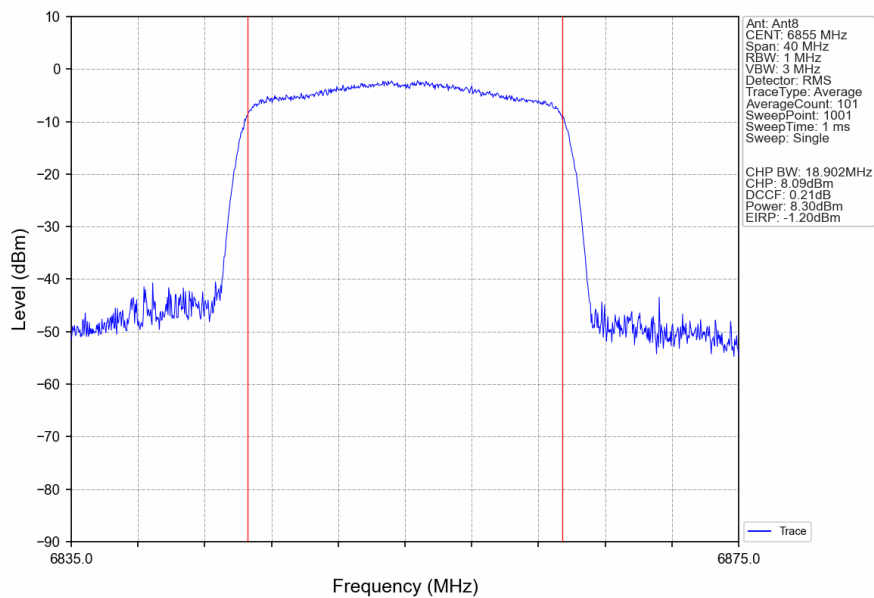
802.11be(EHT20)_HCH_6855MHz_RU242_Left_Ant8_NTNV
