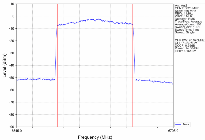
802.11be(EHT80)_LCH_6625MHz_RU996_Left_Ant8_NTNV
