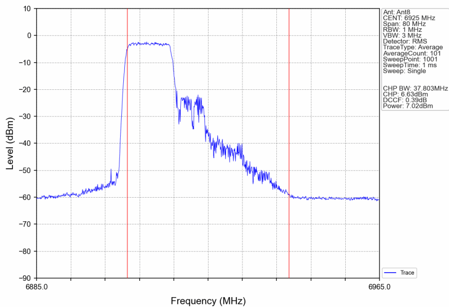
802.11be(EHT40)_LCH_6925MHz_26+106_/_Ant8_NTNV
