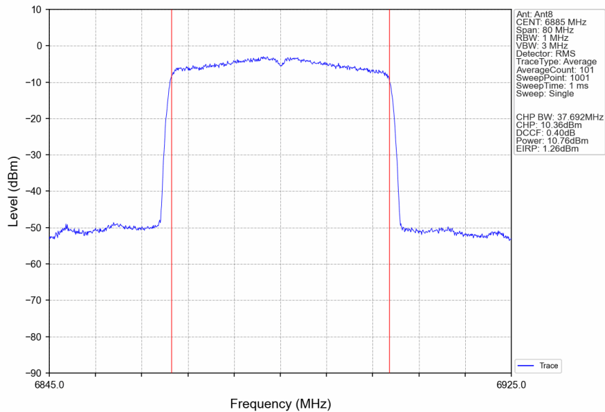
802.11be(EHT40)_HCH_6885MHz_RU484_Left_Ant8_NTNV
