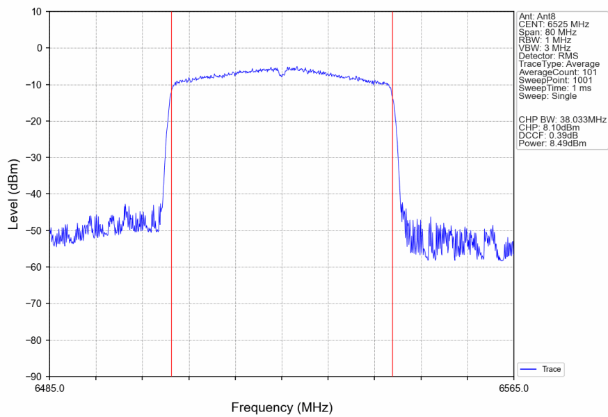
802.11be(EHT40)_HCH_6525MHz_RU484_Left_Ant8_NTNV
