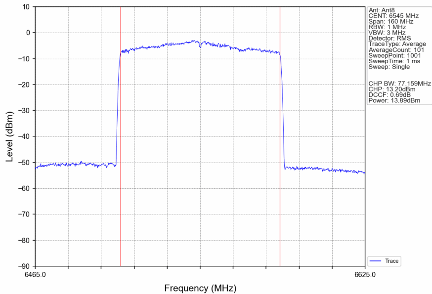
802.11be(EHT80)_HCH_6545MHz_RU996_Left_Ant8_NTNV
