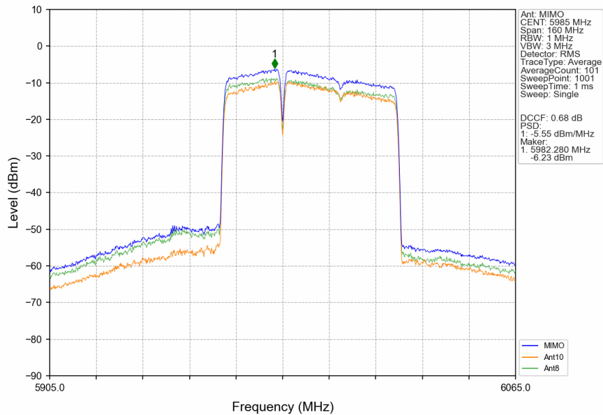
802.11be(EHT80)_LCH_5985MHz_242+484 / _MIMO_NTNV
