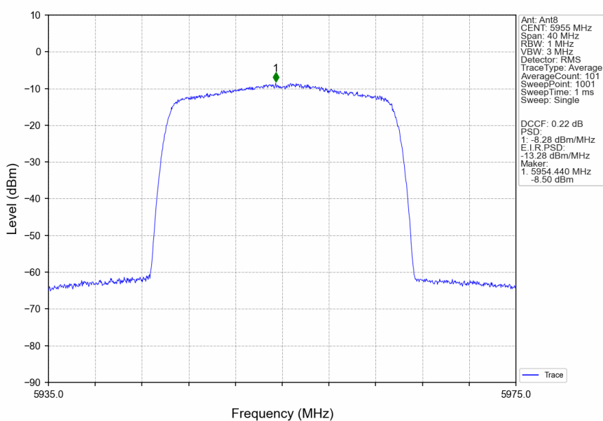
802.11be(EHT20)_LCH_5955MHz_RU242_Left_Ant8_NTNV
