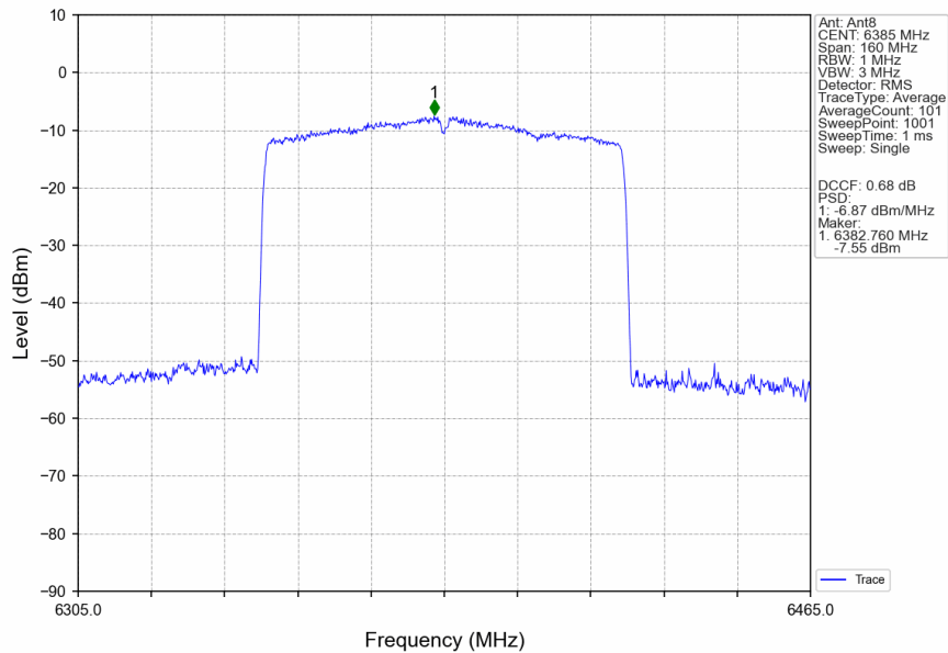
802.11be(EHT80)_HCH_6385MHz_RU996_Left_Ant8_NTNV
