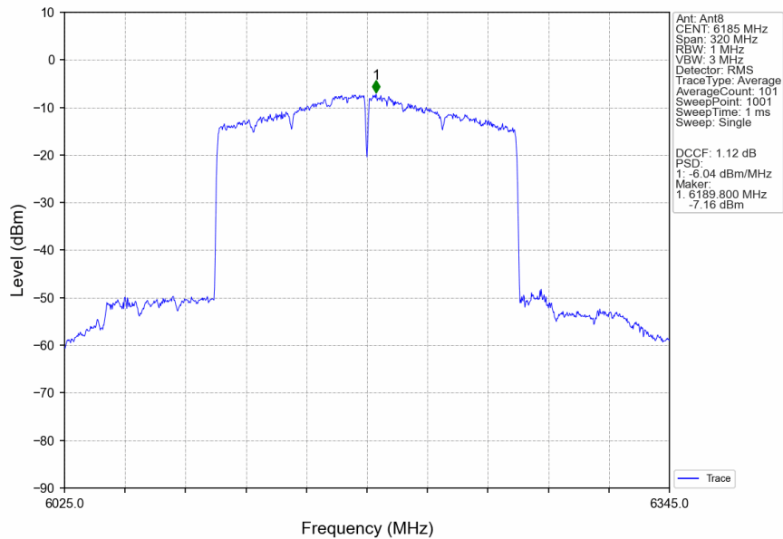
802.11be(EHT160)_MCH_6185MHz_2xRU996_Left_Ant8_NTNV
