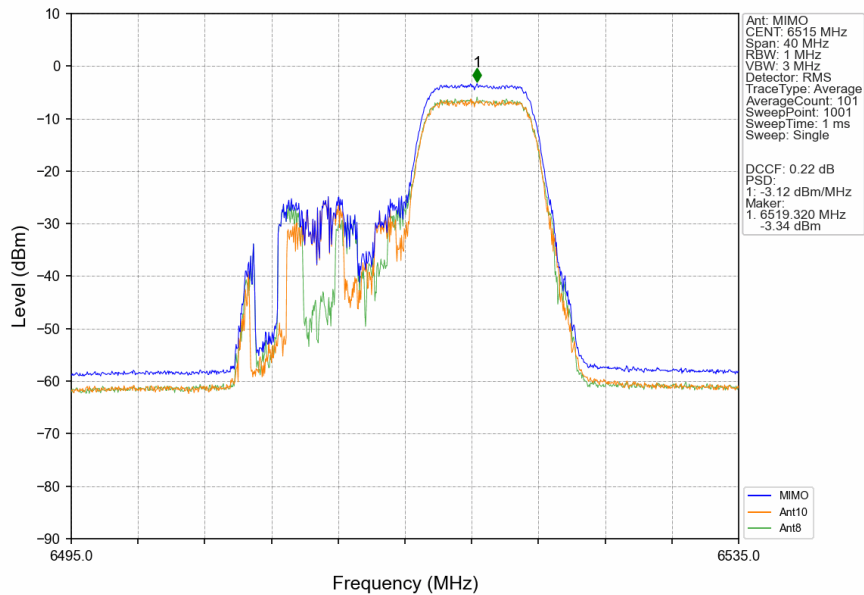
802.11be(EHT20) HCH_6515MHz_26+52 / MIMO_NTNV
