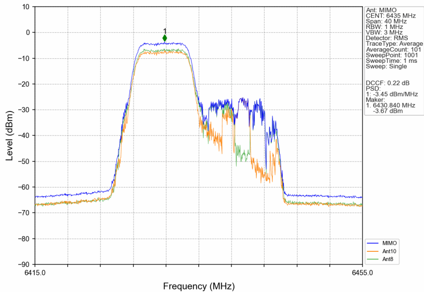
802.11be(EHT20)_LCH_6435MHz_26+52_/_MIMO_NTNV
