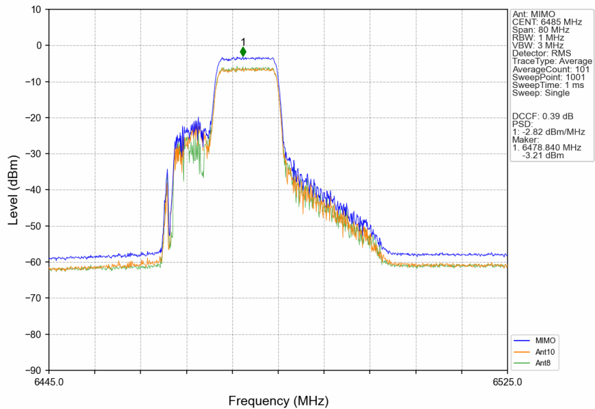
802.11be(EHT40)_MCH_6485MHz_26+106 / MIMO_NTNV
