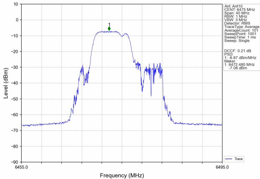
802.11be(EHT20)_MCH_6475MHz_26+52 / Ant10_NTNV
