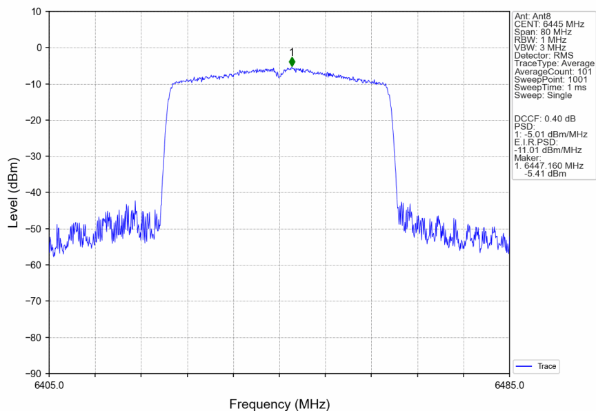
802.11be(EHT40)_LCH_6445MHz_RU484_Left_Ant8_NTNV
