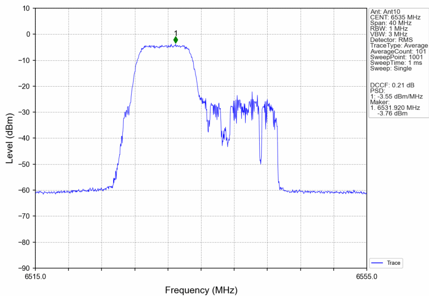
802.11be(EHT20)_LCH_6535MHz_26+52 / Ant10_NTNV
