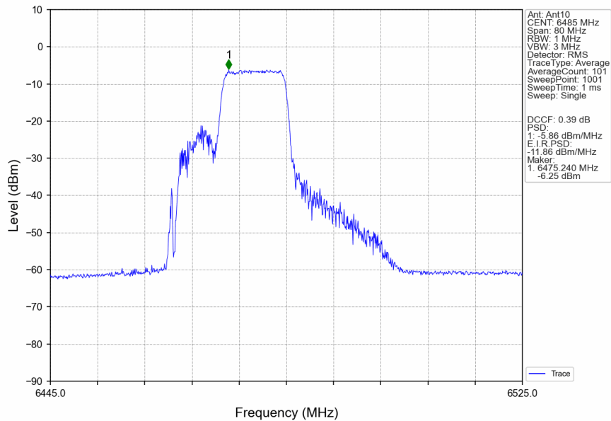
802.11be(EHT40)_MCH_6485MHz_26+106 / Ant10_NTNV
