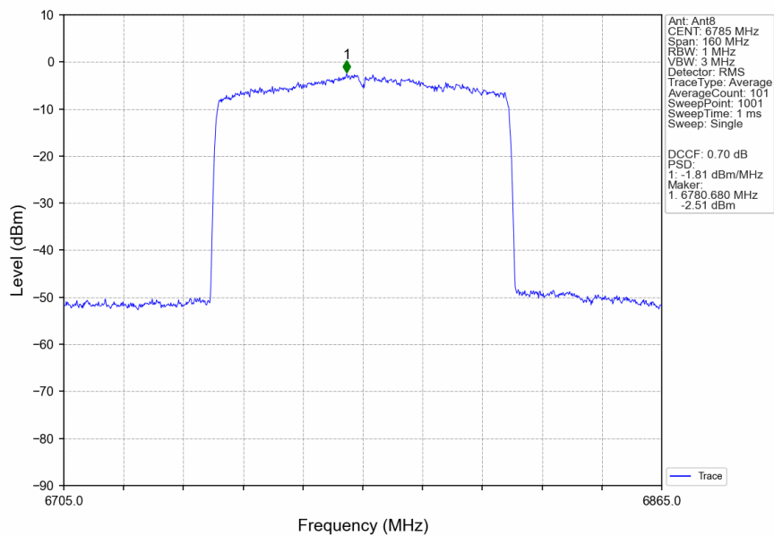
802.11be(EHT80)_HCH_6785MHz_RU996_Left_Ant8_NTNV
