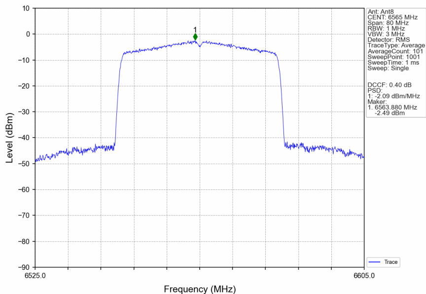
802.11be(EHT40)_LCH_6565MHz_RU484_Left_Ant8_NTNV
