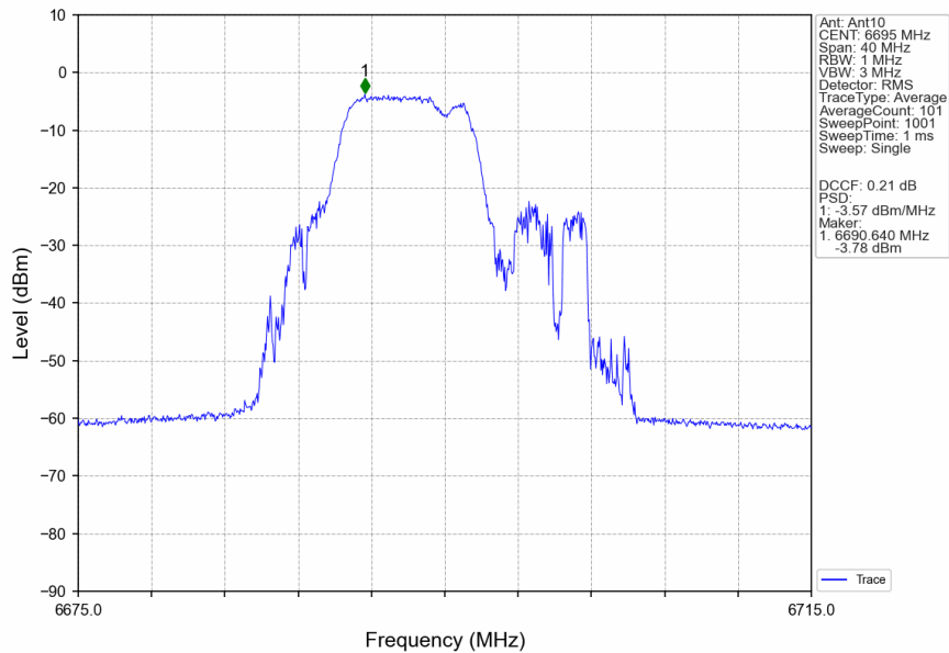
802.11be(EHT20)_MCH_6695MHz_26+52_/_Ant10_NTNV
