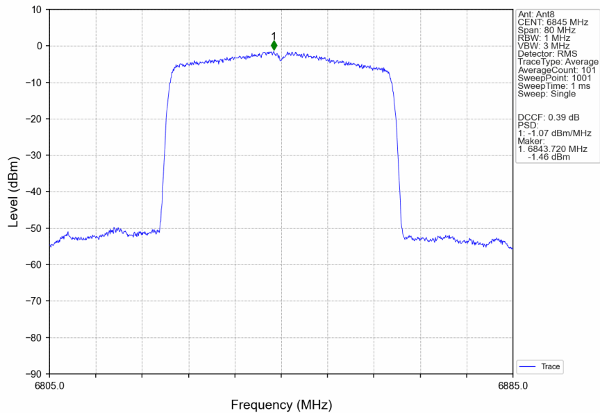
802.11be(EHT40)_HCH_6845MHz_RU484_Left_Ant8_NTNV
