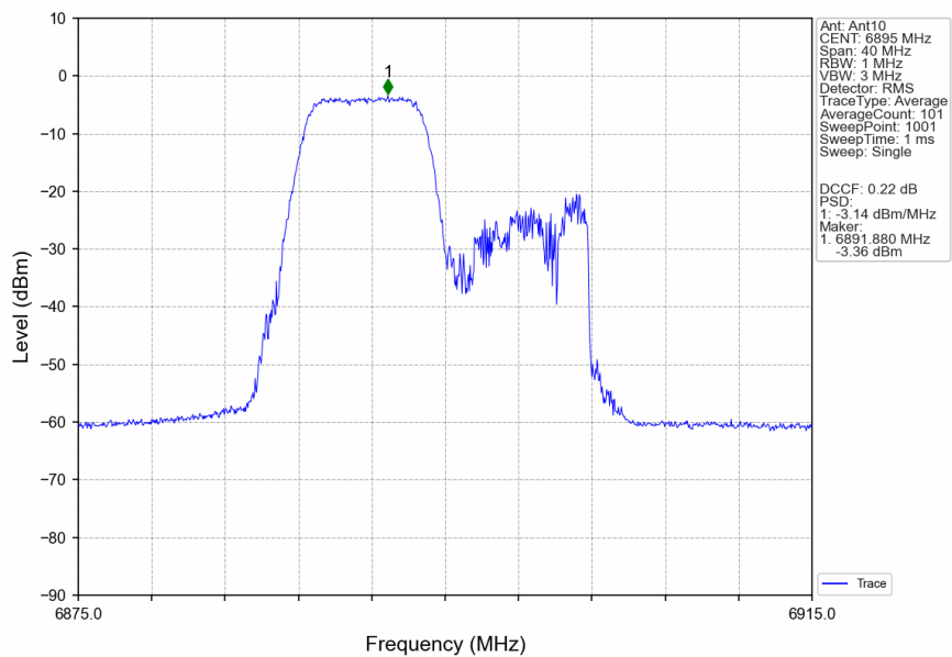
802.11be(EHT20)_LCH_6895MHz_26+52 / Ant10_NTNV
