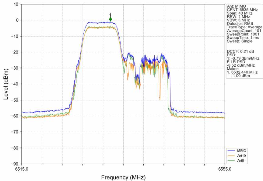
802.11be(EHT20)_LCH_6535MHz_26+52_/_MIMO_NTNV
