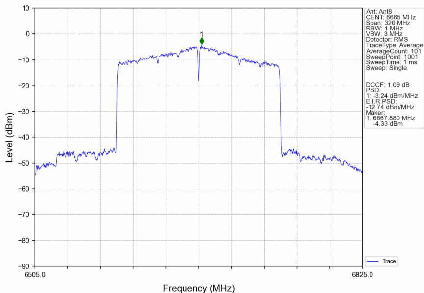
802.11be(EHT160)_MCH_6665MHz_2xRU996_Left_Ant8_NTNV
