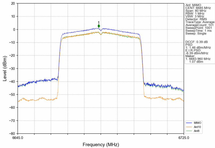
802.11be(EHT40)_MCH_6685MHz_26+106 / Ant10_NTNV
