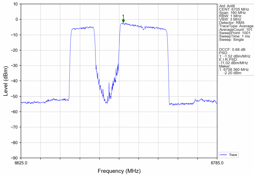
802.11be(EHT80)_MCH_6705MHz_242+484 / MIMO_NTNV
