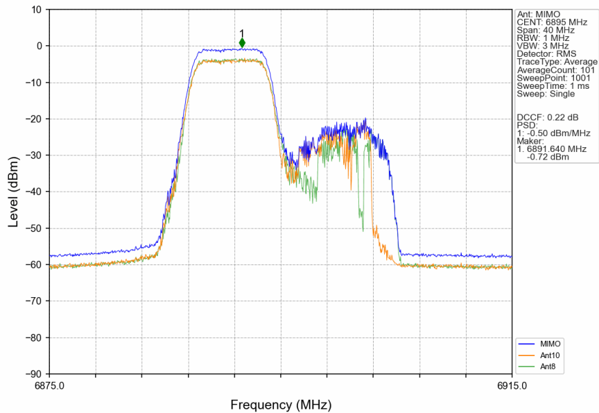
802.11be(EHT20)_LCH_6895MHz_26+52_/_MIMO_NTNV
