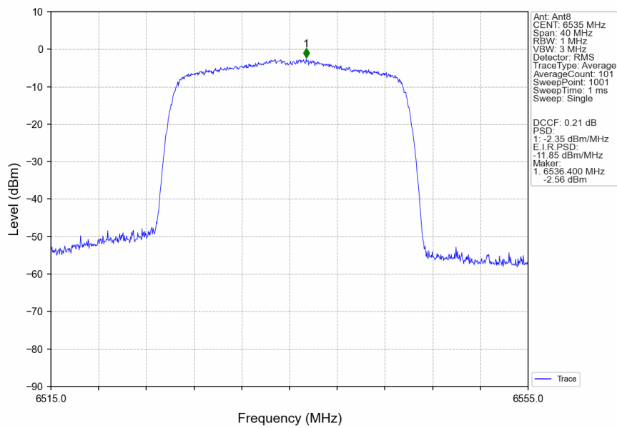
802.11be(EHT20)_LCH_6535MHz_RU242_Left_Ant8_NTNV
