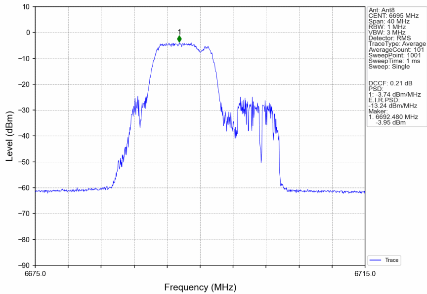
802.11be(EHT20)_MCH_6695MHz_26+52_/_MIMO_NTNV
